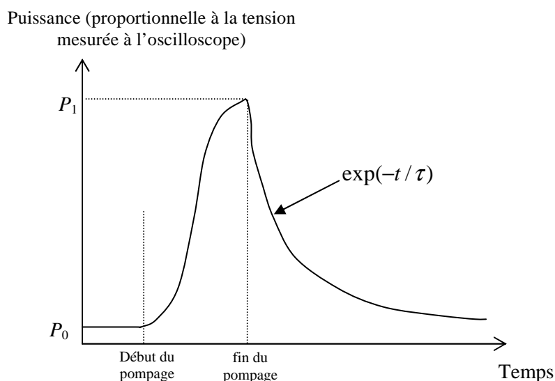
Figure 3.7 : courbe de gain typique mesurée à l'oscilloscope
