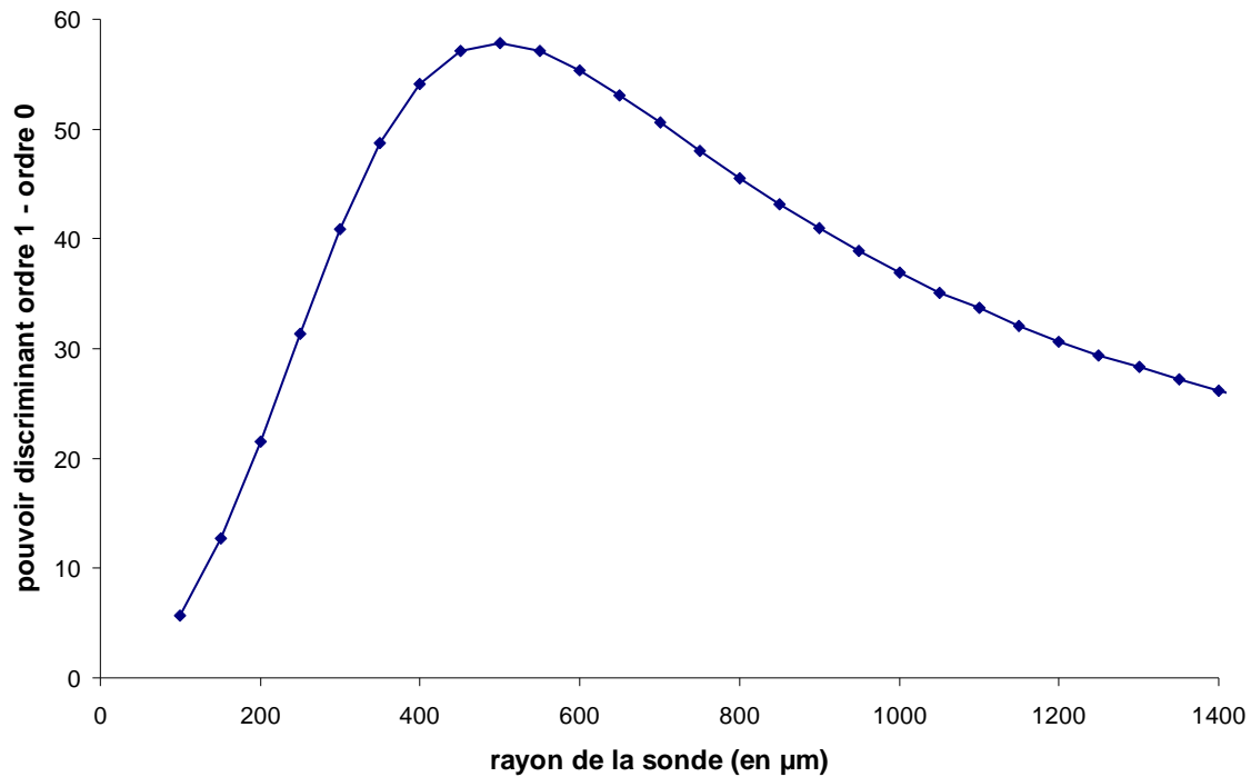
Figure 1.13 : Calcul du pouvoir discriminant des ordres +/-1 par rapport à l'ordre 0 calculés à z=1\text{m} en fonction du rayon de la sonde
