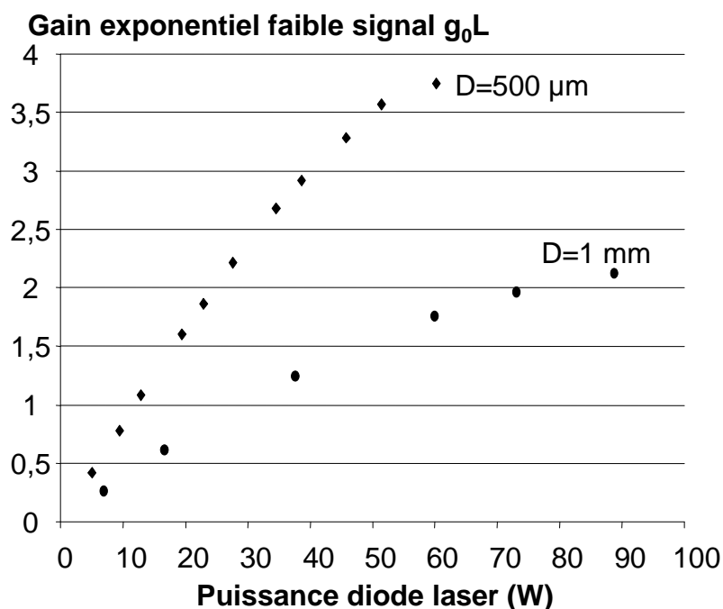
Figure 2.19 : Gain faible signal des fibres cristallines Nd:YAG pompées en régime continu, pour 2 diamètres de fibre (longueur = 5 cm)
