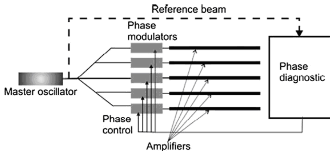
Figure 0.1 : Dispositif permettant de mettre en phase N sources lasers via une boucle de réaction électronique [Desfarges-Berthelemot 2006]
