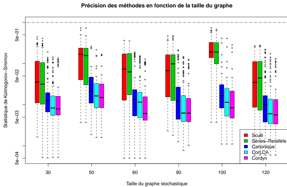
FIGURE 1.6.4 – Précision de cinq méthodes en fonction du nombre de variables aléatoires dans le graphe stochastique (de 30 à 120)
