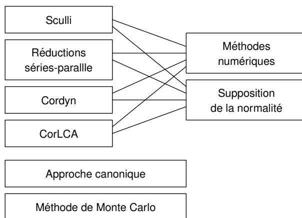
FIGURE 1.6.1 – Méthodes implémentées dans Emapse. Les différentes approches pour traiter la dépendance entre les résultats intermédiaires sont positionnées à gauche. Les méthodes pour évaluer les opérations arithmétiques sont à droite.
