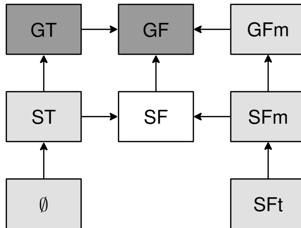
FIGURE 4.7.1 – Bilan de la complexité des problèmes d'évaluation (gris clair pour les problèmes polynomiaux, blanc pour le problème ouvert, gris foncé pour les problèmes \#P' -Complets). Les lettres caractérisent les différentes problématiques : G pour les ordonnancements généraux ; S pour les ordonnancements stricts ; T pour les pannes transitoires ; F pour les pannes franches ; m pour les ordonnancements monotones ; t pour les ordonnancements triangulaires ; \emptyset pour les ordonnancements sans réplication.
