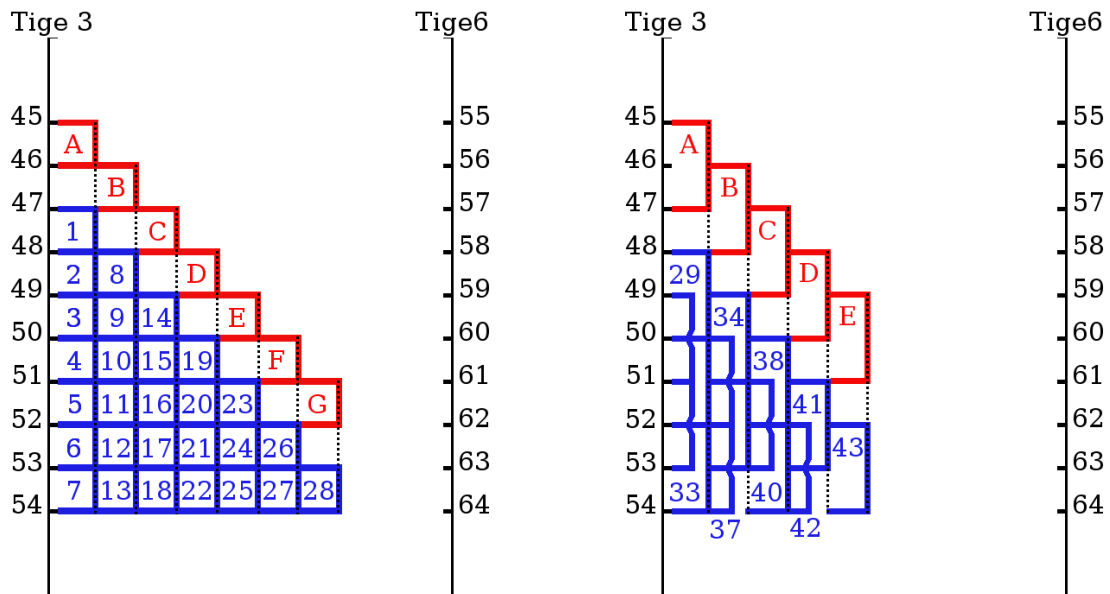
FIGURE 8 – À gauche, Étape 35 de la mesure automatisée de résistivité électrique dans la cuve. Dipôles de distance inter-électrodes 5 cm. À droite, Étape 36 . Dipôles de distance inter-électrodes 10 cm. L'injection de courant apparaît en rouge, la mesure de potentiel en bleu.
