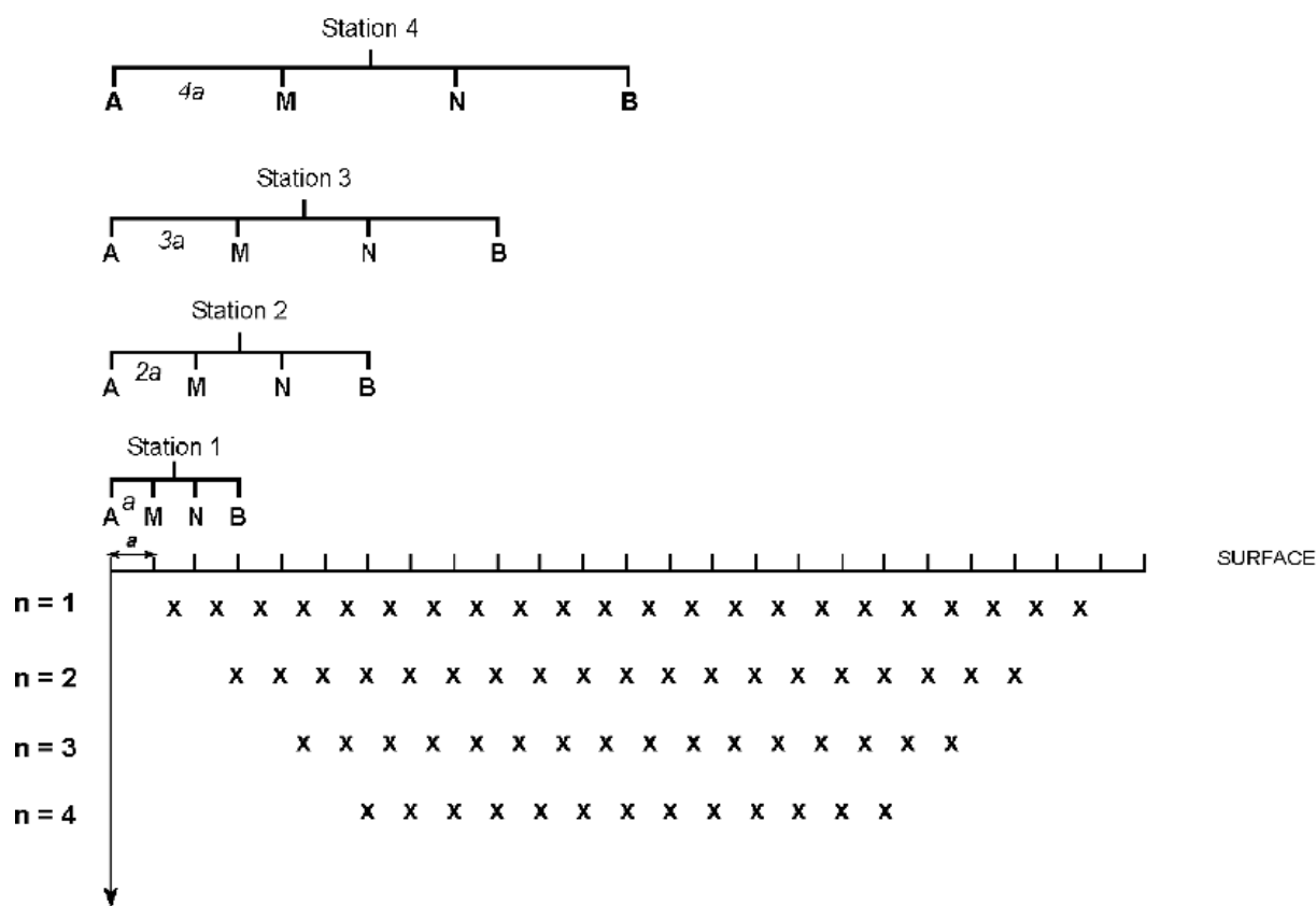
FIGURE 5.3 – Acquisition d'une pseudo-section de résistivité électrique 2D en géométrie d'acquisition de type Wenner. (Samouëlian et al., 2005)
