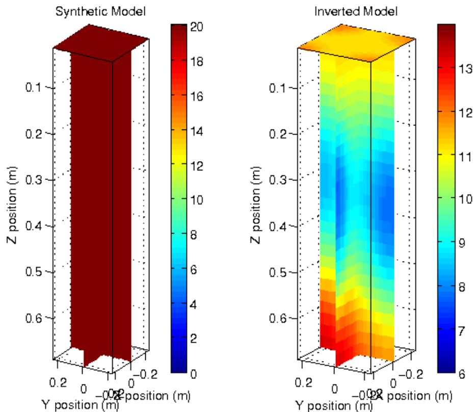
FIGURE 5.18 – Résistivité électrique dans la cuve inversée grâce à RESINVM3D (à droite) à partir d'un modèle initial uniforme (à gauche). Les échelles de couleur représentent la résistivité électrique, en \Omega.m .
