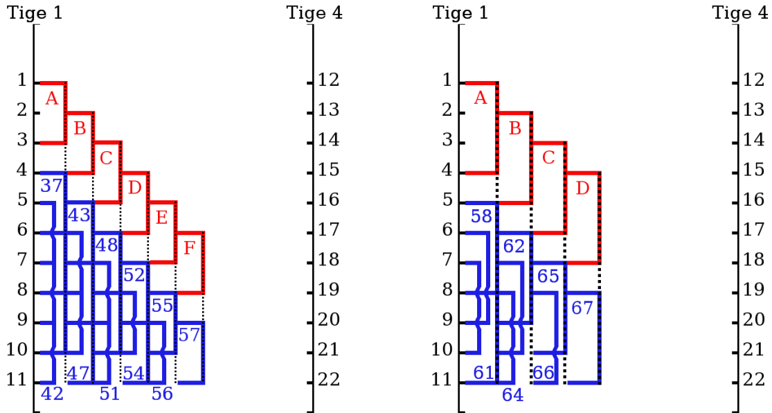
FIGURE 2 – À gauche, Étape 2 de la mesure automatisée de résistivité électrique dans la cuve. Dipôles de distance inter-électrodes 10 cm. À droite, Étape 3 . Dipôles de distance inter-électrodes 15 cm. L'injection de courant apparaît en rouge, la mesure de potentiel en bleu.
