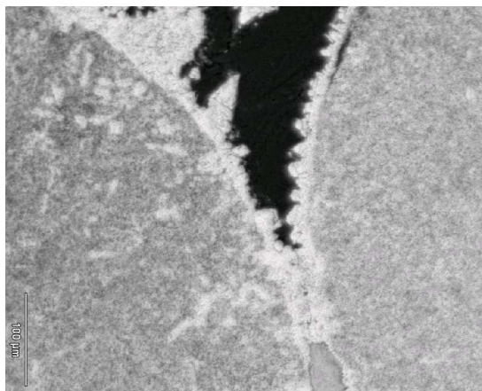
FIGURE 4.34 – Porosité intergranulaire. Détail : cristal de sparite de 50\mu\text{m} .
