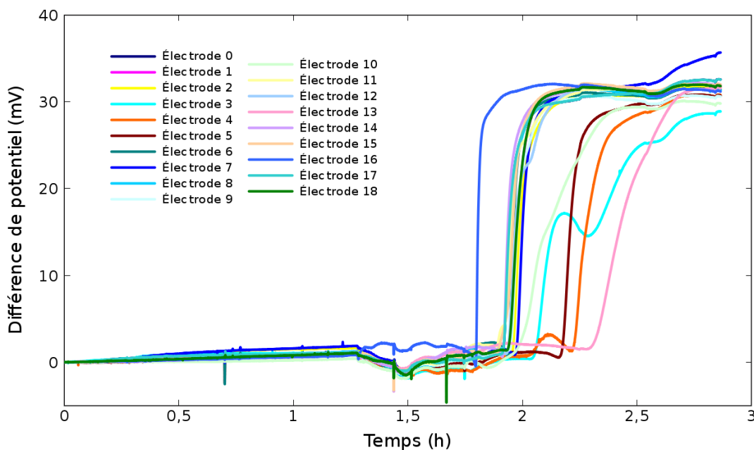
FIGURE 5.14 – Différence de potentiel entre les électrodes de PS de surface et l'électrode de référence enfoncée à mi-profondeur de la cuve en fonction du temps.
