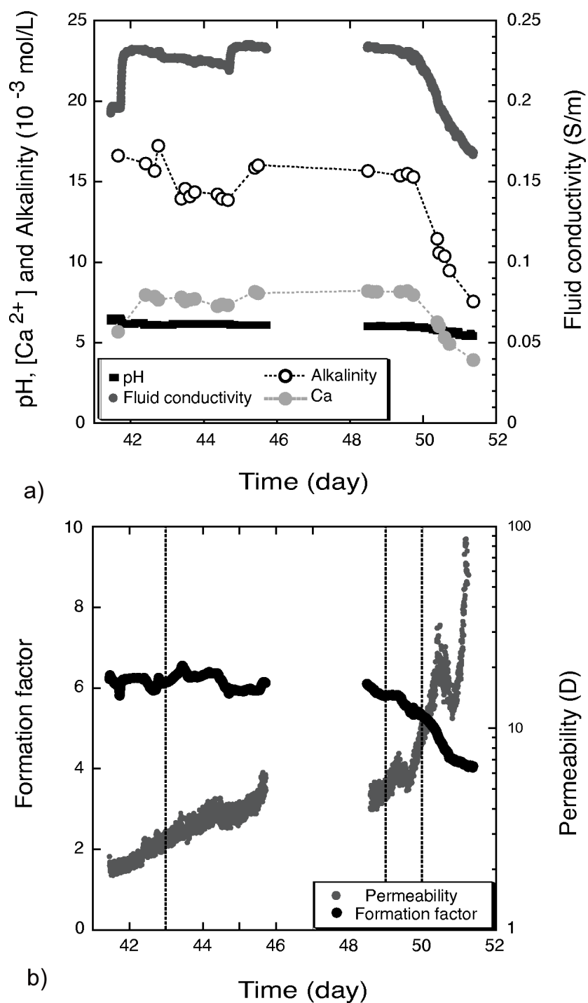
FIGURE 4.6 – a) Évolution de l'alkalinité, de la concentration en ions calcium, du pH et de la conductivité électrique de la solution à la sortie de l'échantillon au cours du temps pendant l'injection d'eau saturée en CO 2 (SC3) dans l'échantillon de calcaire de St-Maximin (M1). Le jour 42 correspond au début de l'injection de CO 2 . b) Évolution de la perméabilité et du facteur de formation électrique pendant l'injection (SC3) de CO 2 dans l'échantillon M1.
