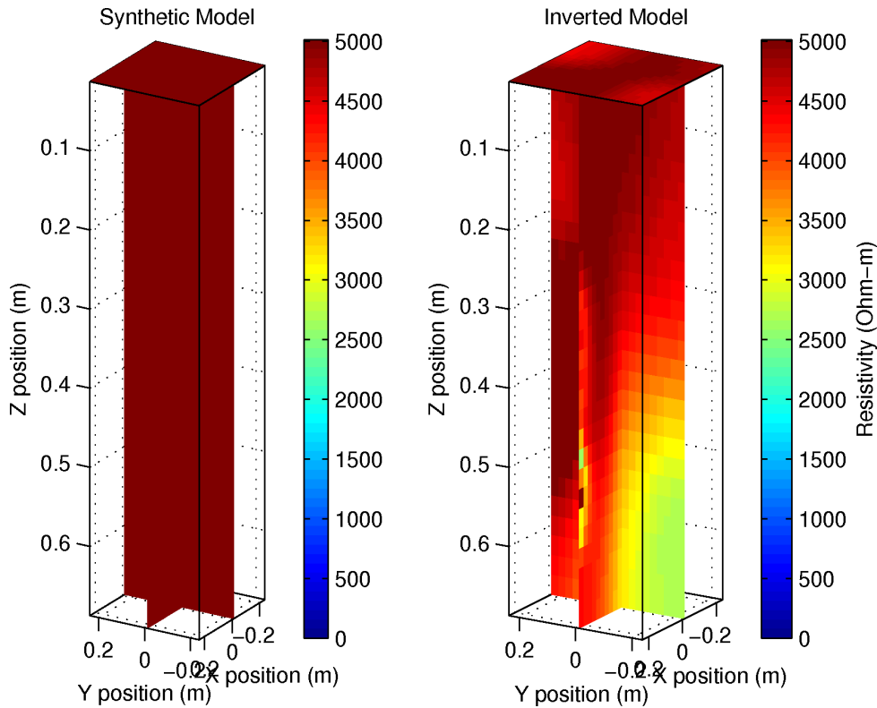
FIGURE 5.23 – Résistivité électrique dans la cuve inversée grâce à RESINVM3D (à droite) à partir d'un modèle initial uniforme (à gauche) de 5 k\Omega.m . Après 7 itérations.
