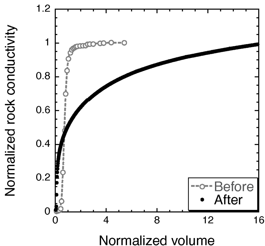
FIGURE 4.18 – Évolution de la conductivité électrique de l'échantillon de calcaire S7 initialement saturé d'eau distillée, avant (en blanc) et après (en noir) expérience, lors de l'injection de 16 volumes poreux d'eau fortement salée ( 25 \text{ g.l}^{-1} ). Cette conductivité de la roche est normalisée à la valeur maximale atteinte en fin d'expérience.
