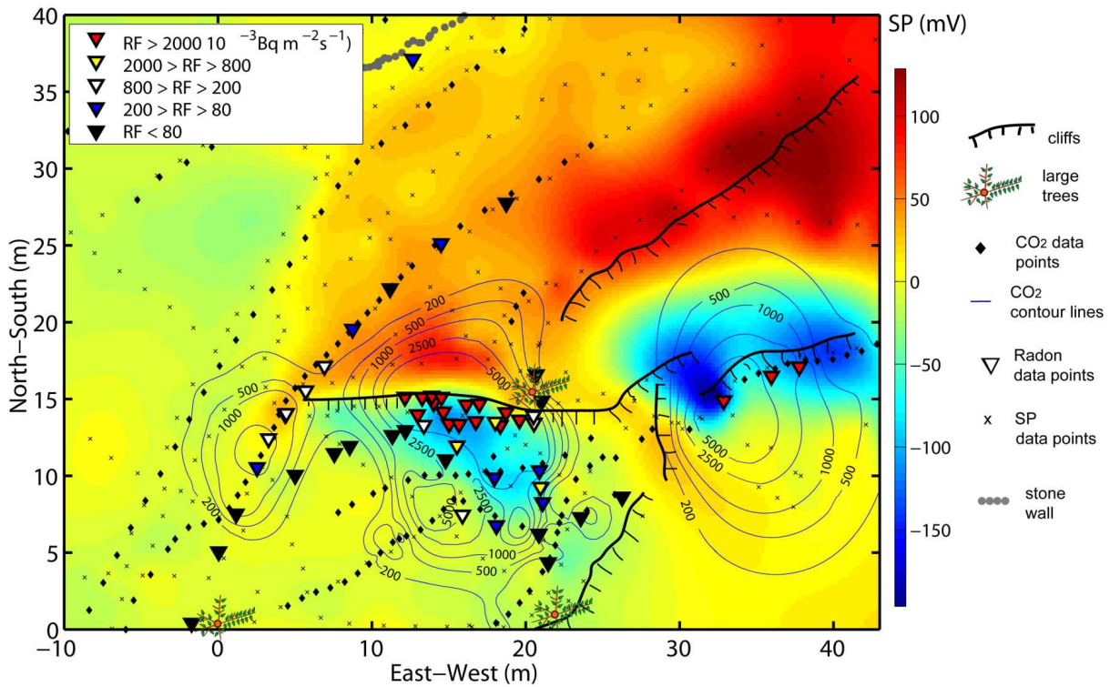
FIGURE 6.9 – Potentiel Spontané dans le voisinage des sources chaudes de Syabru Bensi. Flux local de radon-222 et niveau de flux de CO_2 au sol.
