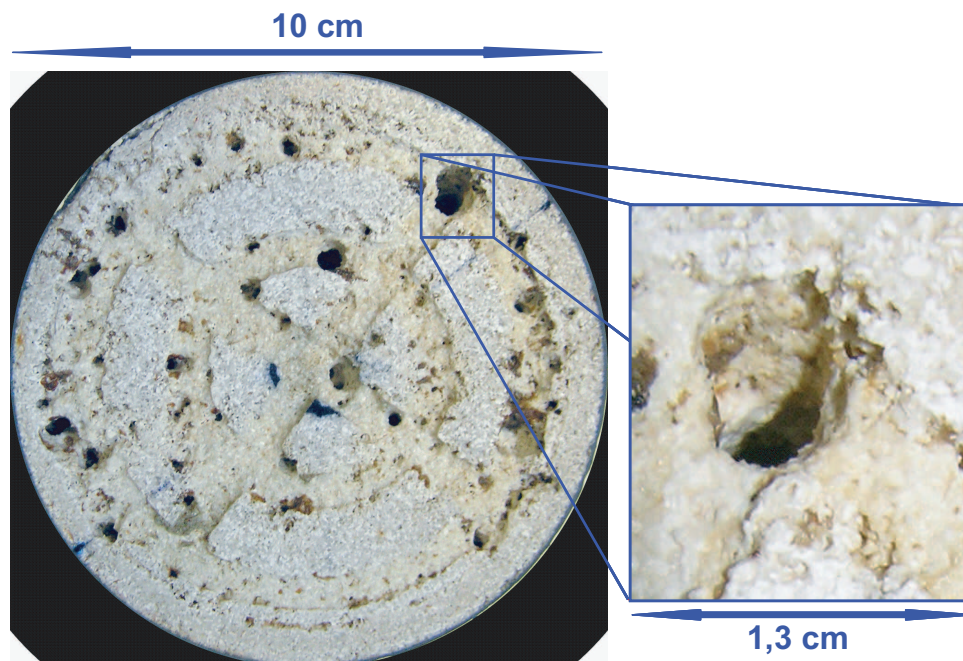
FIGURE 4.19 – Face d'entrée de l'échantillon de calcaire des Estailades après un mois d'injection d'eau saturée en \text{CO}_2 à un débit de 5\text{ml}\cdot\text{min}^{-1} . À droite, agrandissement sur une cavité créée.
