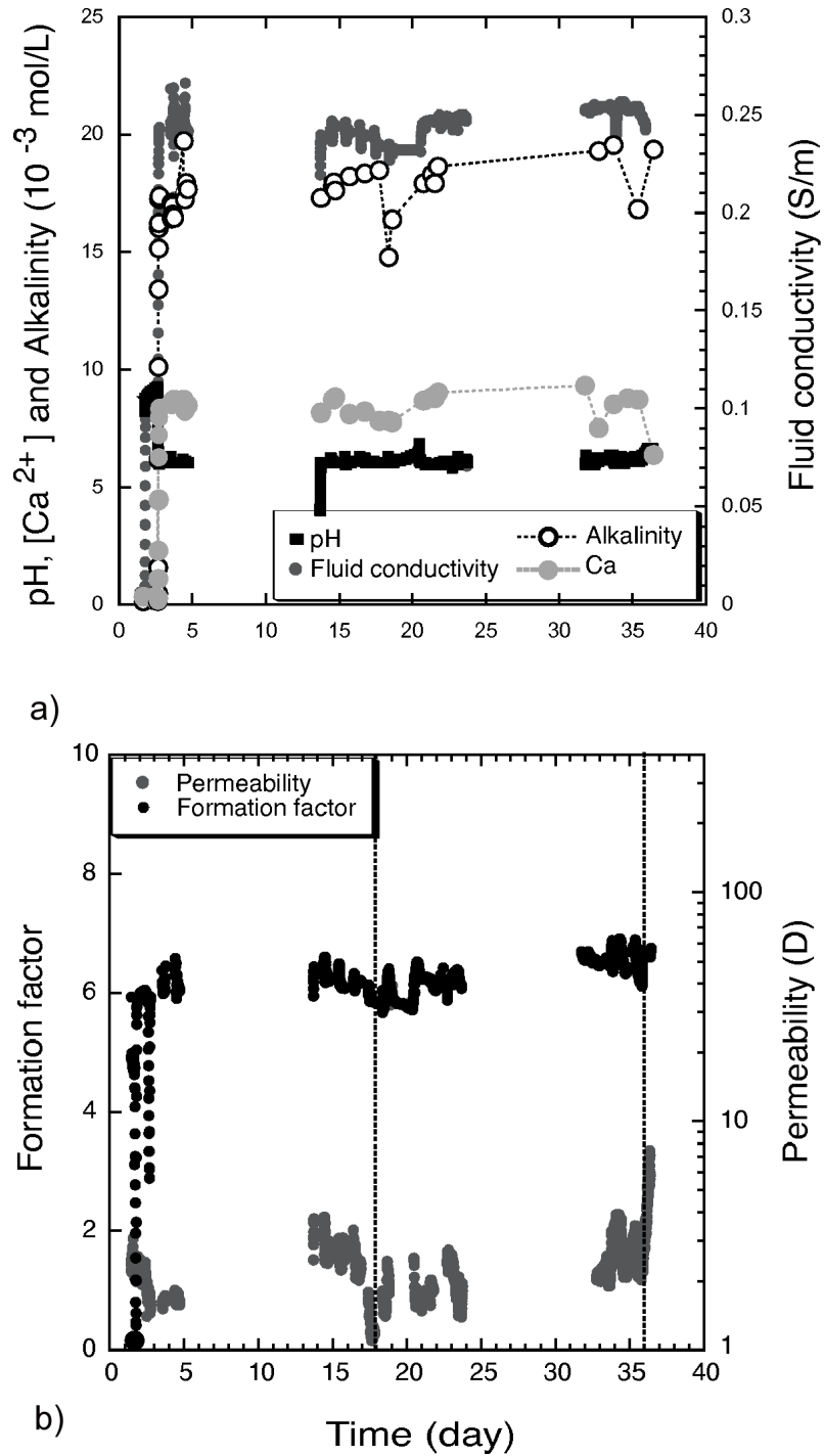
FIGURE 4.5 – a) Évolution de l'alcalinité, de la concentration en ions calcium, du pH et de la conductivité électrique de la solution à la sortie de l'échantillon au cours du temps pendant l'injection d'eau saturée en CO_2 (SC2) dans l'échantillon de calcaire de St-Maximin (M1). b) Évolution de la perméabilité et du facteur de formation électrique pendant l'injection (SC2) de CO_2 dans l'échantillon M1.
