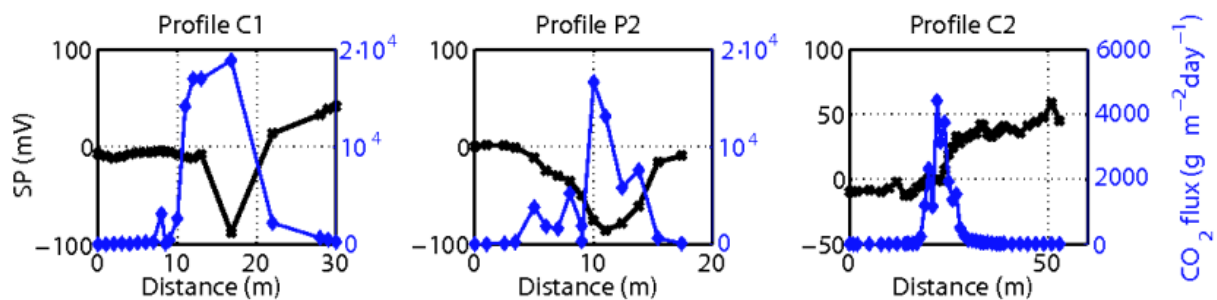
FIGURE 6.10 – Flux de CO_2 au sol (en bleu) et Potentiel Spontané (en noir) pour les profils C1, P2 et C2.
