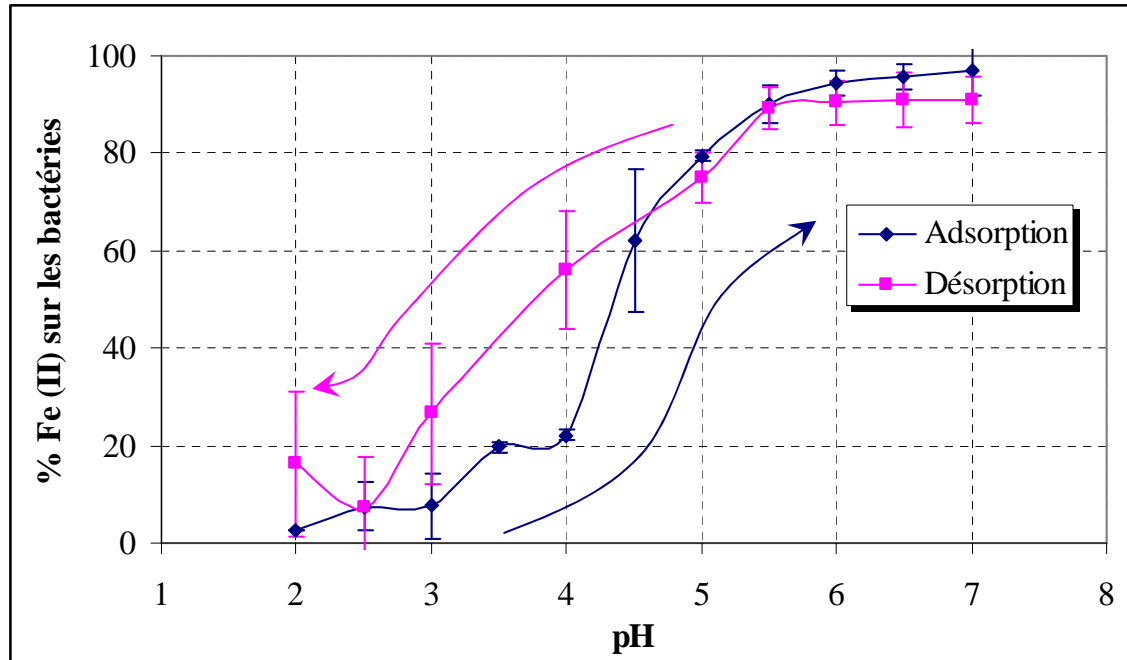
Figure II.2.1. Isothermes d'adsorption et désorption des ions Fe(II) ( 10^{-4} M) à la surface de Bacillus subtilis ( 5 \text{ g.L}^{-1} ). Les barres d'erreur correspondent à cinq répétitions de l'expérience avec cinq suspensions bactériennes différentes.
