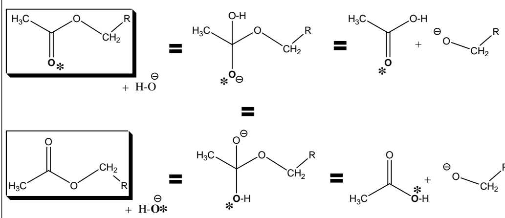
Figure 2. Mécanisme 3 avec un transfert de H + supplémentaire
