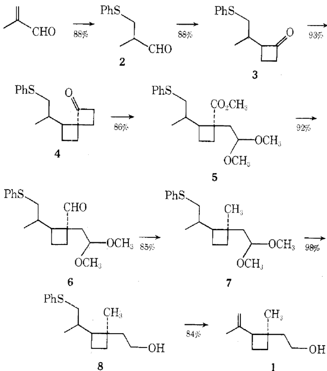
Fig. 2 : Synthèse de Gueldner et al. (extrait de l'article, p. 2013)
