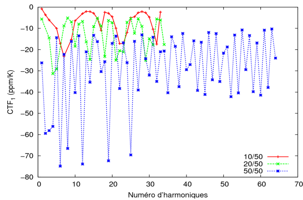
Figure 3.9: Evolution du CTF 1 des modes de l'empilement niobate (YXl)/165° sur quartz (YXl)/35° pour différents rapports d'épaisseur (10µm, 20µm et 50µm de niobate sur 50µm de quartz)
