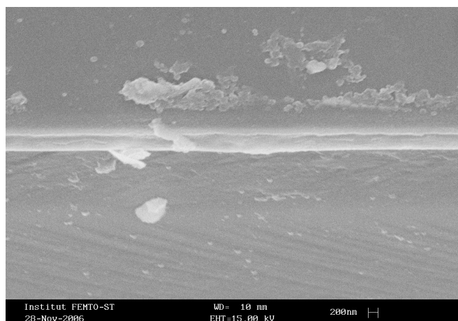
Figure 2.11: Image MEB (microscopie électronique à balayage) de l'interface LiNbO3/Si. On note la couche mince (200nm) d'or uniforme
