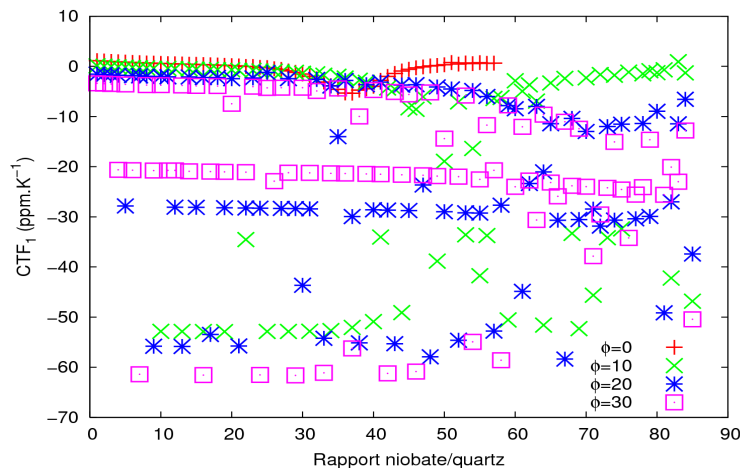
Figure 3.19: Evolution du CTF1 des modes de l'empilement niobate (YXl)/165° sur quartz (YXwl)/ \theta /35° avec \theta variant de 0 à 30° pour un rapport d'épaisseur 1 \mu m de niobate sur 50 \mu m de quartz
