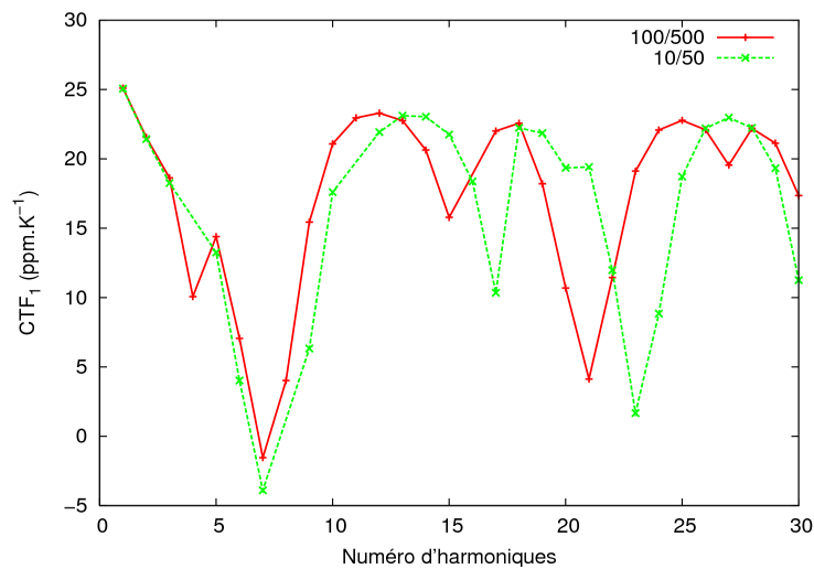
Figure 3.18: Comparaison des CTF 1 des modes de l'empilement niobate (YXl)/165° sur quartz (YXl)/30° pour les rapports d'épaisseur niobate/quartz de 100/500 et 10/50 (implicitement en \mu\text{m} )
