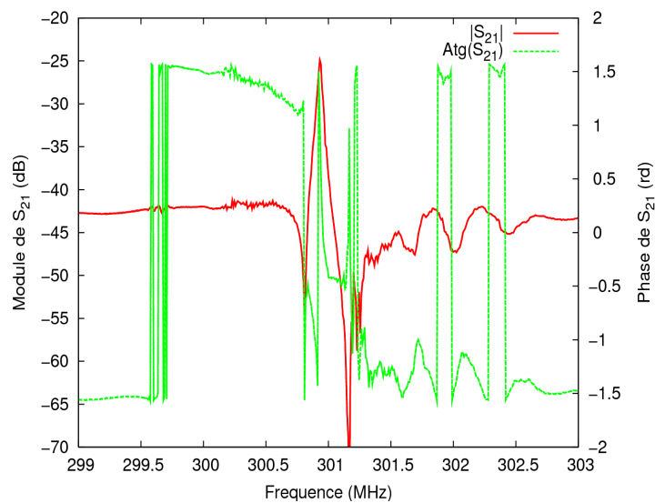
Figure 4.14: Elément de filtre en échelle au voisinage de l'harmonique 3 du mode fondamental de la couche de transduction
