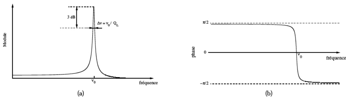
Figure 1.14.: Module (a) et phase (b) de la réponse d'un résonateur.
