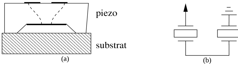
Figure 2.4: Schéma de principe des résonateurs séries
