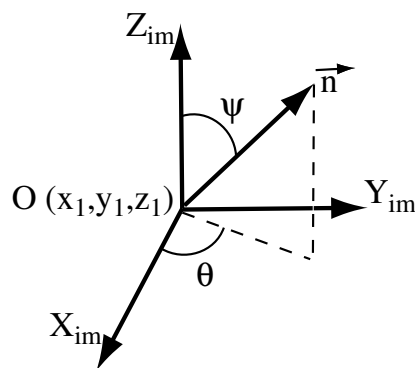
FIGURE 2.5 : Orientation de la normale du miroir par rapport au repère image.
