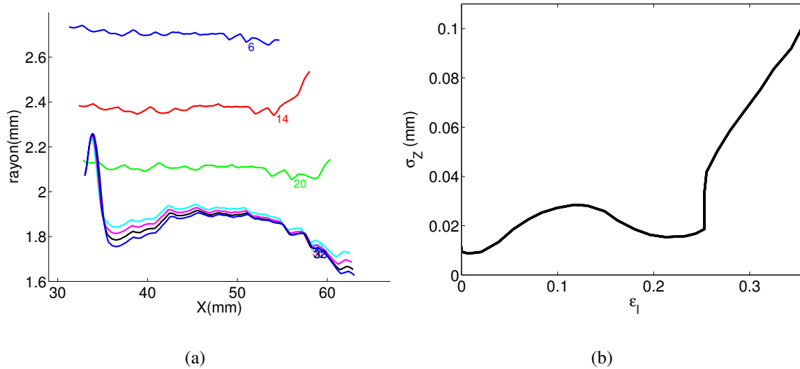
FIGURE 4.20 : Profil de la surface de l'éprouvette cylindrique sollicitée en traction rapide par la méthode spatiotemporelle. Les numéros correspondent aux différents instants.
