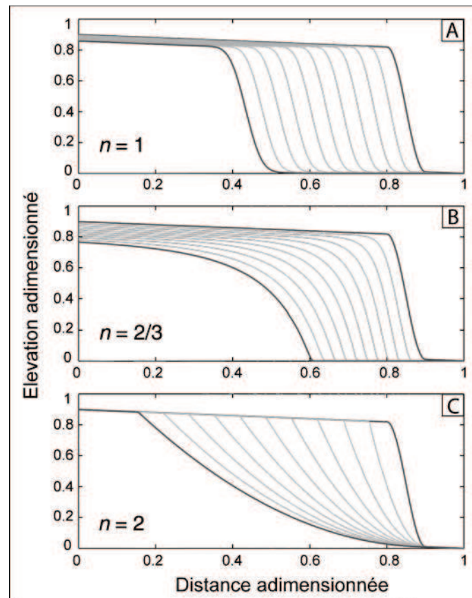
Figure 1.2.13. Exemple de simulations numériques en différences finies reproduisant la réponse d'un modèle limité par le détachement à une chute rapide du niveau de base (profil initial présentant un saut d'élévation dans sa partie inférieure). Chaque graphe (A, B et C) présente une simulation pour un exposant de pente ( n ) différent et illustre les réponses d'incision extrêmement variables suivant la valeur de cet exposant. Modifiée d'après Tucker and Whipple [2002].
