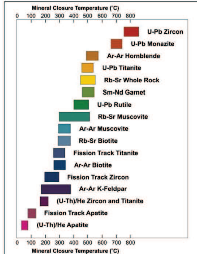
Figure 1.2.2. Estimations de la gamme de températures de fermeture effectives T_c pour différents systèmes thermochronométriques et divers minéraux. Ces gammes prennent en compte la variabilité des paramètres de diffusivité ( E_a , D_0 ) pour un type de minéral, ainsi que l'influence de la vitesse de refroidissement sur la température de fermeture. Modifiée d'après une figure disponible via http://su-thermochronology.syr.edu
