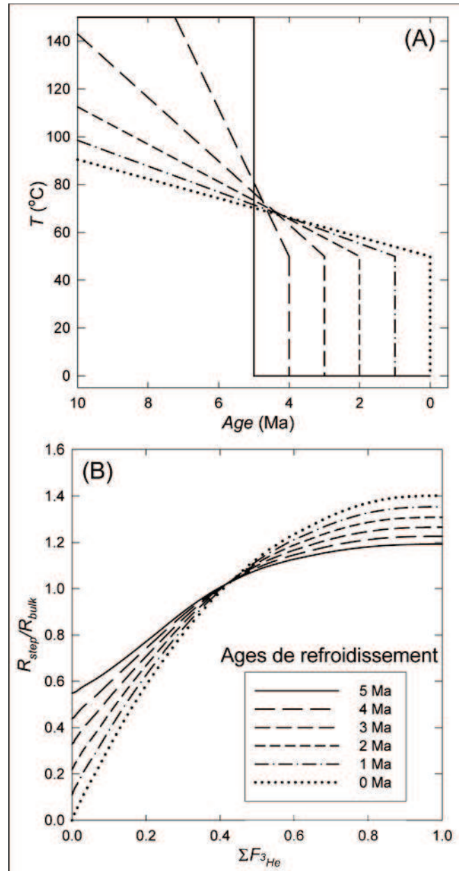
Figure I.2.5. Exemple théorique de la thermochronométrie ^4\text{He}^\beta\text{He} . A) Six histoires t - T synthétiques donnent un âge He similaire ( \sim 5 Ma), cependant le refroidissement terminal de l'échantillon intervient à des périodes différentes (de 5 Ma à l'actuel). B) La distribution spatiale du ^4\text{He} ( R_{step} = rapport ^4\text{He}^\beta\text{He} mesuré pour chaque étape de chauffage; R_{bulk} = rapport ^4\text{He}^\beta\text{He} moyen du grain d'apatite) au sein du grain d'apatite ( \Sigma F_{3_{He}} = 0 pour le début et 1 pour la fin de l'extraction de l'He) pour chaque chemin t - T est différente. Modifiée d'après Shuster and Farley [2005].
