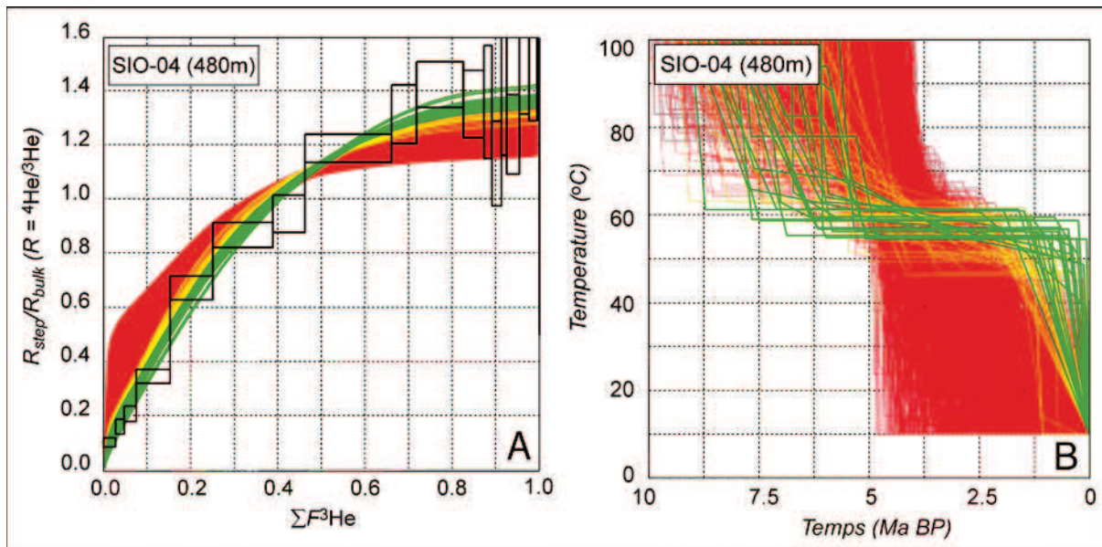
Figure 1.2.9. Exemple d'un spectre d'évolution en {}^4\text{He}^\beta/\text{He} lors d'une expérience de dégazage (A, rectangles ouverts indiquant l'incertitude sur la mesure) et prédictions obtenues par modélisation thermique inverse (courbes colorées). Chaque histoire thermique (B) est associée à un spectre d'évolution en {}^4\text{He}^\beta/\text{He} (les courbes vertes représentent des chemins t - T compatibles avec les données mesurées, tandis que les courbes jaunes et rouges illustrent respectivement les histoires de refroidissement partiellement et non compatibles avec les rapports {}^4\text{He}^\beta/\text{He} mesurés. Modifié d'après Valla et al. [submitted, a]
