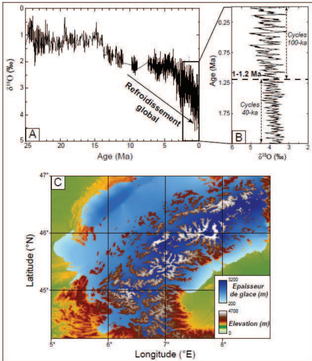
Figure I.1.1. A) Evolution du \delta^{18}O des sédiments marins, proxy de l'évolution du climat global (refroidissement global et augmentation de la variabilité climatique depuis \sim 5 Ma). B) Zoom sur la courbe d'évolution du \delta^{18}O des sédiments marins pour les derniers 2 Ma, illustrant la transition climatique mi-Pléistocène. Modifiées d'après Zhang et al. [2001] et Lisiecki and Raymo [2005]. C) Englacement des Alpes Européennes occidentales lors du Dernier Maximum Glaciaire (DMG \sim 20 ka). Modifiée d'après Ehlers and Gibbard [2004].
