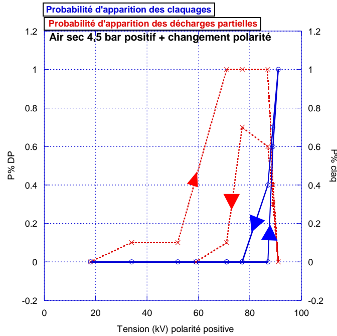
Figure 4.28. Phénomène d'hystérésis dans Air Sec à 4,5 bar, en tension impulsionnelle positive.
