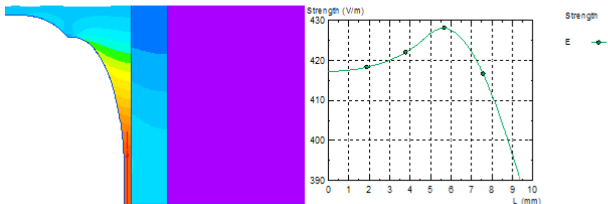
Figure 2.9. Répartition du champ électrique dans le cas d'une courbure ellipsoïdale
