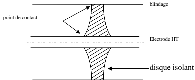
Figure 1.7. Exemple de points (ou jonctions) triples : le disque de support dans un PSEM.
