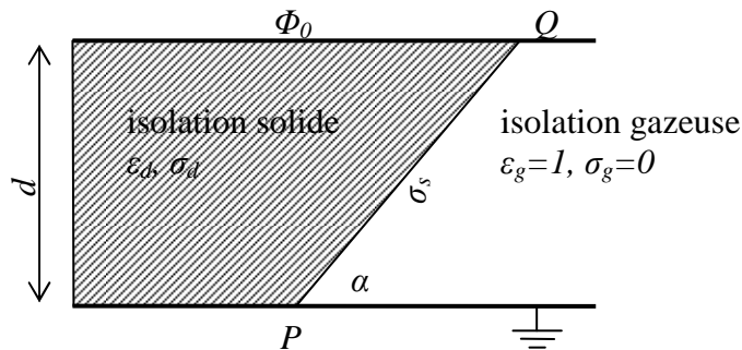
Figure 1.8. Schéma 2D utilisée dans les calculs d'un point triple [35].
