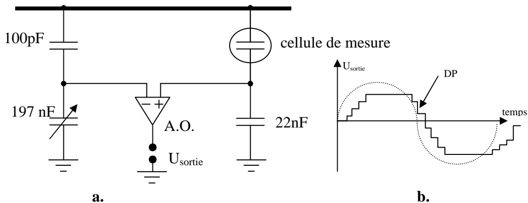
Figure 5.7. a. Circuit différentiel pour mesurer les DP ; b. signal théorique
