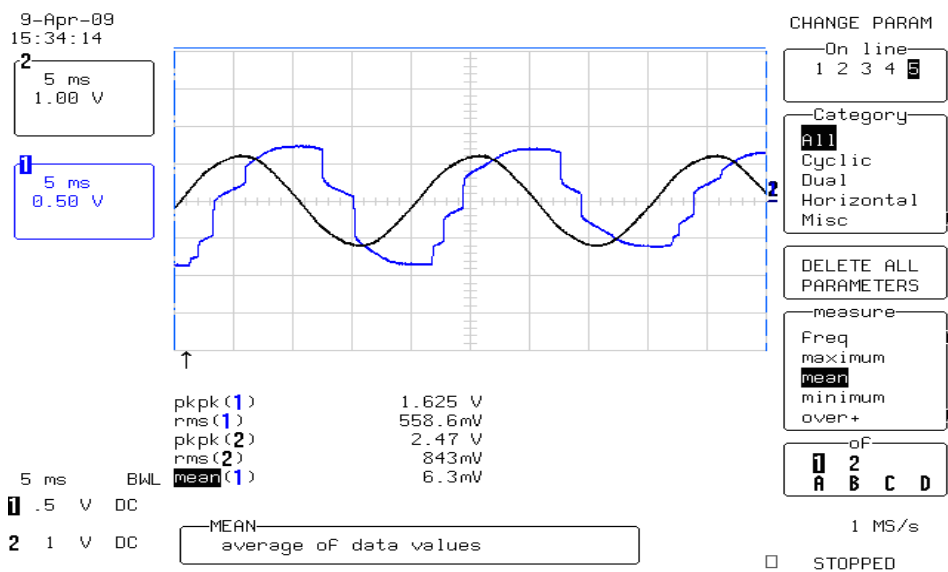
Figure 5.9. Le signal d'alimentation de la cellule (noir) et le signal de sortie de l'ampli op (bleu), qui est composé d'une tension résiduelle et de la tension donnée par les DPs.
