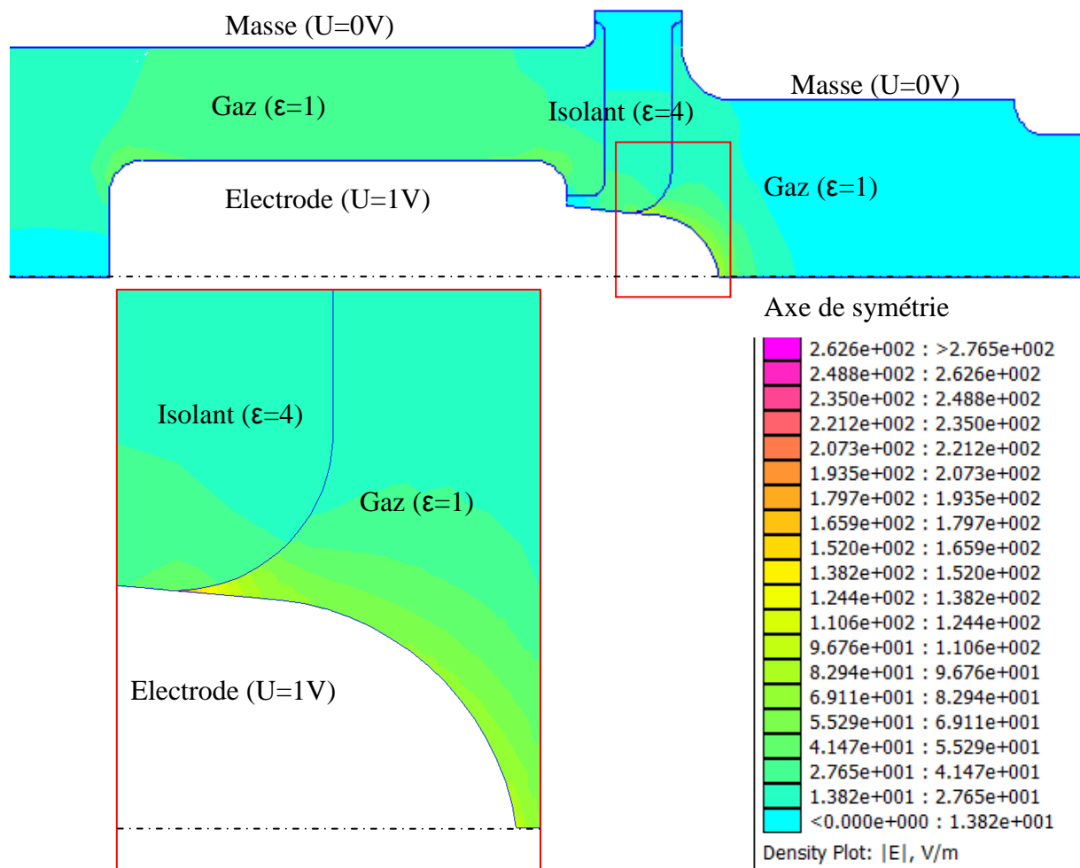
Figure 2.4. Résultat de la simulation des zones de champ renforcé pour l'ensemble de la cellule « AREVA » comprenant la géométrie PT. Détail de la zone du PT.
