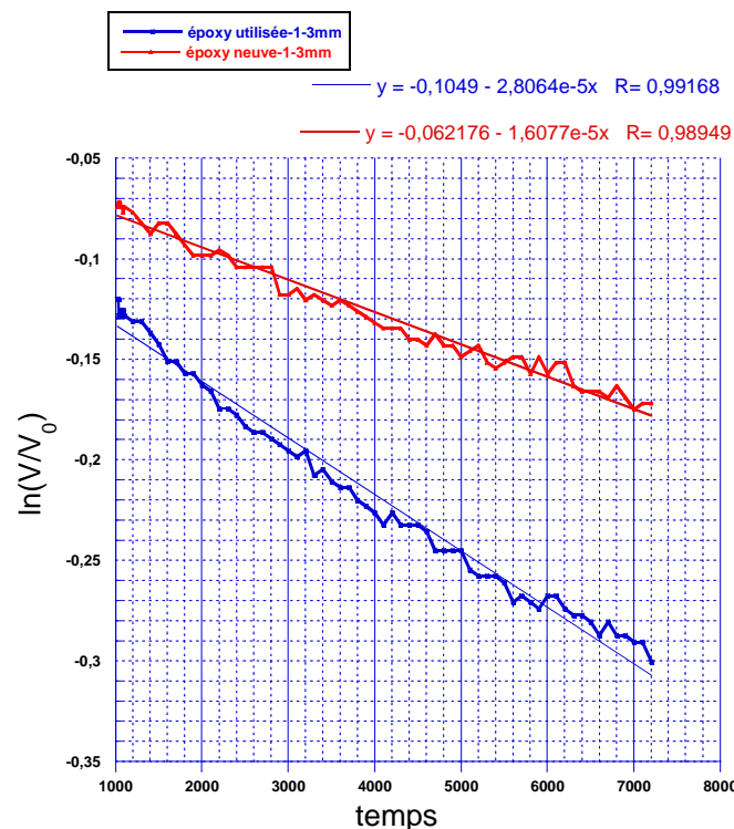
Figure 6.4. Mesures de déclin de potentiel pour deux échantillons de 3 mm en résine époxy.
