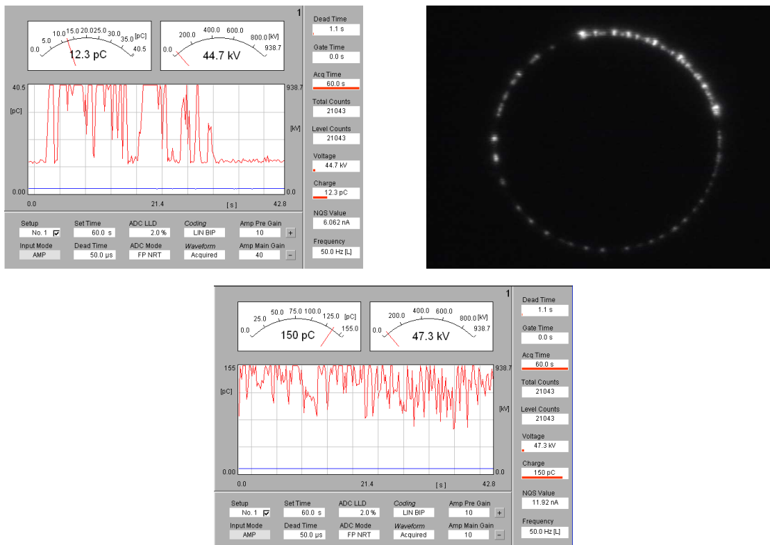
Figure 3.6. Régime de décharges de plus grandes amplitudes ( >50\text{pC} ) qui apparaît pour U_{\text{app}} \gg U_{\text{DP}} (instable à 44.7\text{kV} , quasi-stable à 47.3\text{kV} ). Gaz : Air Sec. Pression : 3,5\text{ bar} .
