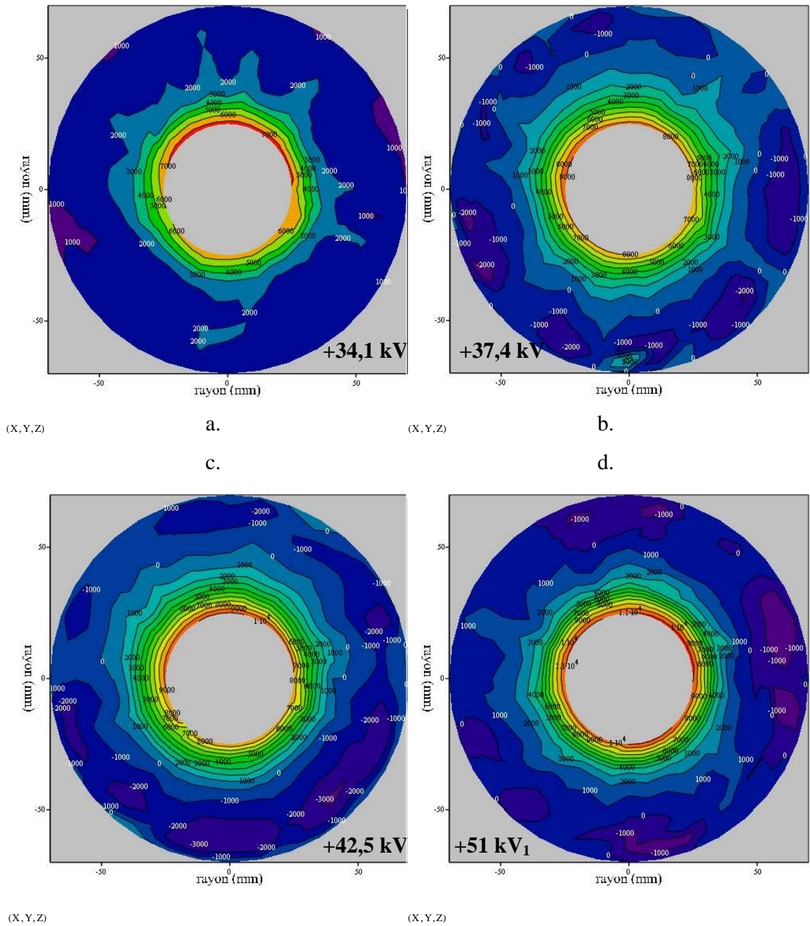
Figure 6.12. Potentiels mesurés sur la surface de l'isolant pour différentes impulsions de tension positive appliquées générant seulement des DP dans la zone du PT.
