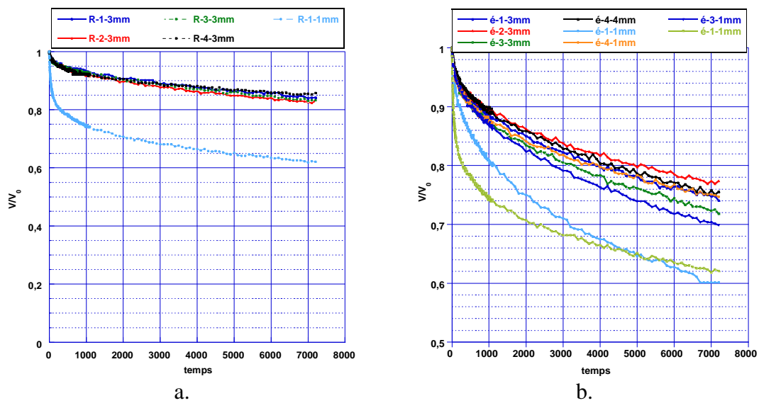
Figure 6.1. Mesures de déclin de potentiel des échantillons en résine époxy. a. résine époxy « neuve » ; b. résine utilisée 3 ans.
