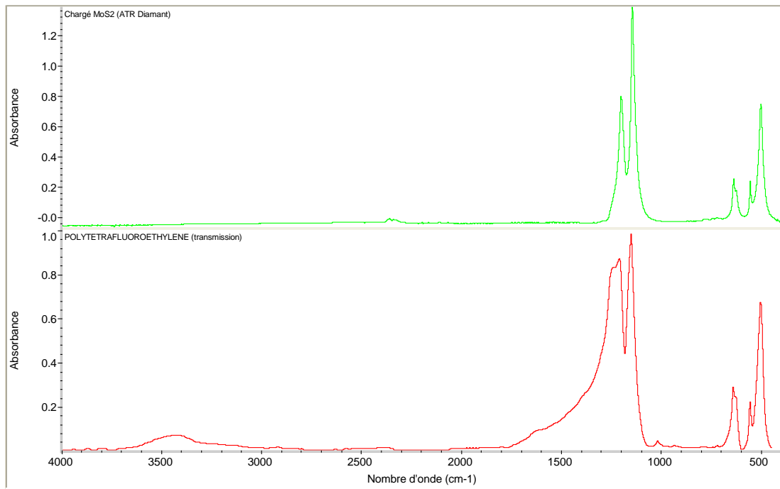
Figure 6.17. PETF chargé MoS 2 vs. PETF de la base de données
