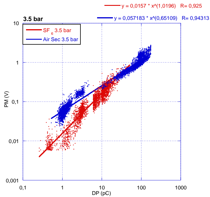
Figure 3.21. Variation de la réponse du PM en fonction des mesures de l'ICMSytem dans le SF6 et dans l'air sec. Pression utilisée : 3,5 bar.
