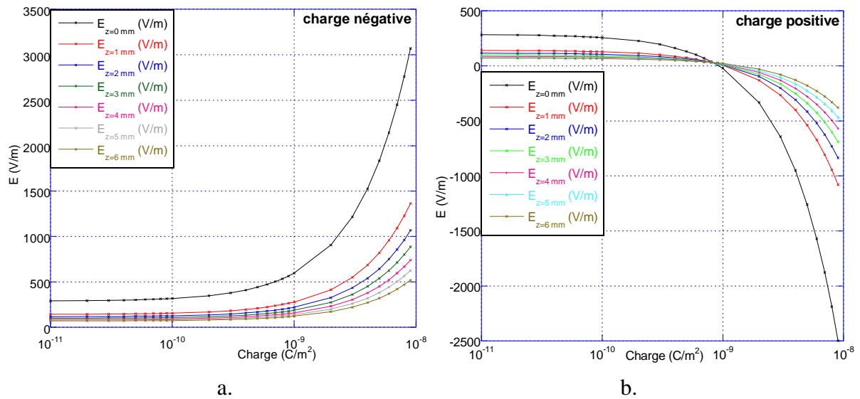
Figure 3.46. Le champ électrique en fonction de la charge déposée sur l'isolant pour différents points à partir du PT, en appliquant 1 V sur l'électrode centrale. a. Charge déposée négative ; b. Charge déposée positive.
