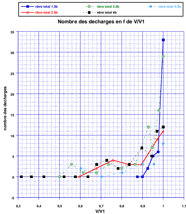
Figure 3.31. Résultats obtenus dans l'étude du point triple sous tension impulsionnelle dans le SF 6 . Nombre des décharges par impulsion en fonction du rapport de la tension à la tension de 100% probabilité ;
