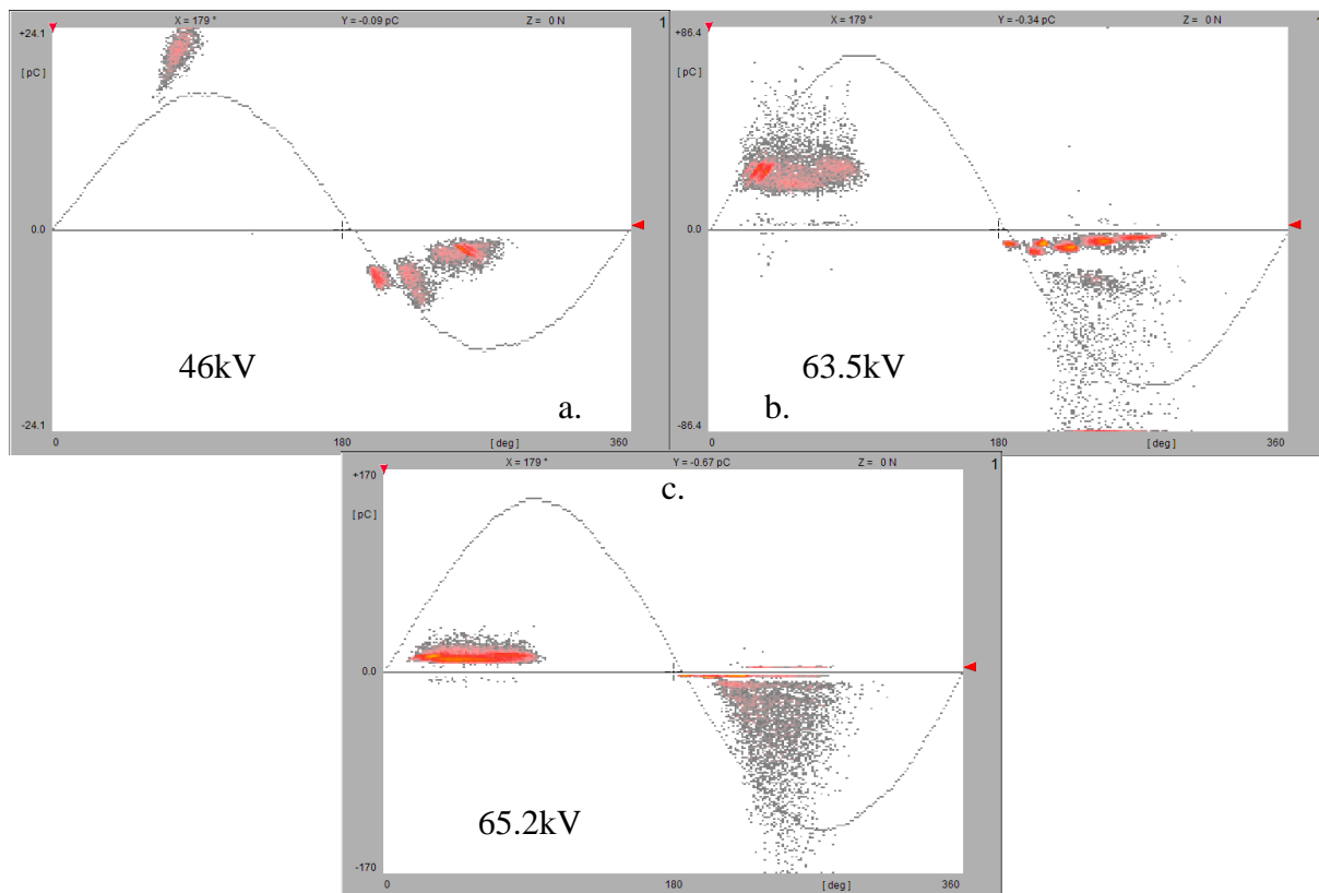
Figure 3.9. Enregistrement des DPs dans l'air sec à 3,5 bar.
