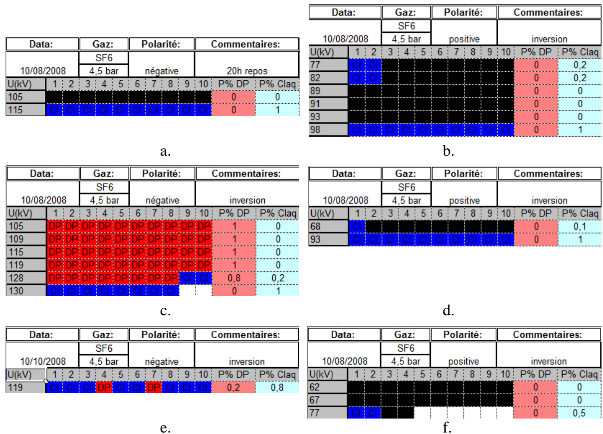
Figure 4.26. Essais en changeant la polarité de la tension appliquée dans le SF 6 , à 4,5 bars.
