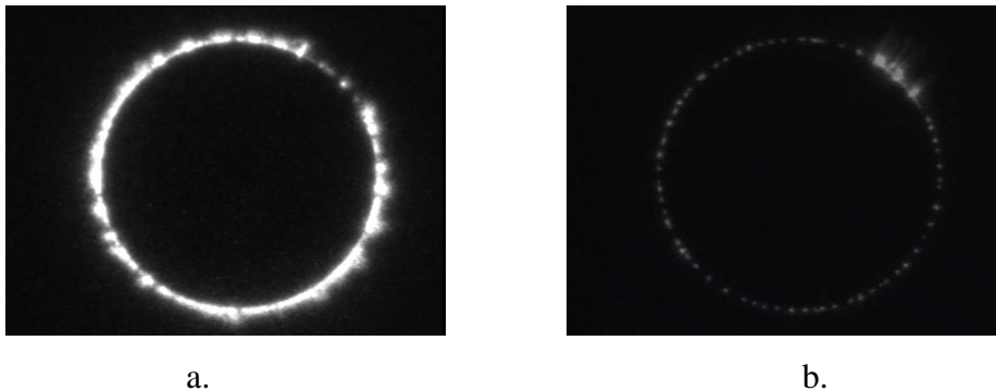
Figure 3.42. DPs sous tension impulsionnelle positive ;
