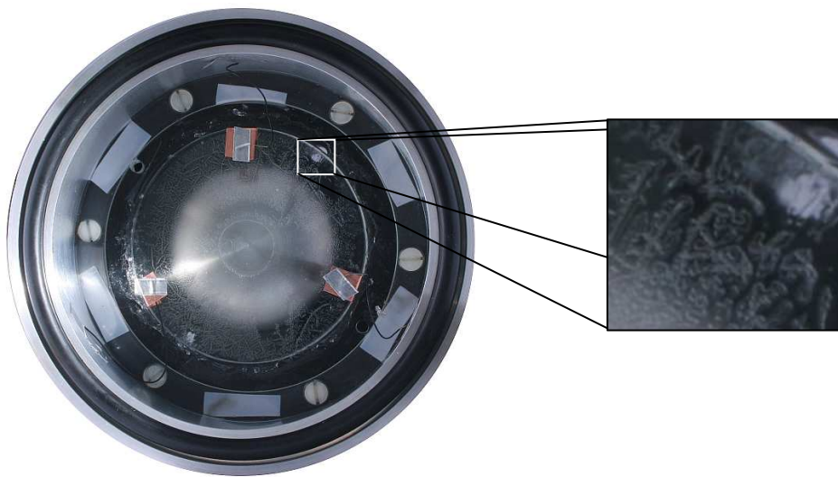
Figure 2.10. Vue de face de la cellule de mesure (champ électrique quasi-uniforme) ; détail montrant les bulles de gaz apparaissant entre la métallisation et le plexiglas.
