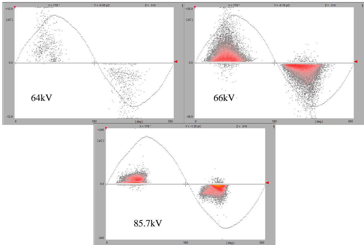
Figure 3.11. Enregistrement des DP dans le SF 6 à 1,5 bar.
