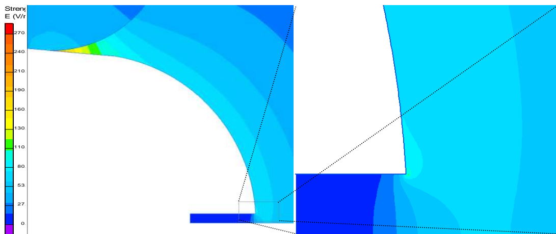
Figure 3.37. Résultats de la simulation du champ électrique dans la région du trou taraudé de l'électrode centrale ; a. vue d'ensemble ; b. détail de la zone de l'arrête du trou.
