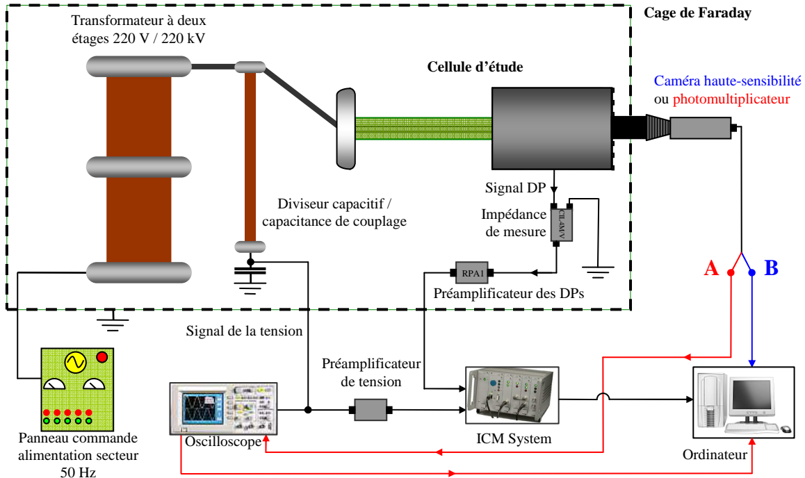
Figure 2.11. Schéma de détection, mesure et visualisation des DP's en tension alternative.
