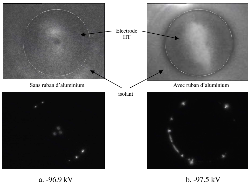
Figure 3.38. Images des décharges pour : a. sans ruban d'aluminium sur le trou central et, b. avec un ruban d'aluminium collé sur le trou central..
