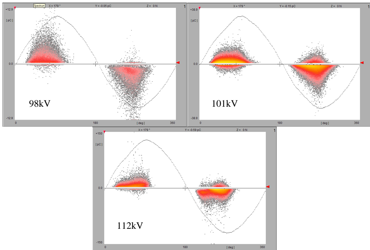
Figure 3.12. Enregistrement des DP dans le SF 6 à 2,5 bar.
