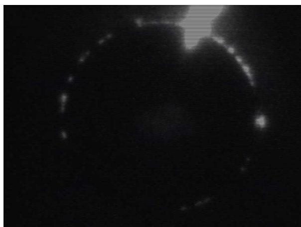
Figure 3.7. Image montrant le claquage (en haut à droite) détecté par la caméra CCD haute-sensibilité, correspondant à la tension de claquage U_b . Gaz : \text{SF}_6 ; Pression : 4,5\text{ bar} . U_{\text{app}} = 157\text{ kV} crête.
