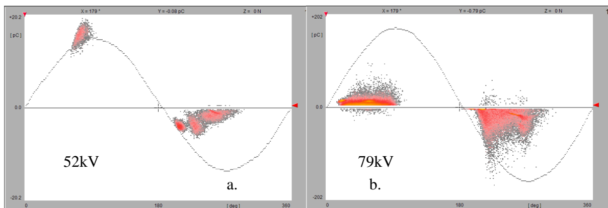
Figure 3.10. Enregistrement des DPs dans l'air sec à 4,5 bar.
