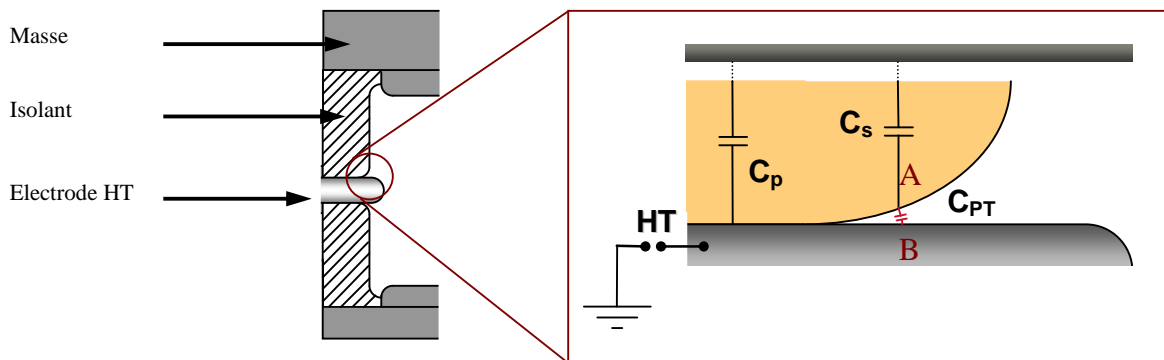
Figure 1.9. Représentation schématique de la zone du PT de la cellule d'essai.
