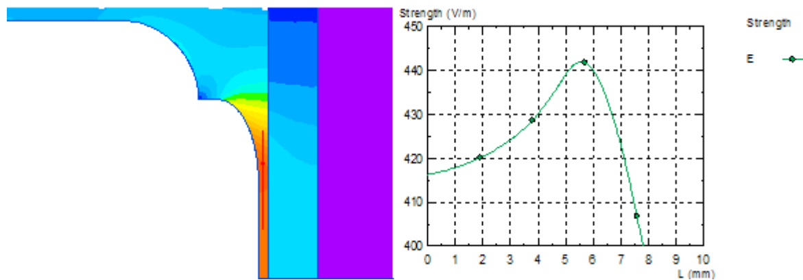
Figure 2.8. Répartition du champ électrique dans le cas d'une courbure ellipsoïdale
