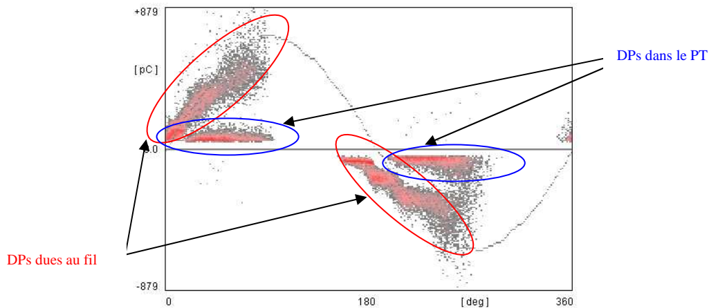
Figure 4.3. Enregistrement typique des DPs synchronisées avec la phase de la HT. Air sec, P=1,5 bar et U_{app}=37,5kV .
