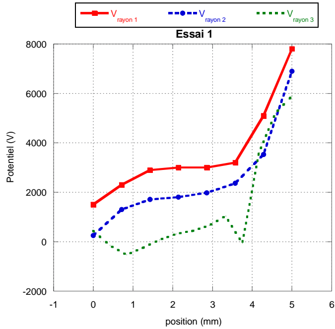
Figure 6.6. Mesure du potentiel de surface sur les rayons de l'isolant (Voir figure 7). Air atmosphérique. U_{app}=34kV .
