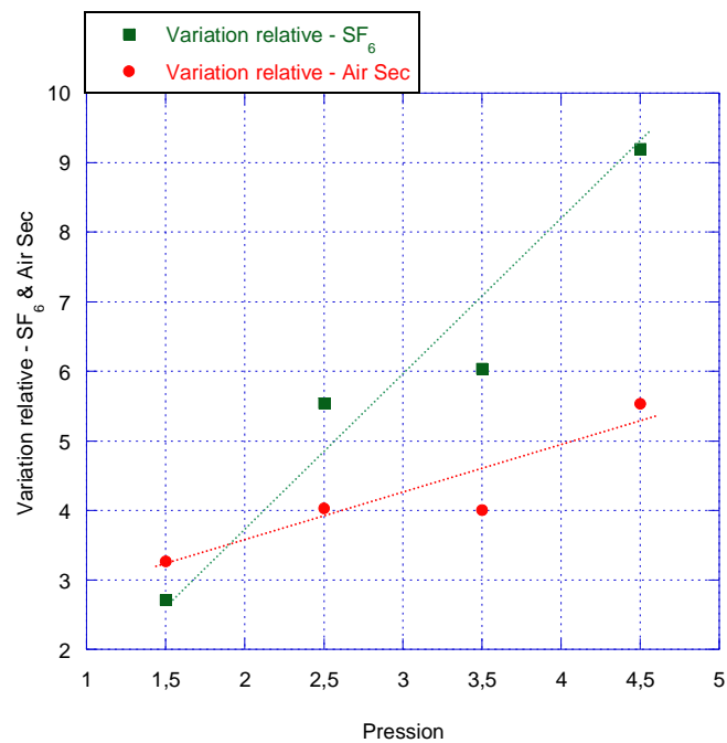
Figure 4.12. Variation relative de l'U b pour l'air et le SF 6 .
