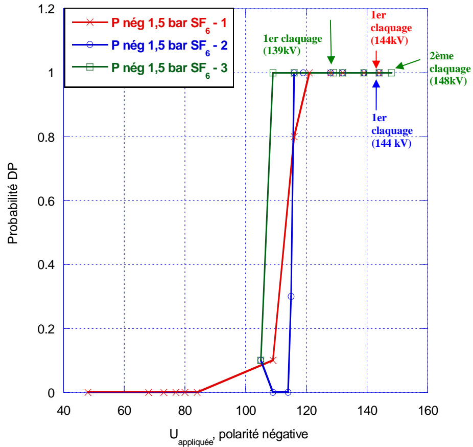
Figure 4.14. Probabilité d'apparition des DP en fonction de la tension impulsionnelle appliquée, pour la géométrie avec défaut, SF 6 , à 1,5 bar
