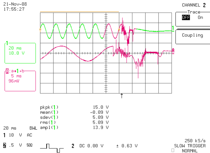
Figure 4.13. Claquage dans l'air sec à 1,5 bar. Les amorçages successifs sont très nombreux.
