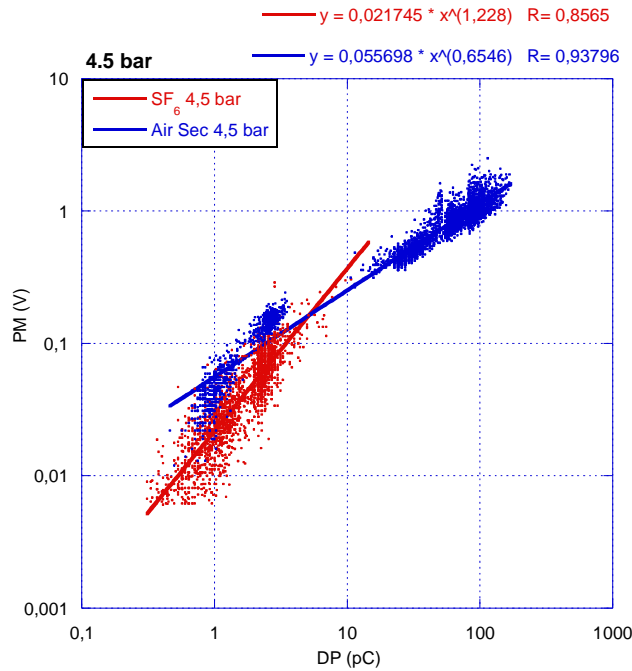
Figure 3.22. Variation de la réponse du PM en fonction des mesures de l'ICMSystem dans le SF6 et dans l'air sec. Pression utilisée : 4,5 bar.
