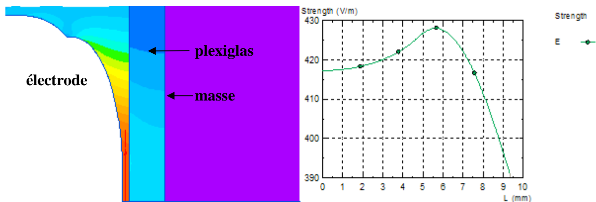
Figure 5.4. Répartition du champ électrique dans le cas d'une courbure ellipsoïdale
