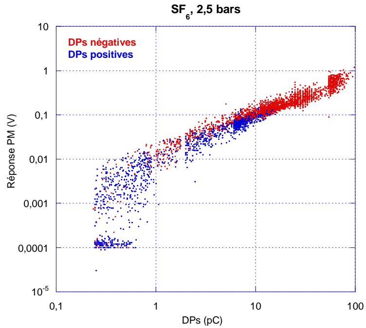
Figure 3.16. Signal du PM en fonction de la valeur de la charge détectée par l'ICMSystem. Gaz : SF6 à 2,5 bar.
