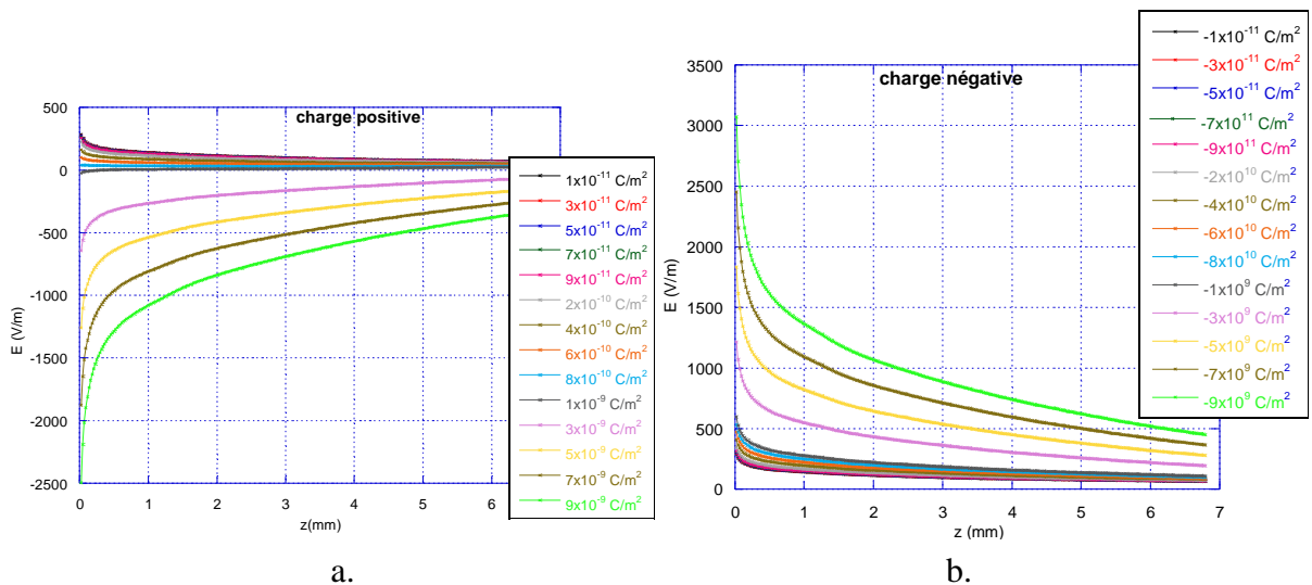
Figure 3.47. Le champ électrique en fonction de la distance du PT pour différentes valeurs de charges déposées sur la surface de l'isolant, en appliquant 1 V sur l'électrode centrale. a. Charge déposée négative ; b. Charge déposée positive.
