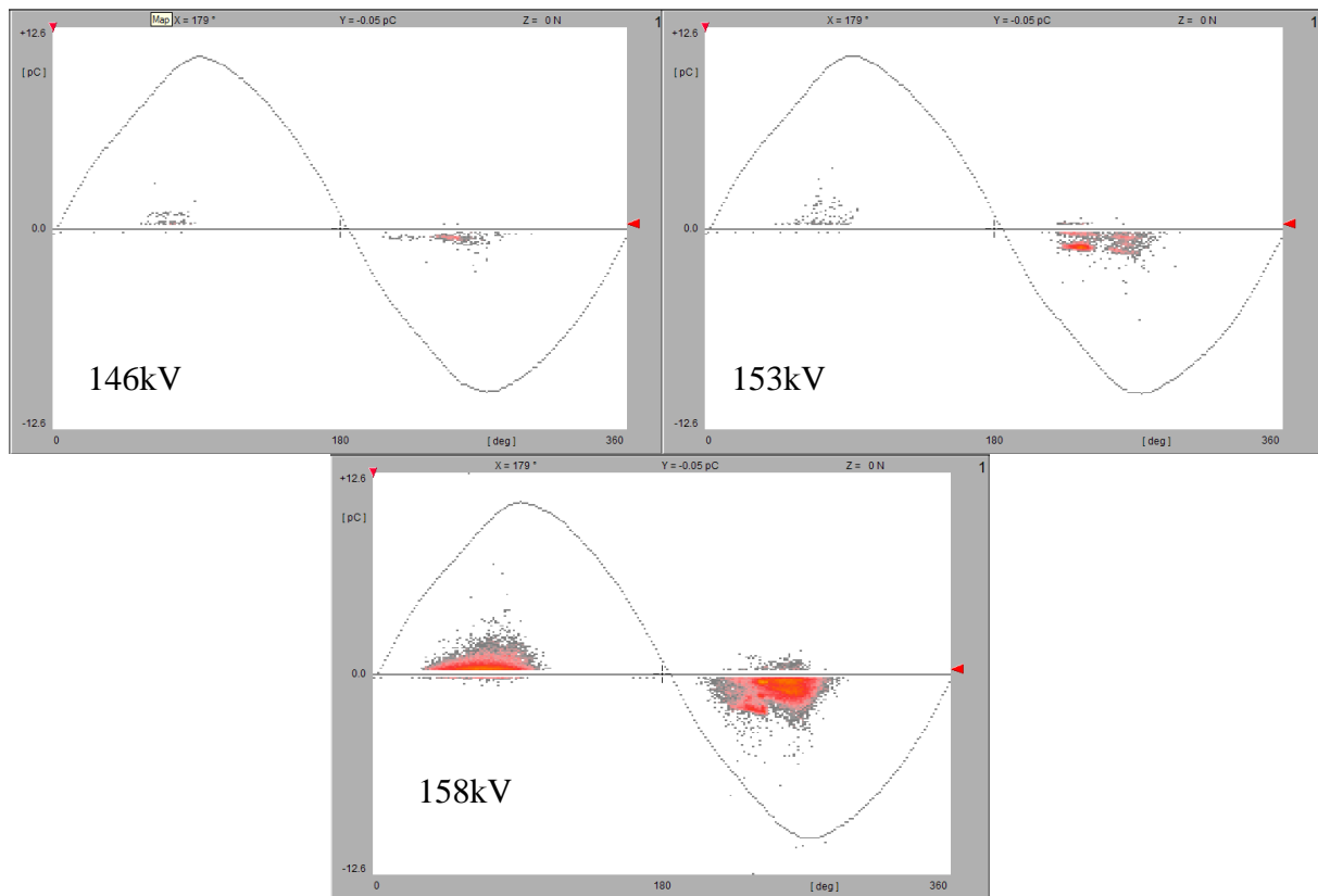
Figure 3.14. Enregistrement des DPs dans le SF 6 à 4,5 bar.
