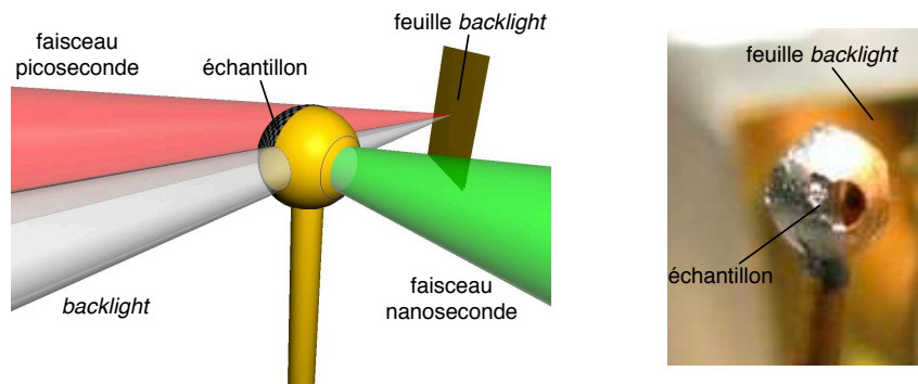
Fig. 6.3 – Gauche : schéma de principe d'utilisation des cibles. Le faisceau nanoseconde (en vert) de chauffage est focalisé sur le trou d'entrée laser \phi 700 \mu\text{m} . La focalisation sur une feuille d'or du faisceau picoseconde (en rouge) est à l'origine du faisceau de radiographie ( backlighter en gris). Les trous de diagnostics \phi 500 \mu\text{m} définissent la partie du flux de radiographie d'intérêt. Droite : photographie des cibles (feuille de conversion au fond). L'échantillon est déposé sur la moitié du trou de diagnostic de sortie.
