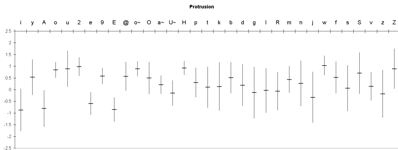
FIG. 4.10 – Mesures de la protrusion (valeurs centrées réduites de la moyenne et de l'écart type) pour chaque phonème d'un grand corpus (Alphabet phonétique SAMPA - cf. Annexe A).
