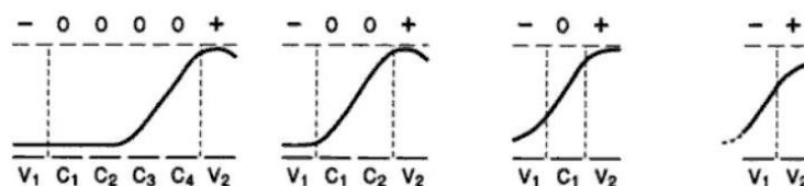
FIG. 2.3 – Evolution de la protrusion dans une séquence /iC..Cu/ selon le modèle Time-Locked d'après E.Farnetani et D. Recasens [32].
