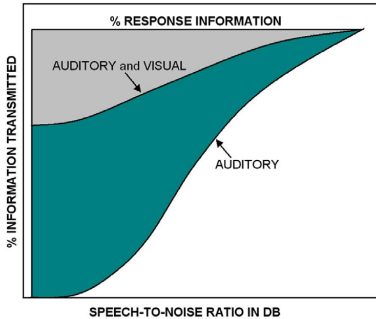
FIG. 3.1 – Contributions du message oral et visuel à l'intelligibilité en fonction du ratio Signal/Bruit (De Sumbly et Pollack [81]).
