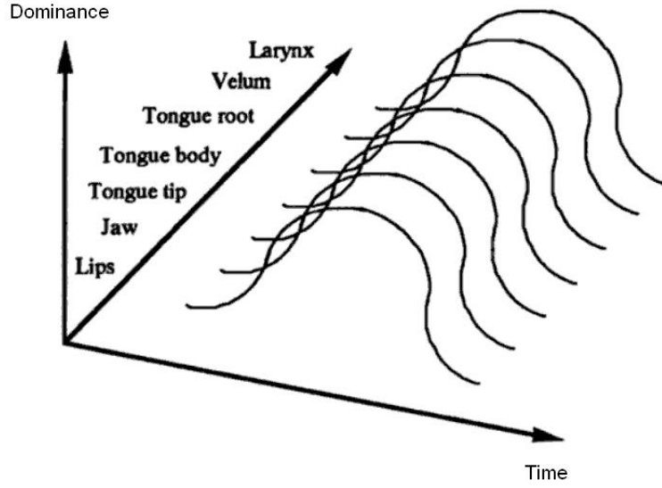
FIG. 3.8 – Influence simultanée des différents articulateurs. Schéma extrait de Lófqvist [51].
