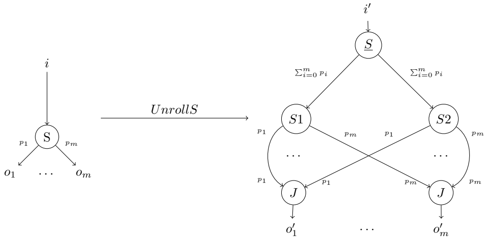
FIGURE 3.12 – Déroulage d'un nœud Split.
