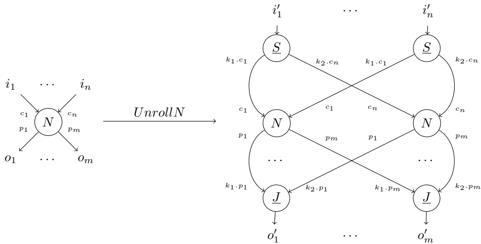
FIGURE 3.13 – Patron général de la transformation de déroulage. Le nœud N peut être remplacé par n'importe quel nœud pur. Les k_i \in \mathbb{N} représentent le nombre de blocs envoyés à chaque instance du nœud déroulé.
