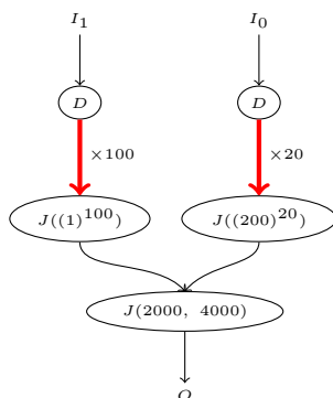
FIGURE 2.28 – Filtre de Hough en SLICES et le graphe SJD compilé.
