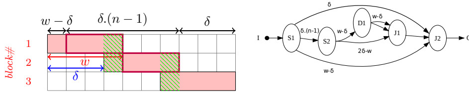
FIGURE 2.18 – Extraction des blocs avec recouvrement partiel ( 1 < \frac{w}{\delta} < 2 )
