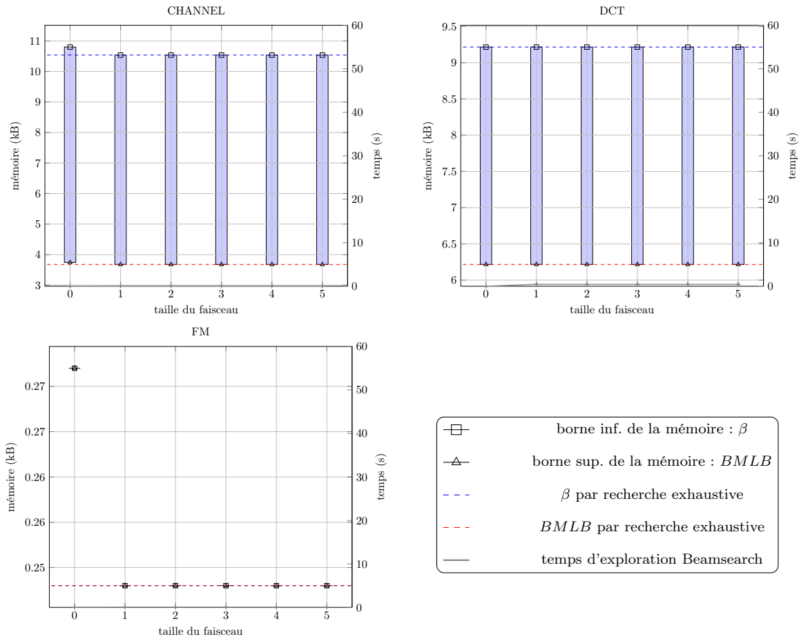
FIGURE 4.7 – Réduction mémoire sur les programmes CHANNEL, FM et DCT. Ces programmes admettent peu de transformations. Le nombre de candidats engendrés est très faible et les réductions mémoire affichées sont négligeables. Pour chaque taille de faisceau on a délimité l'espace entre la borne inférieure et la borne supérieure de la mémoire par une barre verticale ; les bornes mémoire se lisent sur l'échelle gauche. Lorsqu'elles sont connues, on a représenté les bornes inférieures et supérieures optimales obtenues par recherche exhaustive par les pointillées en rouge et en bleu. Enfin le temps d'exploration pour les différentes tailles de faisceau est donné par la ligne brisée grise et se lit sur l'échelle droite ; pour CHANNEL, FM et DCT le temps d'exploration est très court et se confond avec l'axe des abscisses.
