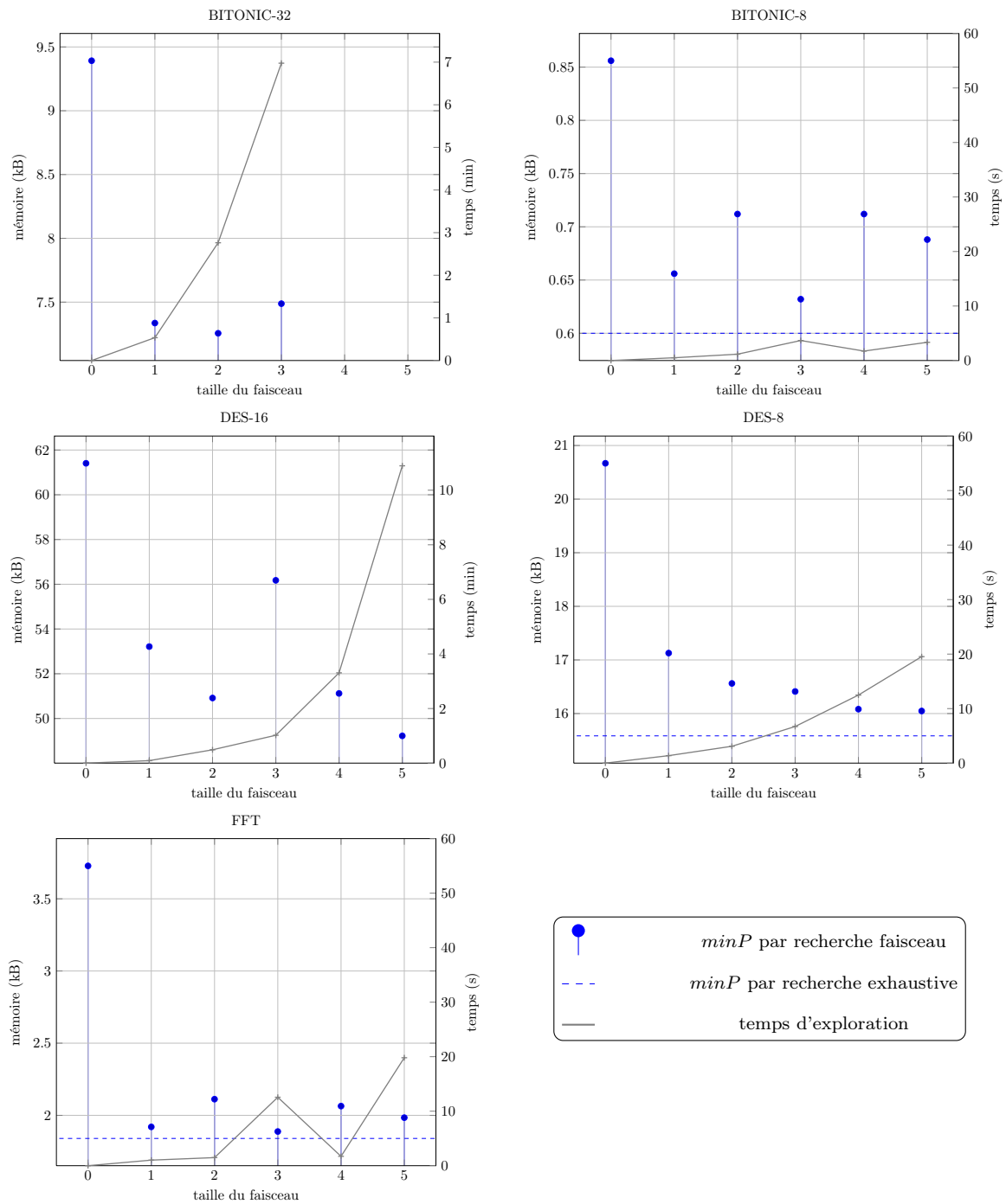
FIGURE 4.12 – Réduction de minP (calculé avec la méthode de Choi) sur 4 cœurs pour les programmes de la suite StreamIt. Pour chaque taille de faisceau on a représenté la taille minP obtenue par les barres verticales. Lorsque le minP optimum obtenu par recherche exhaustive est connu, il est indiqué par les pointillées. Enfin le temps d'exploration pour les différentes tailles de faisceau est donné par la ligne brisée grise et se lit sur l'échelle droite.
