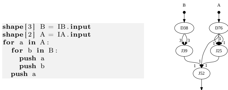
FIGURE 2.22 – Compilation des nids de boucles : à gauche, un exemple de nids de boucles, à droite, le sous-graphe SJD correspondant.
