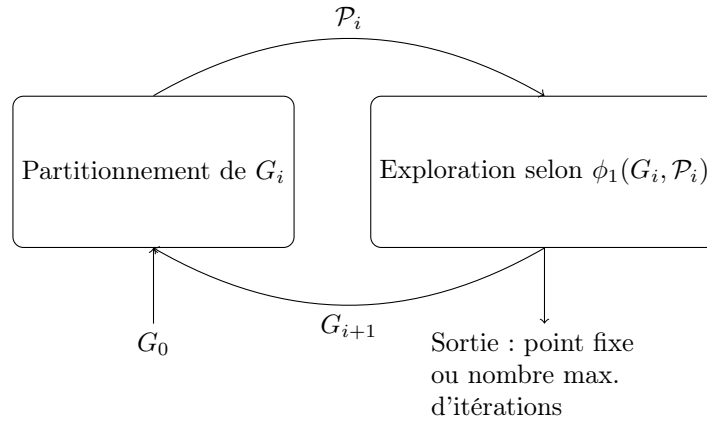
FIGURE 4.16 – L’exploration itérative permet de prendre en compte le partitionnement pour le calcul de \phi .
