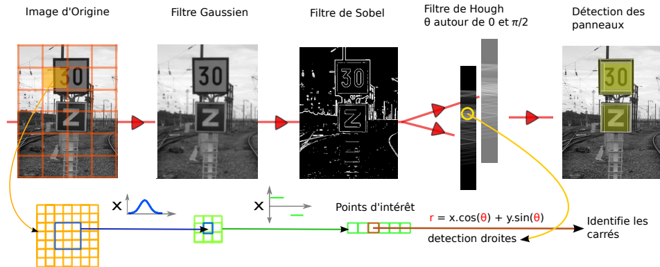
FIGURE 2.1 – Chaîne pour la détection de de panneaux ferroviaires (photographie d'Aurélien Braidà)
