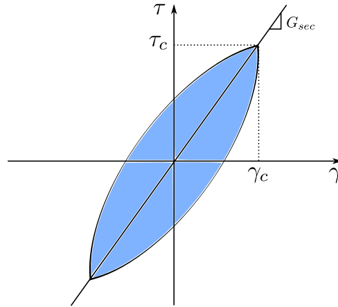
FIGURE 1.1 – Définition des paramètres de l'approche linéaire équivalente
