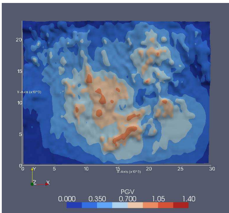
FIGURE 2.13 – Peak Ground Velocity (PGV) dans le cas non linéaire pour une modélisation à 0.6 Hz.
