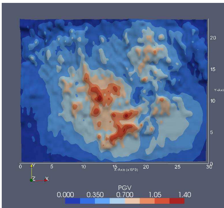
FIGURE 2.12 – Peak Ground Velocity (PGV) dans le cas linéaire pour une modélisation à 0.6 Hz.
