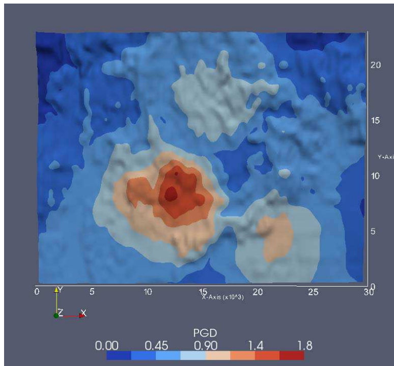
FIGURE 2.10 – Peak Ground Displacement (PGD) dans le cas linéaire pour modélisation à 0.6 Hz.
