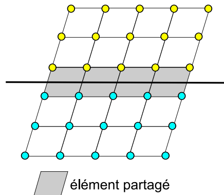
FIGURE 1.2 – Schéma de la méthode de partitionnement element-cut .
