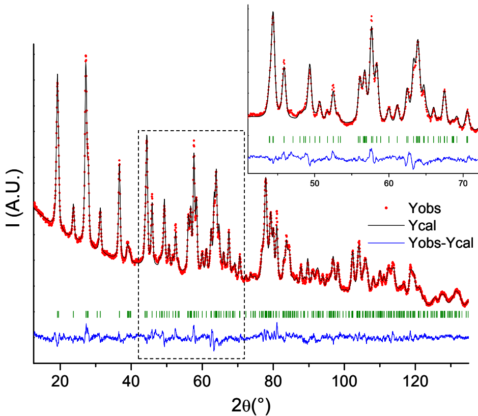
Figure IV.6 : Comparaison des diffractogrammes neutrons expérimental et calculé de la phase \text{FePO}_4 \cdot \text{H}_2\text{O} . Un agrandissement de la figure dans l'intervalle 41-72^\circ ( 2\theta ) est également donné.
