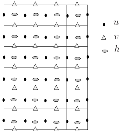
FIG. 21.2 – Maillage de \Omega
