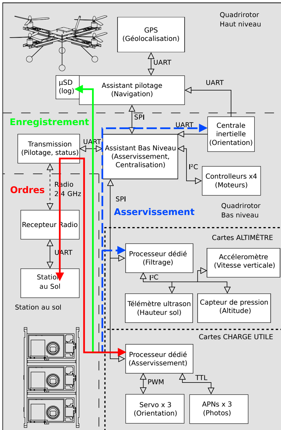
FIGURE 3.23 – Différentes liaisons entre la charge utile et les autres sous-systèmes Source : ©ATIS
