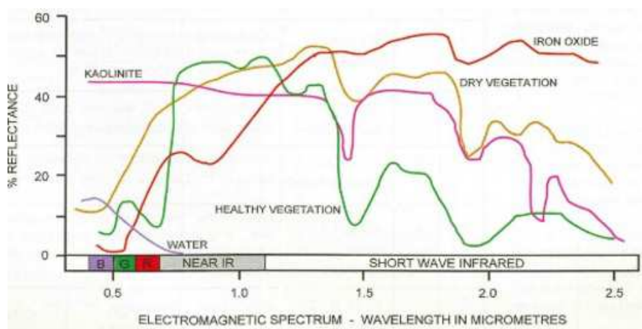
FIGURE 1.10 – Signatures spectrales de sources naturelles entre 400 et 2500 nanomètres. On remarquera la différence de signature entre la végétation chlorophyllienne active et la végétation sèche. Source : Geoimage, geoimage.com.au
