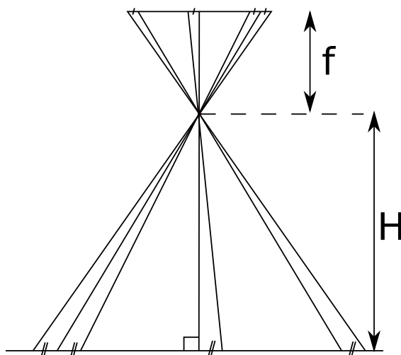
FIGURE 2.42 – Variation de la taille de l'échantillon au sol lors d'une prise de vue nadir Source : Gademmer
