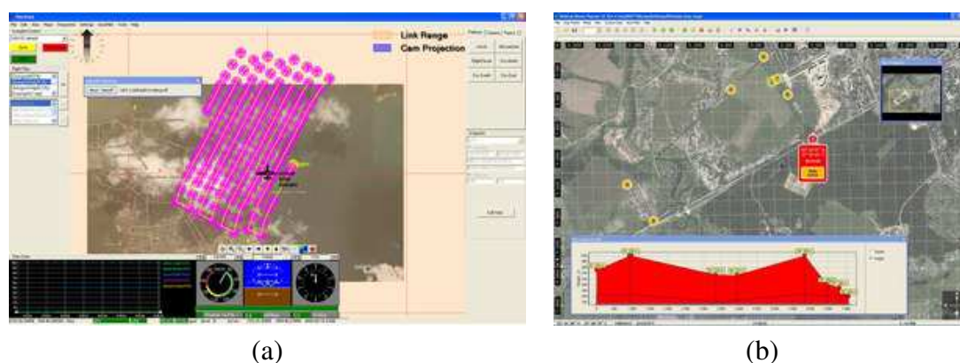
FIGURE 3.35 – Programmation du plan de vol. — (a) Les passages successifs au-dessus de la zone sont programmés afin d'assurer un recouvrement minimal entre les photographies. Source : gisondemand.blogspot.com — Lorsque l'information est disponible, une représentation du relief permet d'estimer l'altitude de vol, compromis le plus favorable entre la sécurité de l'appareil et l'homogénéité d'échelle des images. Source : www.tekno1.ru
