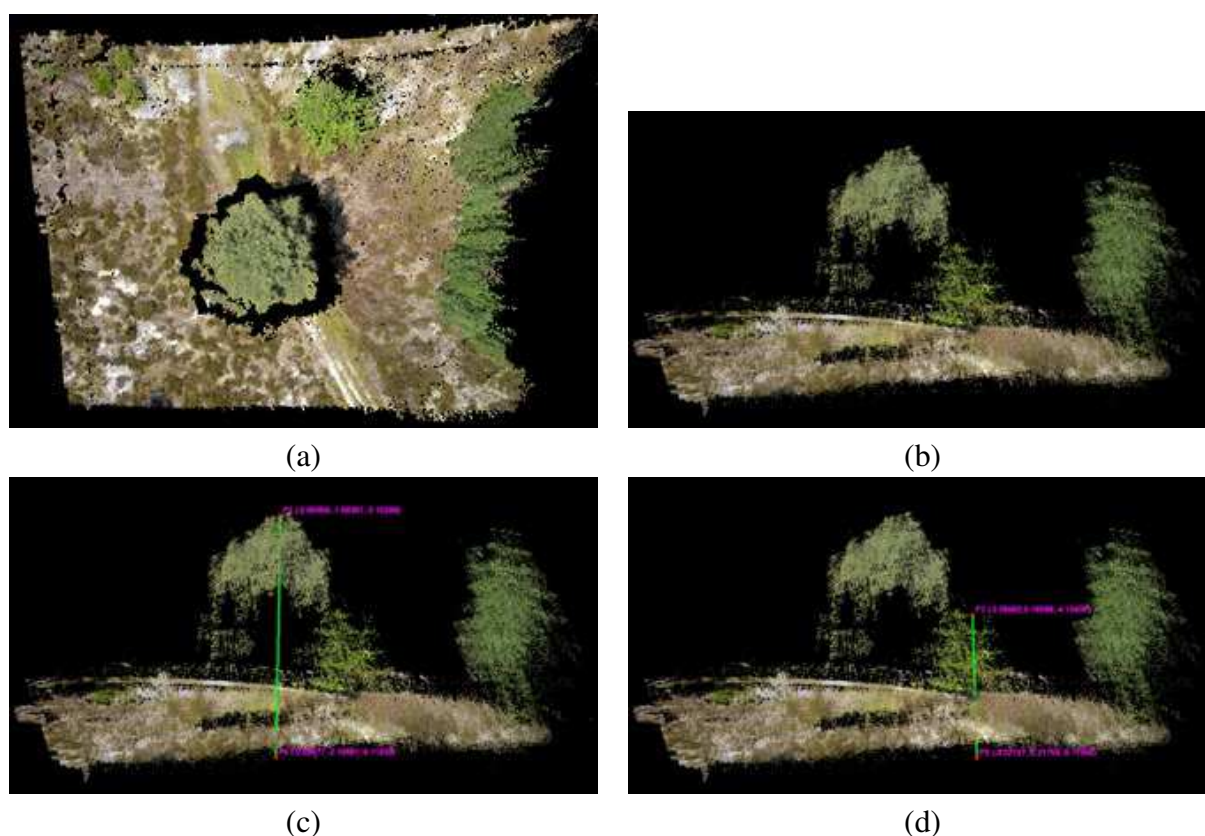
FIGURE 4.23 – Nuage de point 3D obtenu par Petitpas et al. [2010a] à partir du couple d'images précédent. — (a) Vue verticale — (b) Vue en coupe. — (c&d) Mesures de distance Source : ©ATIS/Gademer
