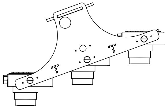
FIGURE 3.13 – Compensation de l'inclinaison en tangage de l'appareil. Source : Gademer
