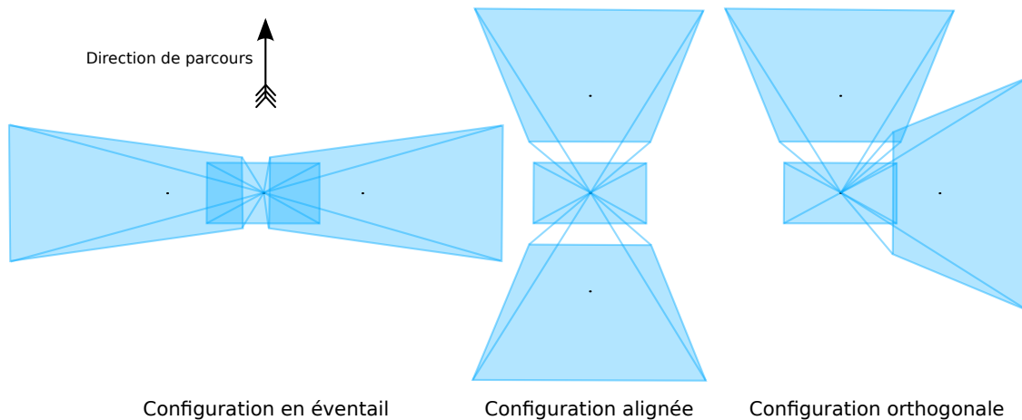
FIGURE 3.10 – Différentes configurations possible pour un système tri-caméras
