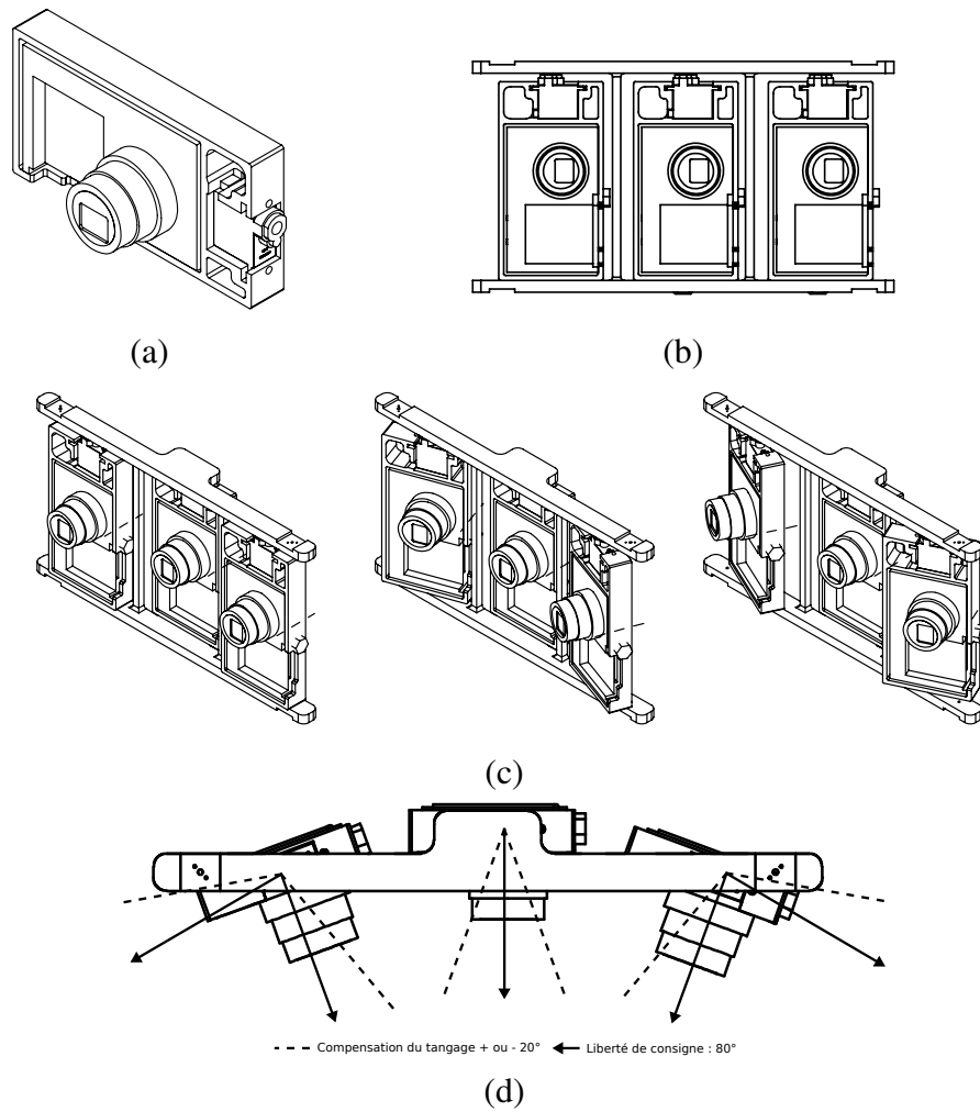
FIGURE 3.12 – (a) Association de l'appareil photographique et du servo-moteur (à droite) — (b) Les trois appareils sont alignés dans l'axe de vol — (c) Grâce aux servo-moteurs, l'orientation relative des appareils est configurable en fonction des besoins. — (d) Illustration des angles de débattement autorisés par les servo-moteurs. Source : Gademer
