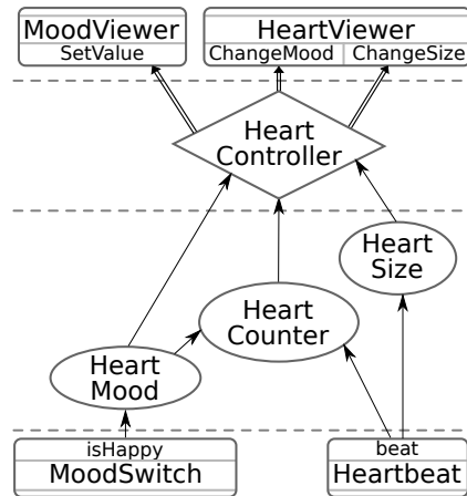
FIGURE 21: L'application cœur décrite avec DiaSpec
