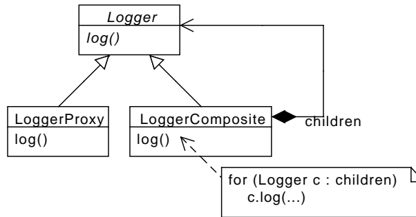
FIGURE 15: Utilisation du motif de conception Composite pour interagir avec les entités Logger
