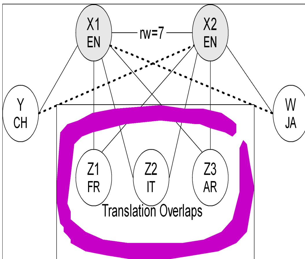
Fig. 45: MPG expansion
