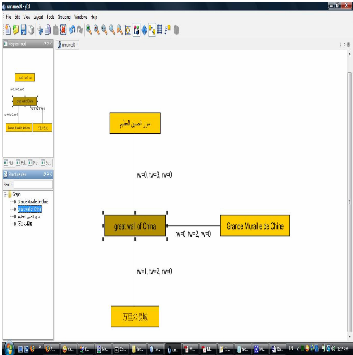
Fig. 48: Sample MPG
