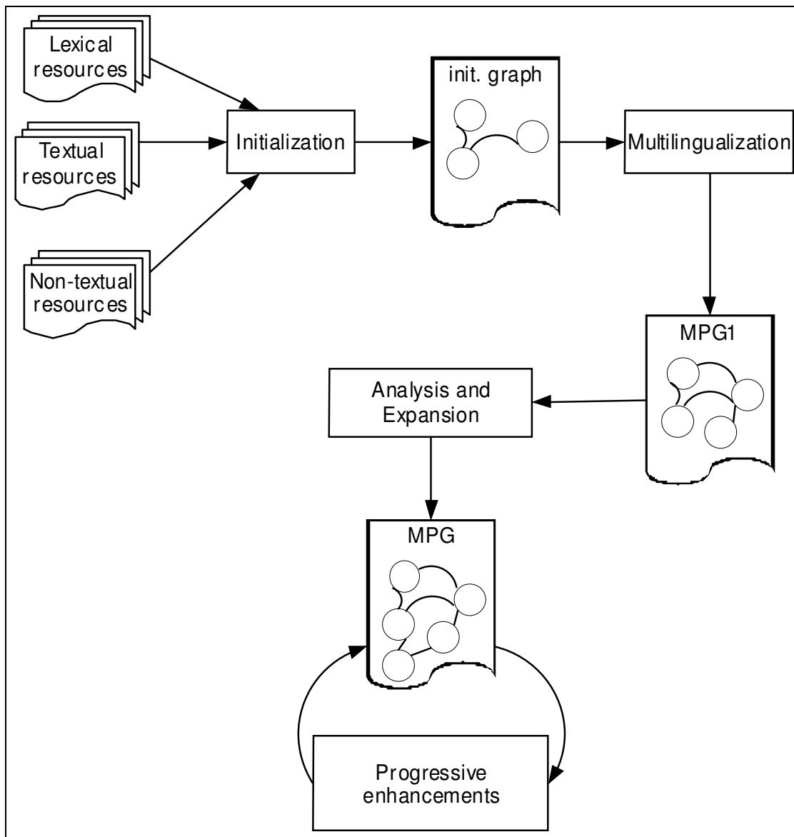
Fig. 37: MPG construction
