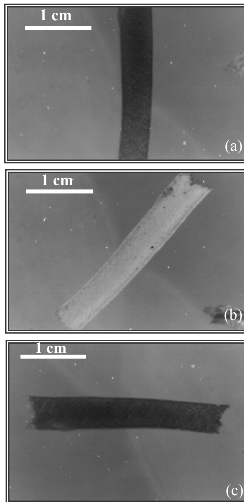
Figure III.24 : Photographie de microscopie optique à lumière polarisée d'un ruban de nanotubes de carbone. Le polariseur et l'analyseur sont en position croisée à 90°. (a) : Le ruban est dans l'axe du polariseur. (b) : Le ruban est incliné de 45° par rapport aux polariseurs. (c) : Le ruban est dans l'axe de l'analyseur.
