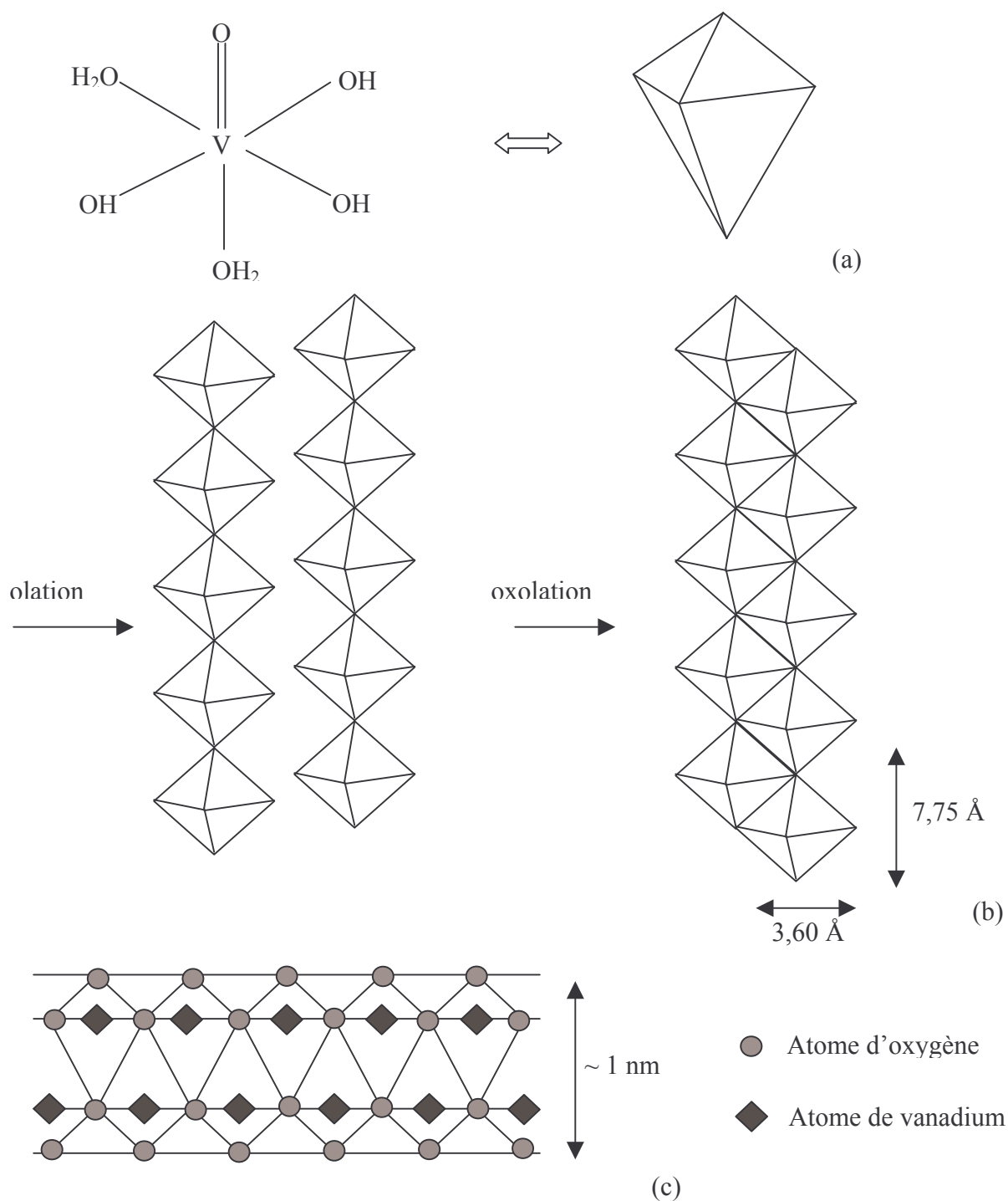
Figure II.1 : Formation et structure des rubans de V_2O_5 . (a) : Formule développée et structure tridimensionnelle du précurseur neutre des rubans. (b) : Réaction d'ololation suivie d'une oxolation conduisant à la formation d'un ruban. (c) : Structure d'un ruban de V_2O_5 .
