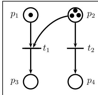
FIGURE 3.1 – Exemple de réseau de Petri
