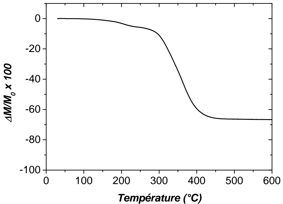
Courbe thermo-gravimétrique d'une poudre de nanotubes monoparoi Hipco (#R0211). Expérience réalisée sous air.
