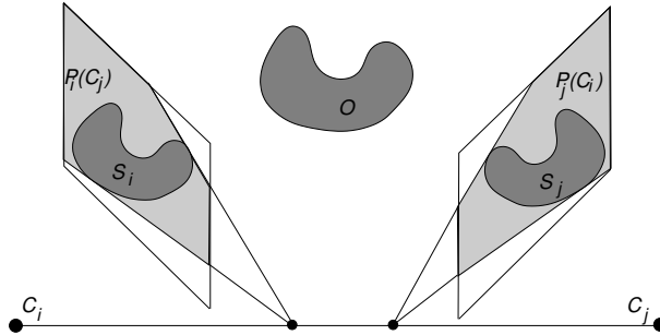
FIG. 3.2 – Dans l'image i , à gauche, la silhouette S_j est incluse dans la projection P_i(S_j) du cône associé à la silhouette S_j et inversement dans l'image j à droite.
