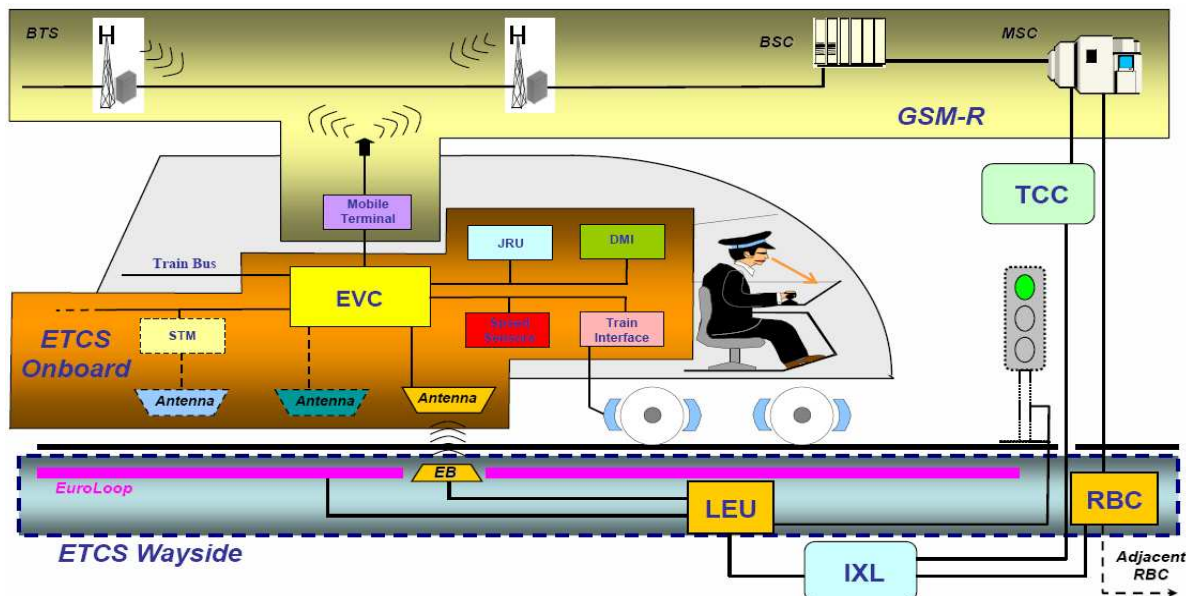
Figure 1.8: Architecture ETCS niveau 2 [Lévêque, 2007]
