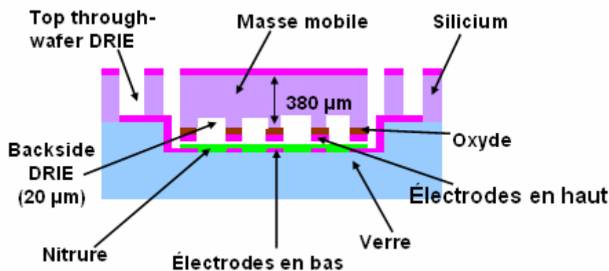
Fig. 11 Structure modifiée
