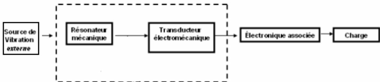
Fig. 2 Architecture générale d'un convertisseur d'énergie mécanique en énergie électrique
