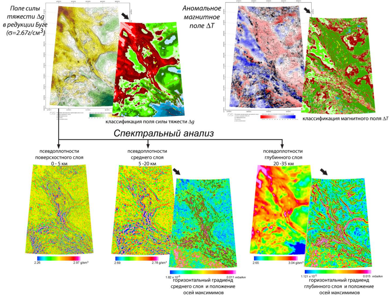
Рис. 3.10 Примеры различных типов трансформаций потенциальных полей для Енисейского кряжа и сопредельных территорий.
