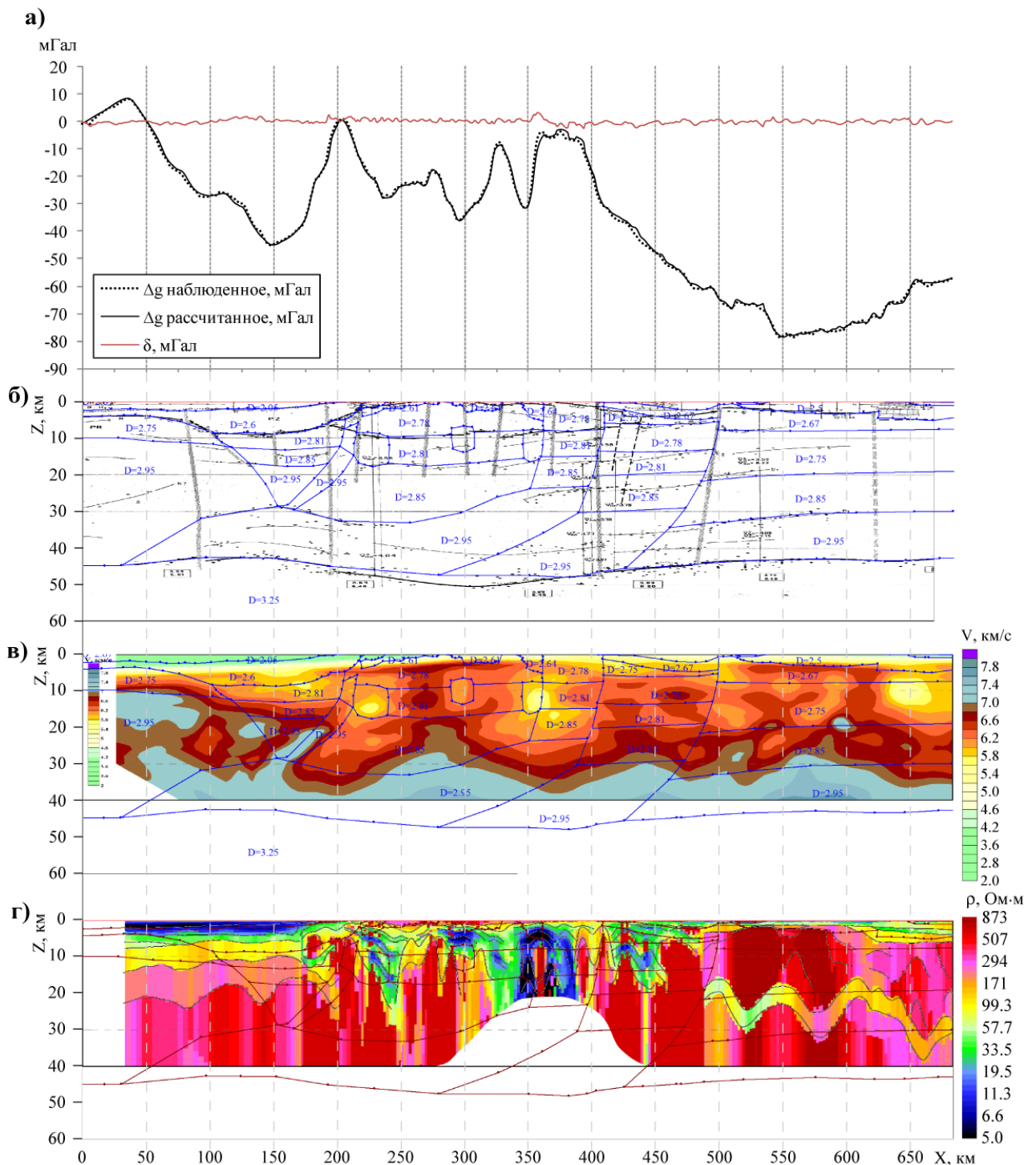
Рис. 3.16 Сопоставление результатов интерпретации методами гравиразведки, сейсморазведки и электроразведки а) плотностной модели вдоль геотраверса «Батолит» (синие линии на рисунках (б), (в) и зеленые на рисунке (г) линии, цифрами обозначены плотности блоков, г/см^3 ) с б) результатами интерпретации данных ГСЗ (Егоркин, 1982), в) данными сейсмотомографии и г) данными МТЗ (Фельдман, 2007)
