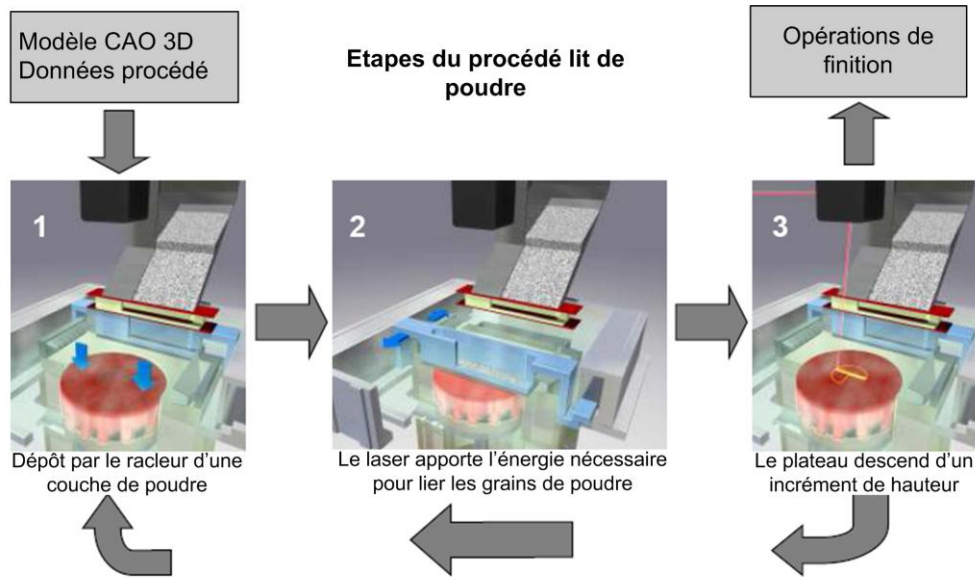
Figure 5 : Principe de la fabrication lit de poudre [NOB05]
