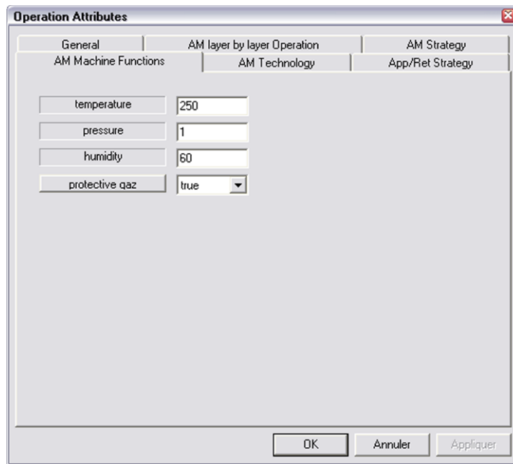
Figure 115 : Définition des paramètres de l'enceinte de fabrication dans PosSFP-AM
