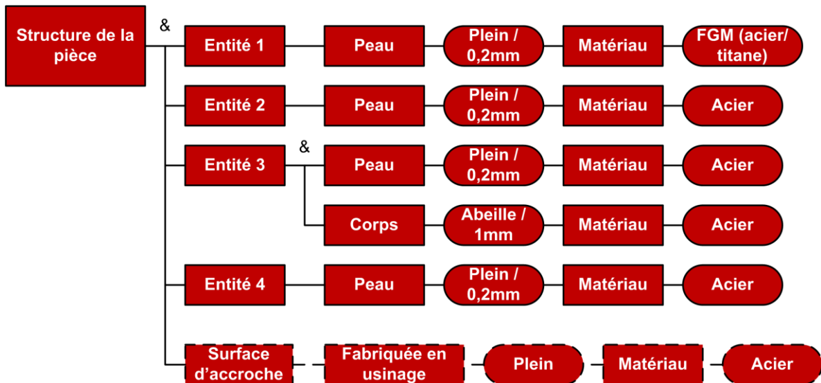
Figure 69 : Structure de la pièce-test
