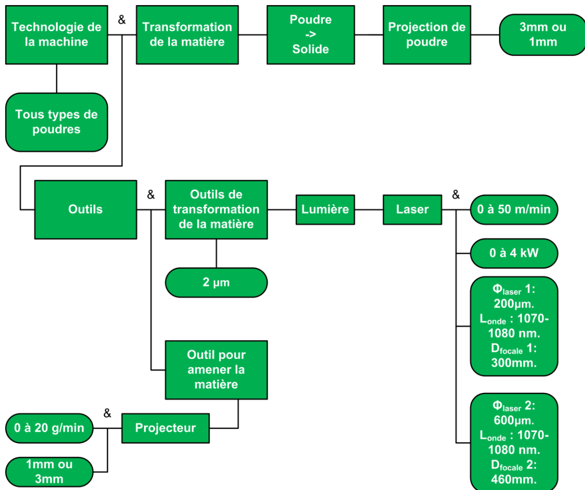
Figure 63 : Description de la technologie de fabrication additive de la machine CLAD
