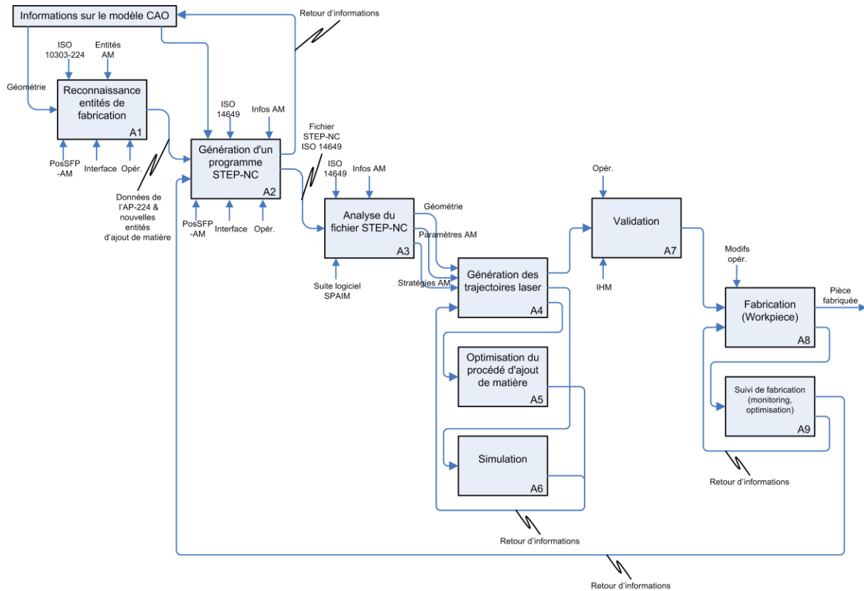
Figure 104 : Structure fonctionnelle d'une plateforme STEP-NC pour la fabrication additive
