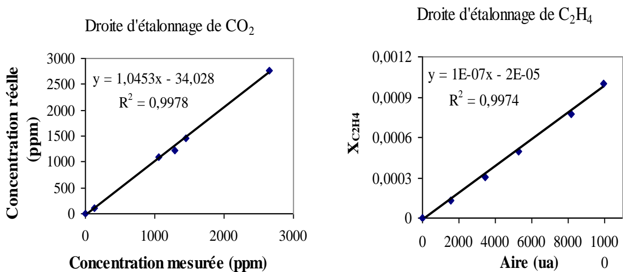
Figure III-7 Exemples de courbes d'étalonnage en IRTF ( \text{CO}_2 ) et en CPG ( \text{C}_2\text{H}_4 )
