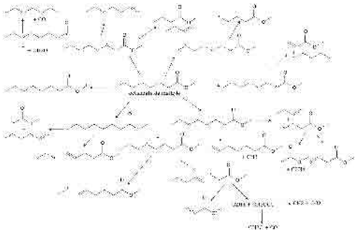
Figure V-35 : Voies de dégradations principales de l'octanoate de méthyle lors de l'oxydation d'un mélange octanoate de méthyle/oxygène/azote (P=10 atm, φ=1) en réacteur auto-agité à T=950 K
