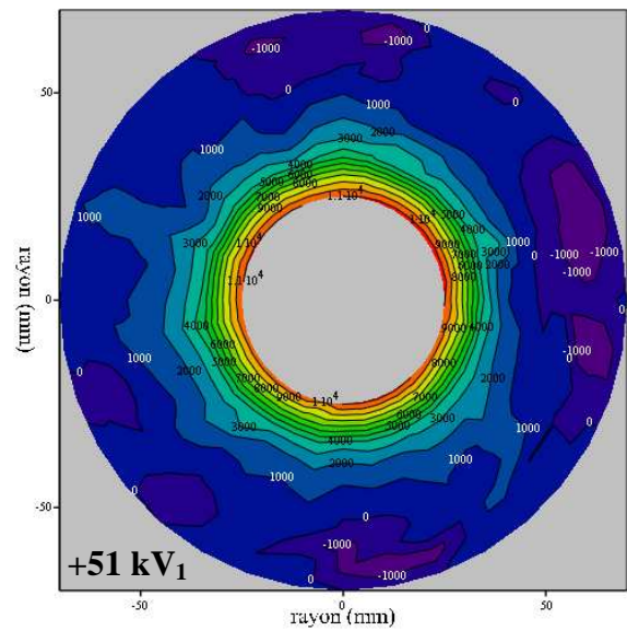
Figure 6.12. Potentiels mesurés sur la surface de l'isolant pour différentes impulsions de tension positive appliquées générant seulement des DP dans la zone du PT.
