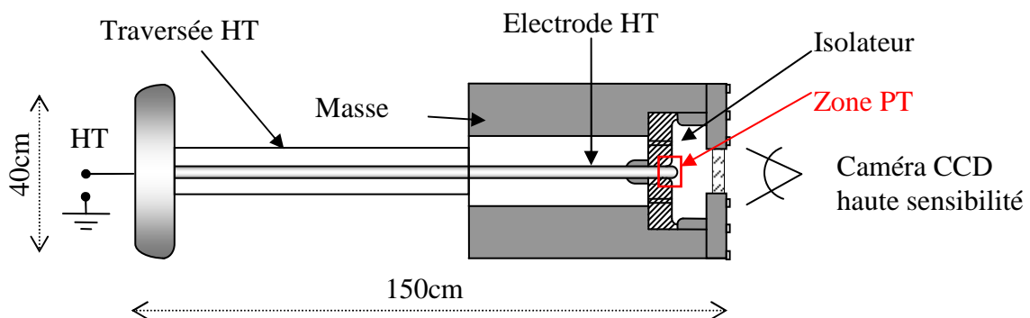
Figure 2.1. Schéma de la cellule d'essai AREVA
