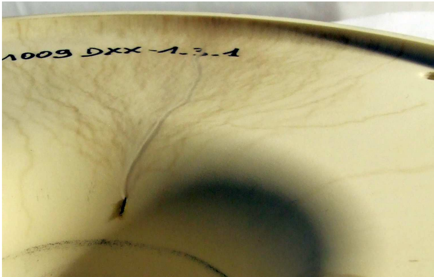
Figure 4.36. La rayure présente sur la surface de l'isolant dans le voisinage du défaut dans le PT, après plusieurs claquages
