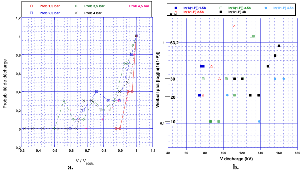
Figure 3.32. Résultats obtenus dans l'étude du point triple sous tension 0,4/1400µs :
