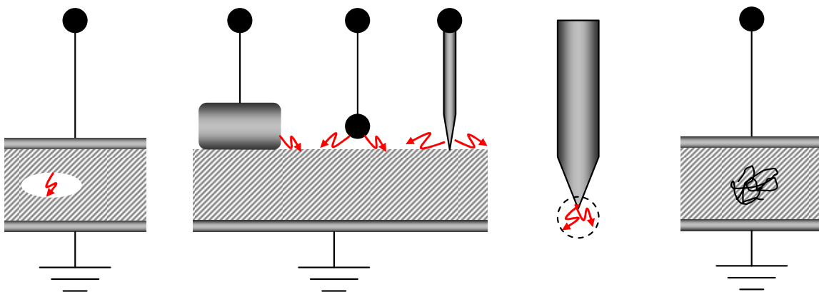
Figure 1.4. Types de décharges partielles : a) internes ; b) de surface ; c) couronne ; d) en arborescence.
