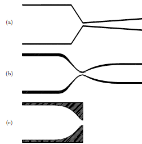
FIG. 1.4 – Trois types de tuyère étudiées par O. Hagena et al [14] : a) Tuyère conique b) Tuyère de Laval c) Tuyère sonique
