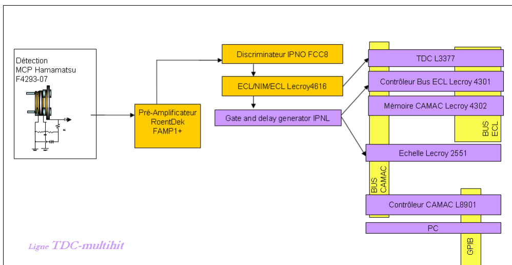
FIG. 2.3 – Chaîne d'acquisition CAMAC
