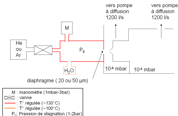
FIG. 1.6 – Schéma de la source utilisée pour former nos agrégats
