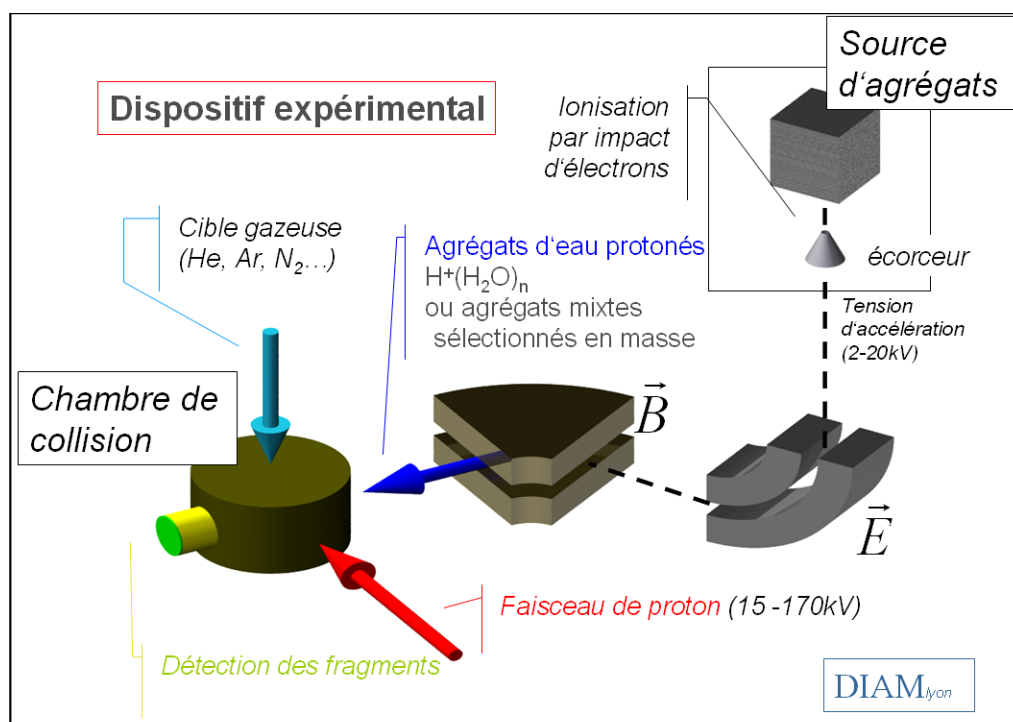
FIG. 1.1 – Dispositif expérimental DIAM
