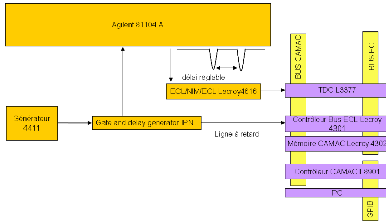
FIG. 2.6 – Schéma du système de test du TDC
