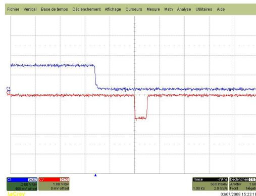
FIG. 2.5 – Mesure du temps mort du DFC : les signaux entrants étaient séparés de 34.75\text{ ns} et seul le premier signal a été discriminé
