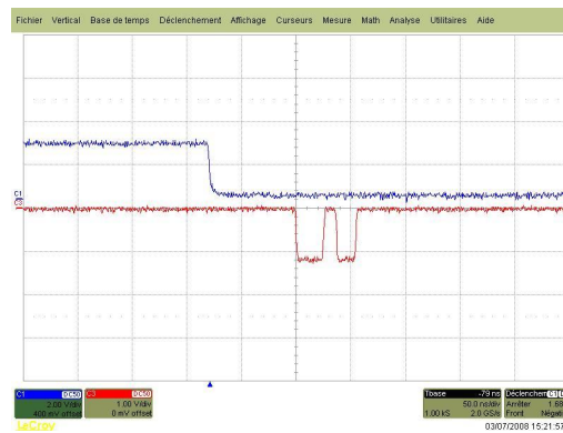
FIG. 2.4 – Mesure du temps mort du DFC : les signaux entrants étaient séparés de 34.80\text{ ns} et les deux signaux ont été discriminés
