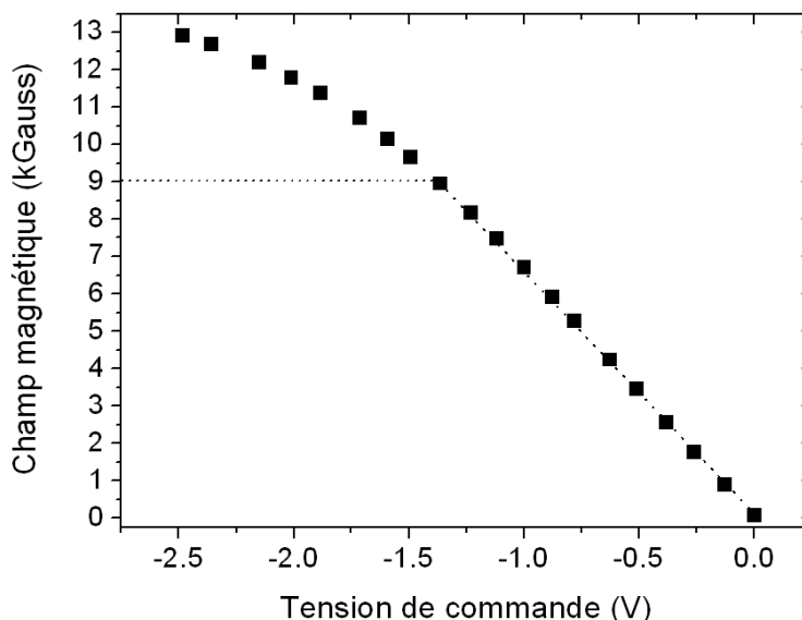
FIG. 1.32 – Champ magnétique en fonction de la tension de commande
