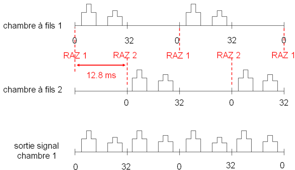
FIG. 1.20 – Schéma de principe de l'utilisation des deux modules de chambre à fils
