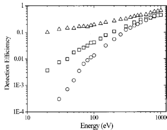
FIG. 2.36 – Efficacité de détection absolue en fonction de l'énergie d'impact pour O^+ (cercles) O^- (triangles) et O (carrés) [31]
