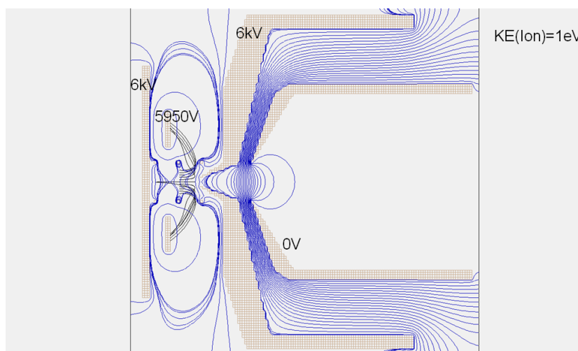
FIG. 1.11 – Simulation des trajectoires des ions lors de l'accélération de 6kV : aucun ion (d'énergie 1eV dans la direction de la détente) n'entre dans le spectromètre
