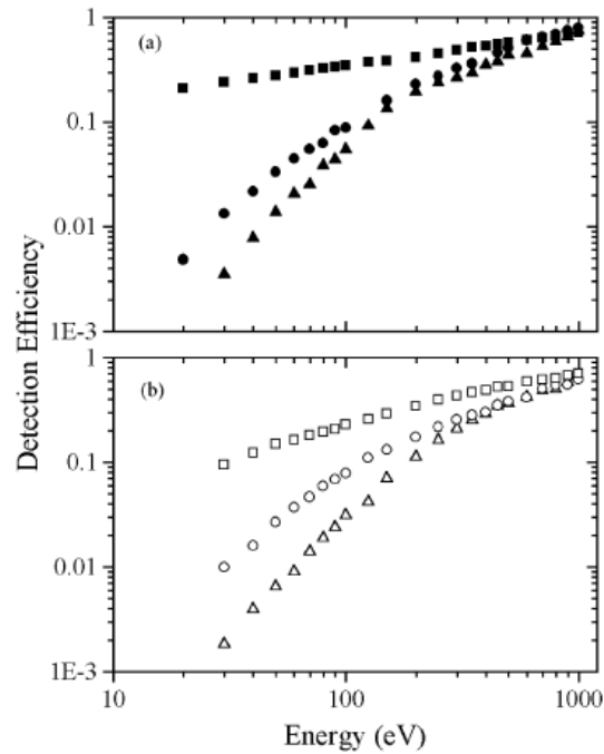
FIG. 2.35 – Efficacité de détection absolue en fonction de l'énergie d'impact pour : (a) : H^+ (cercles) H (triangles) et H^- (carrés) (b) : D^+ (cercles) D (triangles) et D^- (carrés) [30]
