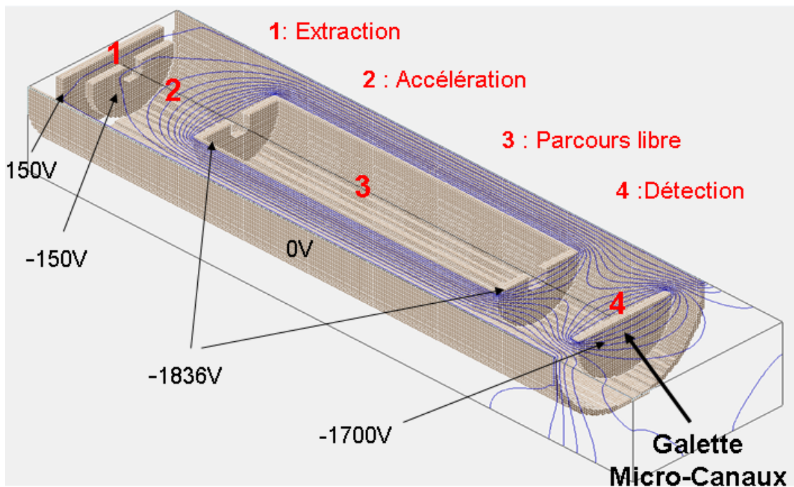
FIG. 2.24 – Géométrie du tdv utilisée avec le logiciel SIMION
