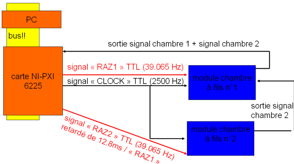
FIG. 1.19 – Schéma du système de contrôle des deux modules de chambre à fils
