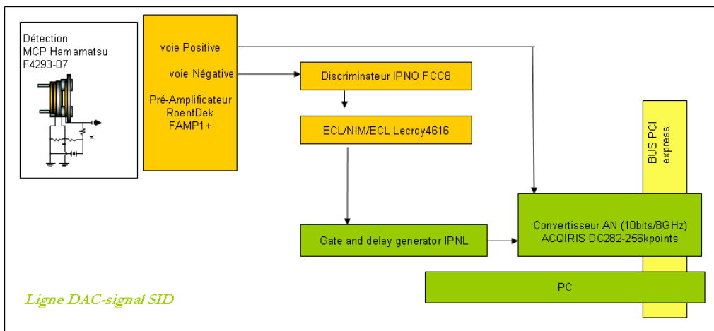
FIG. 2.12 – Chaîne d'acquisition Acqiris
