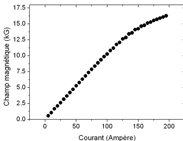
FIG. 1.22 – Champ magnétique en fonction de l'intensité
