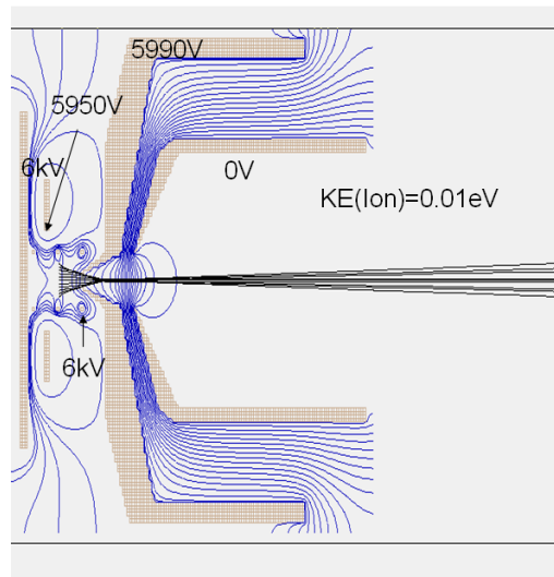
FIG. 1.12 – Simulation des trajectoires des ions lors de l'accélération de 6kV : les ions (d'énergie 0.01eV dans la direction de la détente) sont soumis à une différence de 10V. L'intégralité pénètre dans le spectromètre.
