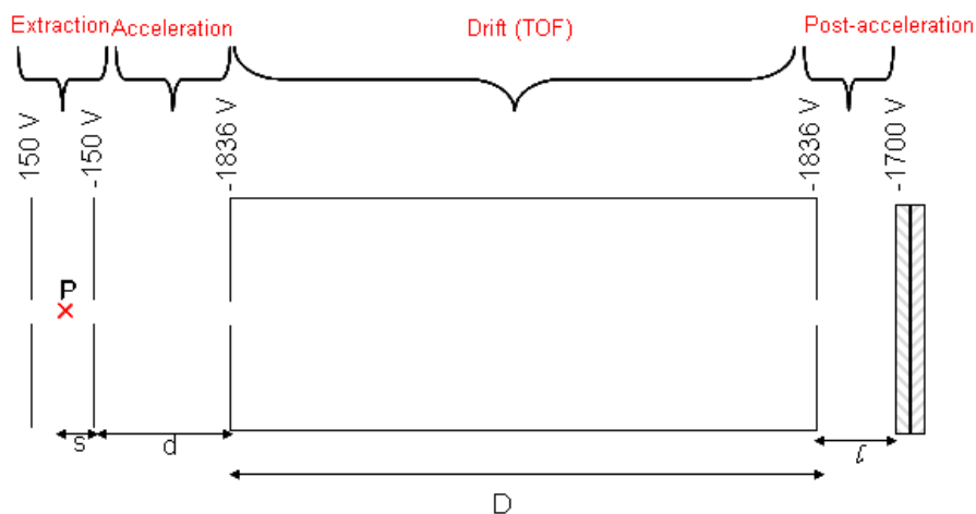
FIG. 2.22 – Schéma de notre temps de vol
