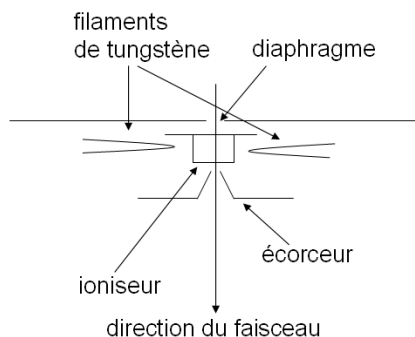
FIG. 1.8 – Vue schématique du dispositif d'ionisation
