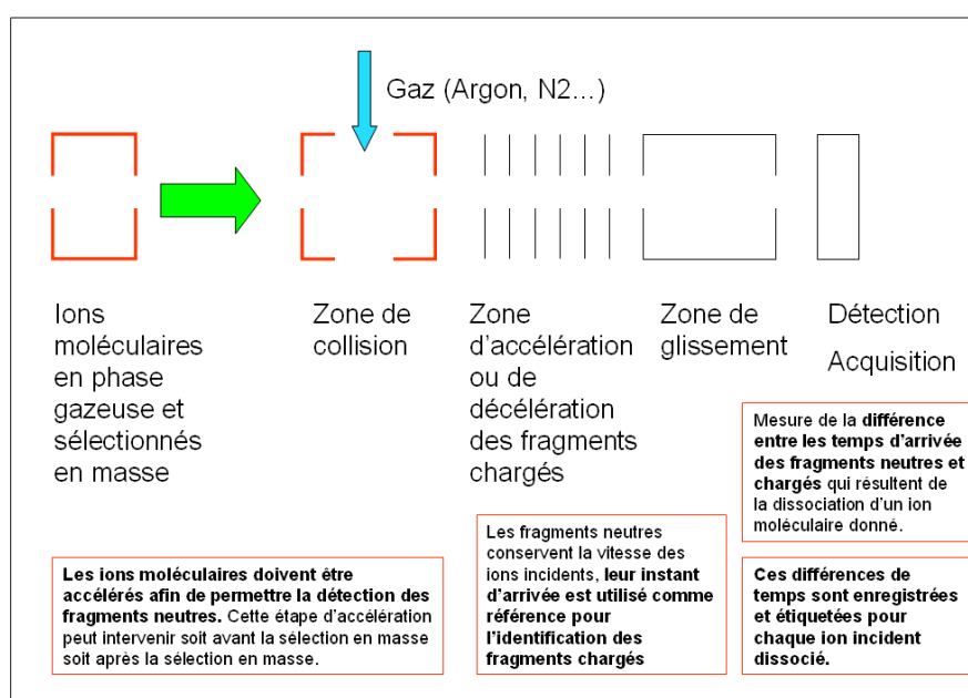
FIG. 2.1 – Principe du temps de vol sans start externe
