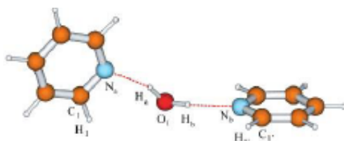
FIG. 3.56 – Géométrie optimisée du dimère de pyridine associée à une molécule d'eau, S. Schlicker et al [135]
