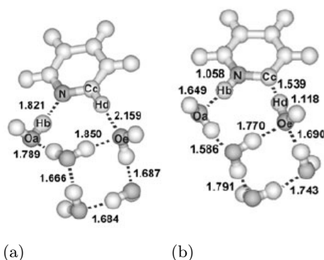
FIG. 3.51 – (a) Valeurs des distances (en angströms) les plus significatives concernant \text{Pyr}(\text{H}_2\text{O})_5 ; (b) Valeurs des distances (en angströms) les plus significatives concernant la structure obtenue pour l'agrégat \text{PyrH}^+(\text{H}_2\text{O})_5 M.C. Sicilia et al., [132])
