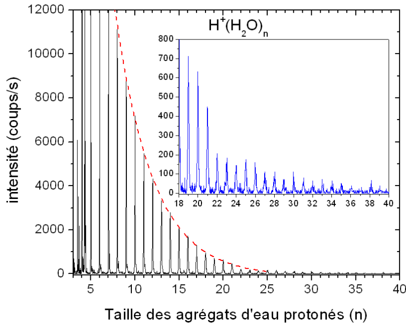
FIG. 1.25 – Spectre de masse d'agrégats d'eau protonés H^+(H_2O)_n n=3-39 . En insert, n=19 à 39. [20], (cf. tableau 1.3)
