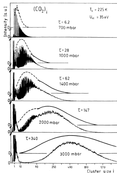
FIG. 1.5 – Évolution de la forme de la distribution d'agrégats ionisés (\text{CO}_2)_n lorsque la taille moyenne des agrégats augmente [15]. \tau représente la taille moyenne théorique des agrégats, ajustée pour correspondre aux résultats expérimentaux.
