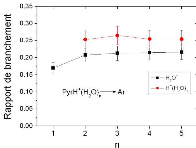
FIG. 3.47 – Rapport de branchement de H_3O^+ et H^+(H_2O)_2 comparés à celui de C_5H_5NH^+ lors de la dissociation induite par collision à 95 \times 10^3 m/s de C_5H_5NH^+(H_2O)_n n=1-5 sur une cible d'argon
