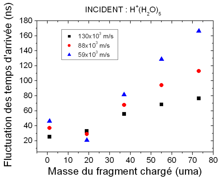
FIG. 2.25 – Dispersion des temps d'arrivée des fragments chargés dans le cas d'une dissociation induite par collision d'un agrégat incident H^+(H_2O)_5 et ce, pour trois vitesses initiales différentes
