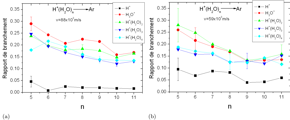
FIG. 3.20 – Rapport de branchement de production des différents fragments ioniques issus de H^+(H_2O)_n n=5-11 . (a) : v = 88 \times 10^3 m/s (b) : v = 59 \times 10^3 m/s
