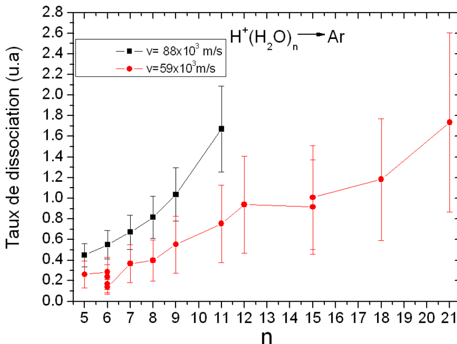
FIG. 3.25 – Taux de dissociation relatif de dissociation des agrégats H^+(H_2O)_n ( n=5-9;11 ) sur une cible d'Ar à v = 88 \times 10^3 m/s et v = 59 \times 10^3 m/s , et n=12;15;18;21 à v = 59 \times 10^3 m/s
