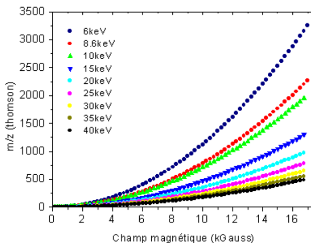
FIG. 1.23 – Masses accessibles dans le spectromètre en fonction du champ magnétique et pour une tension d'accélération donnée
