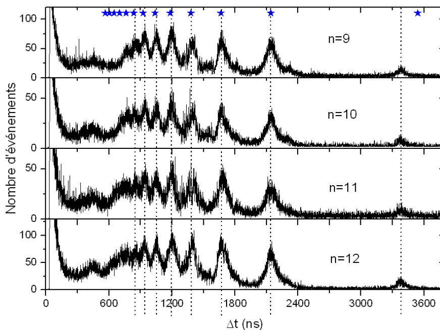
FIG. 3.11 – Spectre de fragmentation des agrégats d'eau protonés H^+(H_2O)_n , n=9-12 . La dissociation est induite par collision par croisement avec un jet d'argon. La collision se produit à une vitesse de 59 \times 10^3 m/s .
