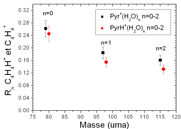
FIG. 3.43 – Rapport de branchement de production du fragment \text{C}_4\text{H}_4\text{H}^+ provenant de \text{C}_5\text{H}_5\text{NH}^+(\text{H}_2\text{O})_n ( n=0,1,2 ) et de \text{C}_4\text{H}_4^+ provenant de \text{C}_5\text{H}_5\text{N}^+(\text{H}_2\text{O})_n ( n=0,1,2 )
