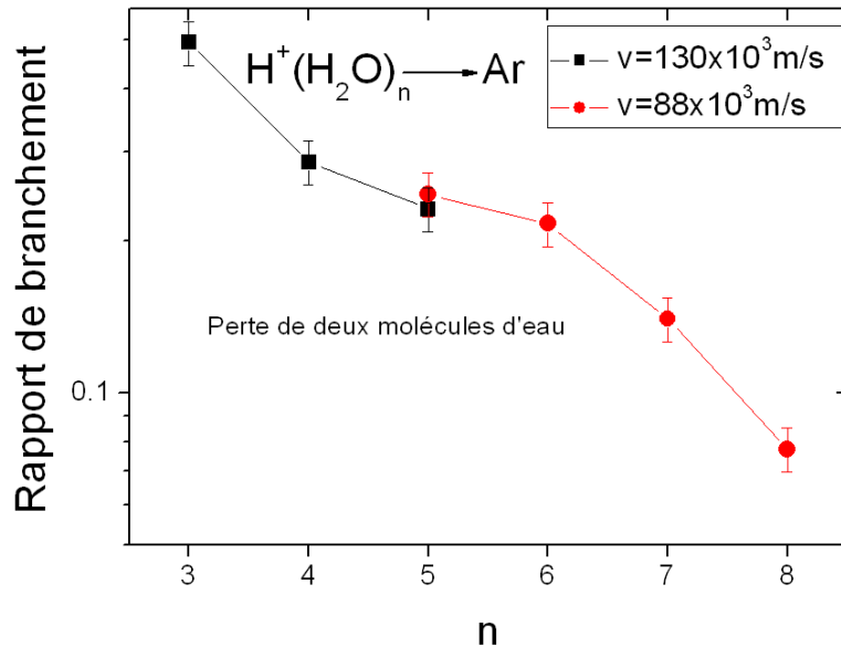
FIG. 3.15 – Rapport de branchement de perte de deux molécules d'eau lors de CID sur H^+(H_2O)_n n=3-5 à v = 130 \times 10^3 m/s et n=5-8 à v = 88 \times 10^3 m/s .
