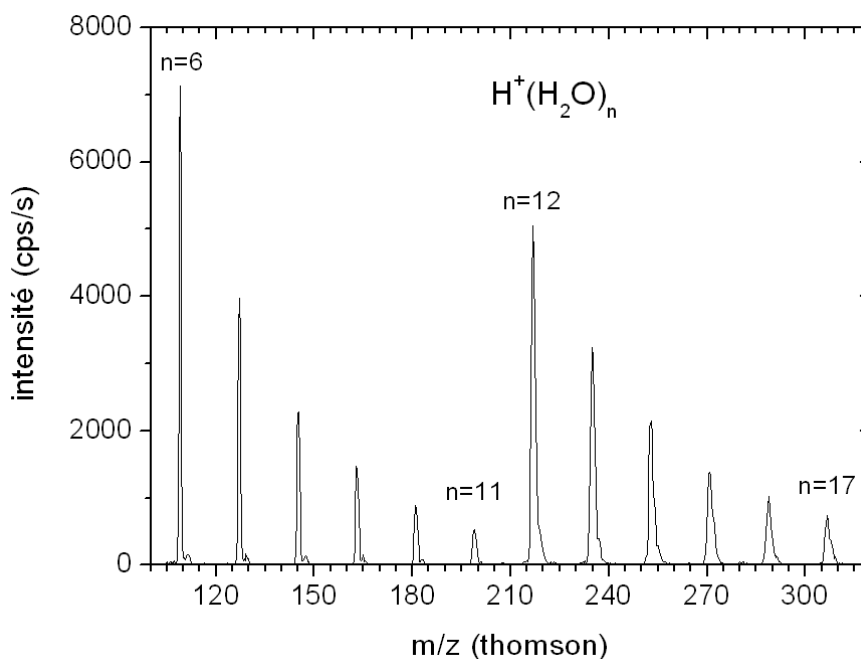
FIG. 1.24 – Spectre de masse d'agrégats d'eau protonés H^+(H_2O)_n n=6-17 . La vanne d'ajout de gaz porteur (2bar He) a été ouverte puis refermée entre n=11 et n=12 (cf. tableau 1.2)
