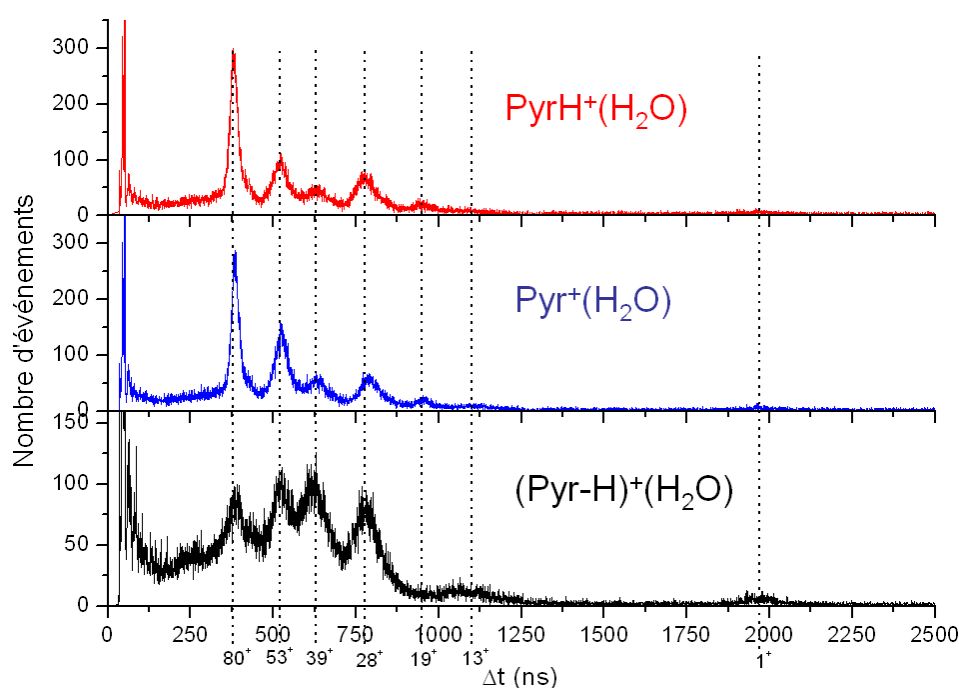
FIG. 3.38 – Spectres issus de CID sur trois types de pyridine ionisée ( PyrH^+ , Pyr^+ et (Pyr - H)^+ ) chacune associée à une molécule d'eau
