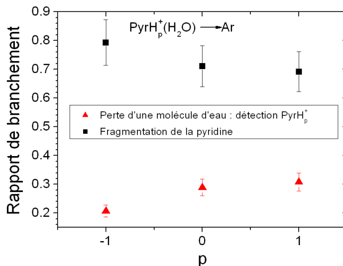
FIG. 3.40 – Rapport de branchement de PyrH_p^+ ( p = -1, 0, 1 ) et de l'ensemble des autres voies de dissociation mesurées lors de CID sur PyrH_p^+(H_2O) ( p = -1, 0, 1 ) à 95 \times 10^3 m/s
