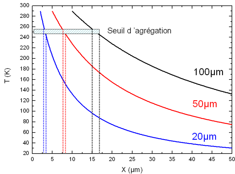
FIG. 1.10 – Température en fonction de la distance à l'endroit de la détente, pour différentes tailles de diaphragme. Le seuil de nucléation est issu de [16] et le modèle pour les courbes de décroissance de température de [17].
