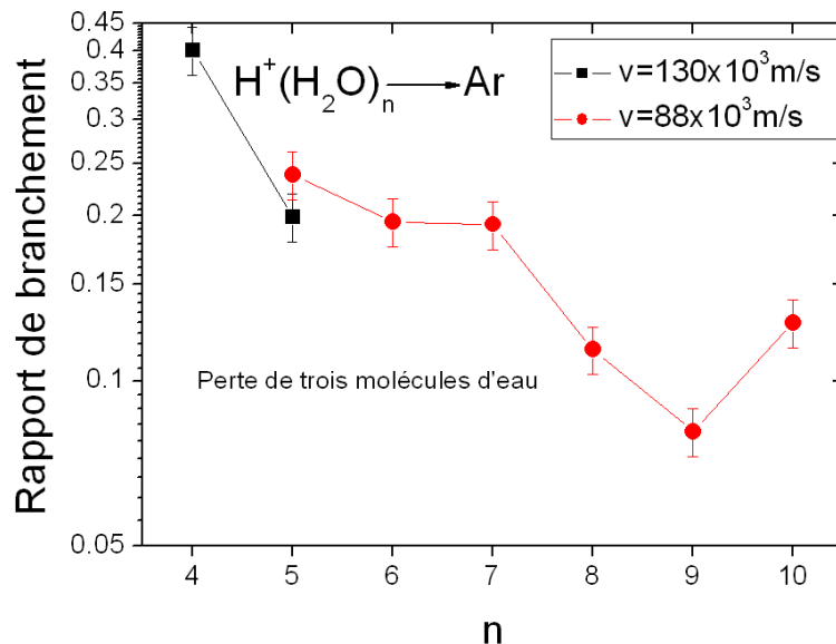
FIG. 3.16 – Rapport de branchement de perte de trois molécules d'eau lors de CID sur H^+(H_2O)_n n=4-5 à v = 130 \times 10^3 m/s et n=5-10 à v = 88 \times 10^3 m/s .
