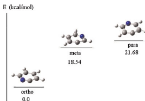
FIG. 3.42 – Energie des différents isomères de pyridine déshydrogénée ionisée, S. Yao et al [118]
