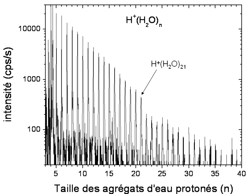
FIG. 3.1 – Spectre de masses d'agrégats H^+(H_2O)_n [20]
