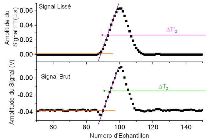
FIG. 2.20 – Détermination des temps d'arrivée pour les signaux bruts et les signaux filtrés : en haut signal traité par TF, en bas signal brut. Pour chaque signal, le temps est déterminé par la méthode du piedestal. La différence de temps entre les deux signaux présents dans l'événement est ensuite calculée. Seul le premier pic de l'événement est présenté.
