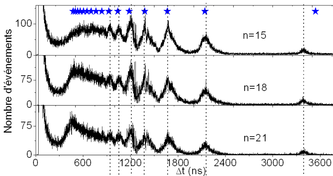
FIG. 3.12 – Spectre de fragmentation des agrégats d'eau protonés H^+(H_2O)_n , n=15;18;21 . La dissociation est induite par collision par croisement avec un jet d'argon. La collision se produit à une vitesse de 59 \times 10^3 m/s .
