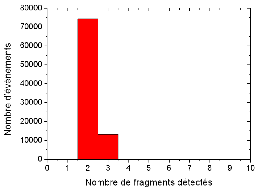
FIG. 3.6 – Distribution des événements de dissociation en fonction du nombre de fragments détectés pour un lot de 87283 dissociations d'agrégats H^+(H_2O)_3 (8keV-Ar) associés à la détection du fragment H^+(H_2O)
