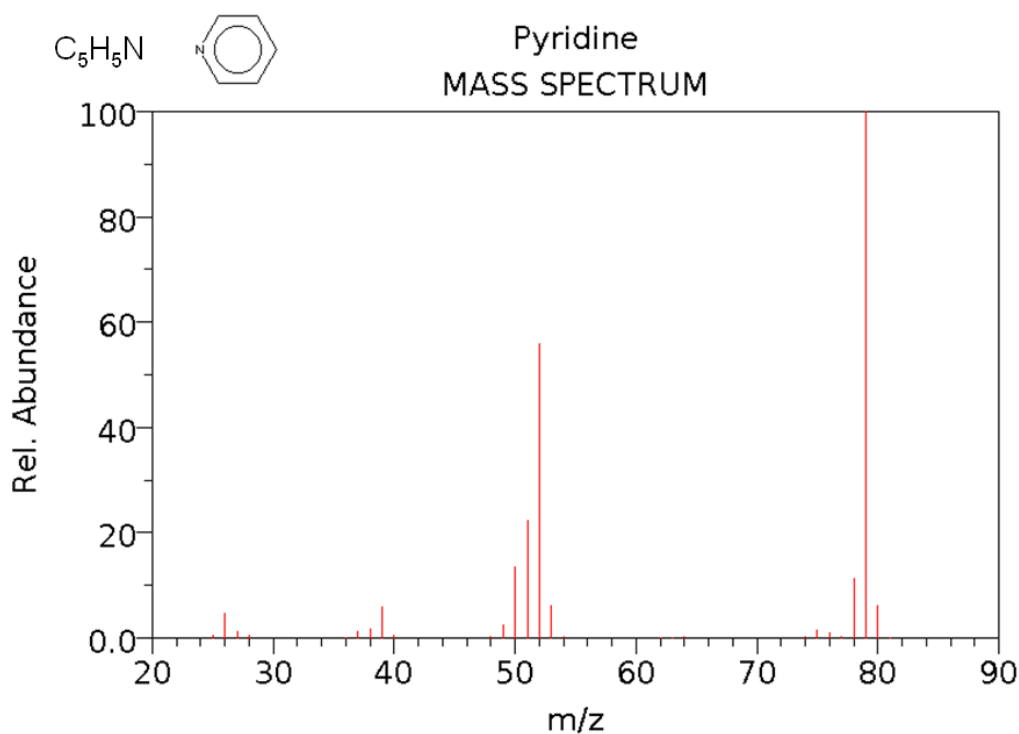
FIG. 3.26 – Spectre de masse de la pyridine obtenu par impact d'électrons [22]
