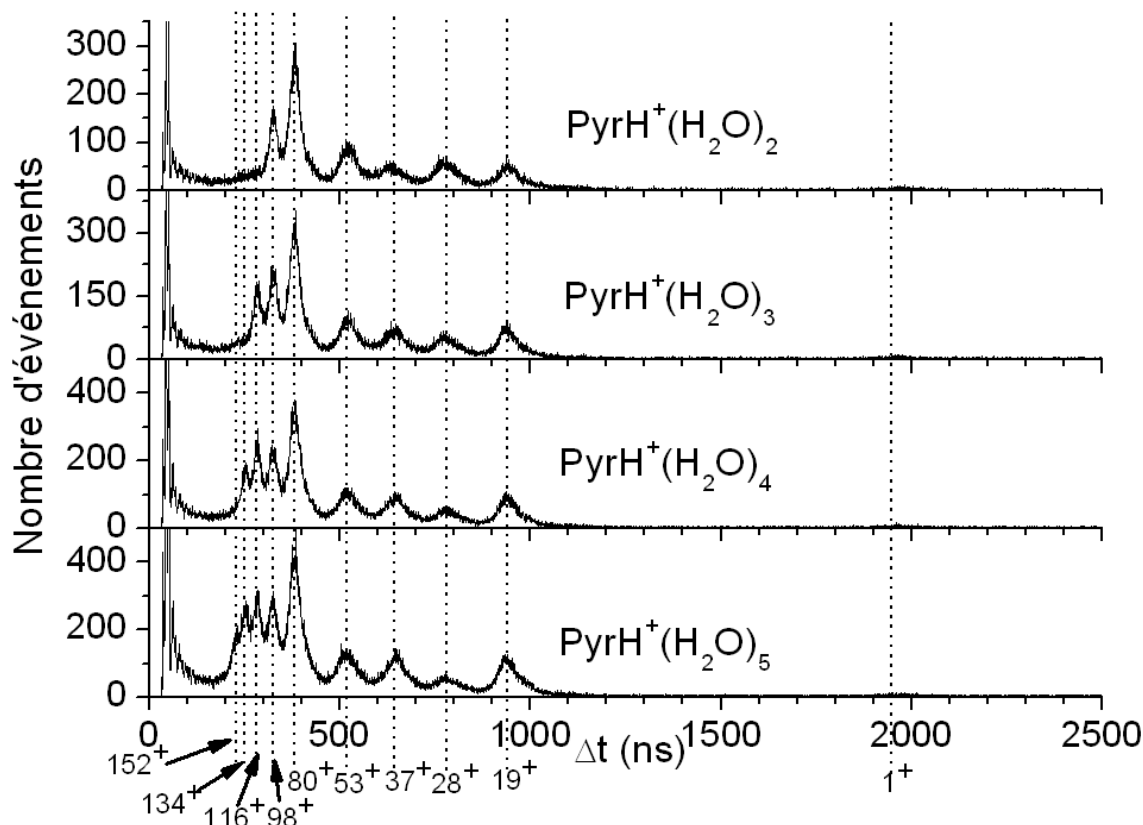
FIG. 3.46 – Spectre de fragmentation des agrégats protonés mixtes PyrH^+(H_2O)_n , n=2-5
