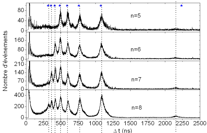
FIG. 3.8 – Spectre de fragmentation des agrégats d'eau protonés H^+(H_2O)_n , n=5-8 . La dissociation est induite par collision par croisement avec un jet d'argon. La collision se produit à une vitesse de 88 \times 10^3 m/s . Les étoiles correspondent aux différences de temps, calculées par SIMION, associées aux pertes d'une, deux, trois, ... n molécules d'eau de la part de l'agrégat incident.
