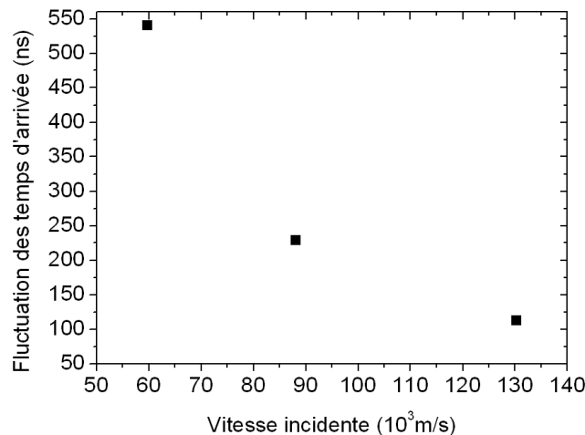
FIG. 2.26 – Dispersion des temps d'arrivée des fragments neutres dans le cas d'une dissociation induite par collision d'un agrégat incident H^+(H_2O)_5 et ce, pour trois vitesses initiales différentes
