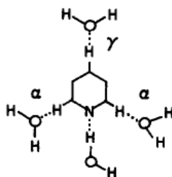
FIG. 3.49 – Complexe pyridine-eau. Trois points signifient une liaison hydrogène, M.R. Zakin et al. [131]
