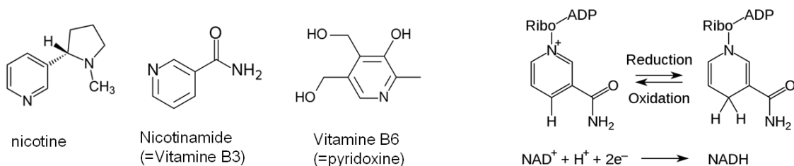
FIG. 1.27 – Molécules d'intérêt biologique constitué de pyridine
