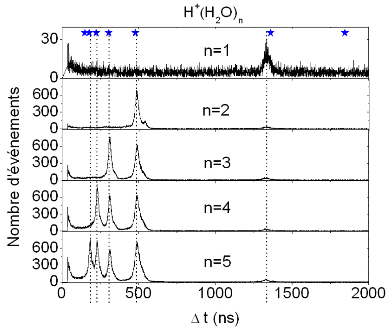
FIG. 2.2 – Spectres de temps de vol des fragments issus de la dissociation induite par collision de l'agrégat H^+(H_2O)_n ( n=1-5 ), à une vitesse initiale de 130 \times 10^3 \text{ m/s}
