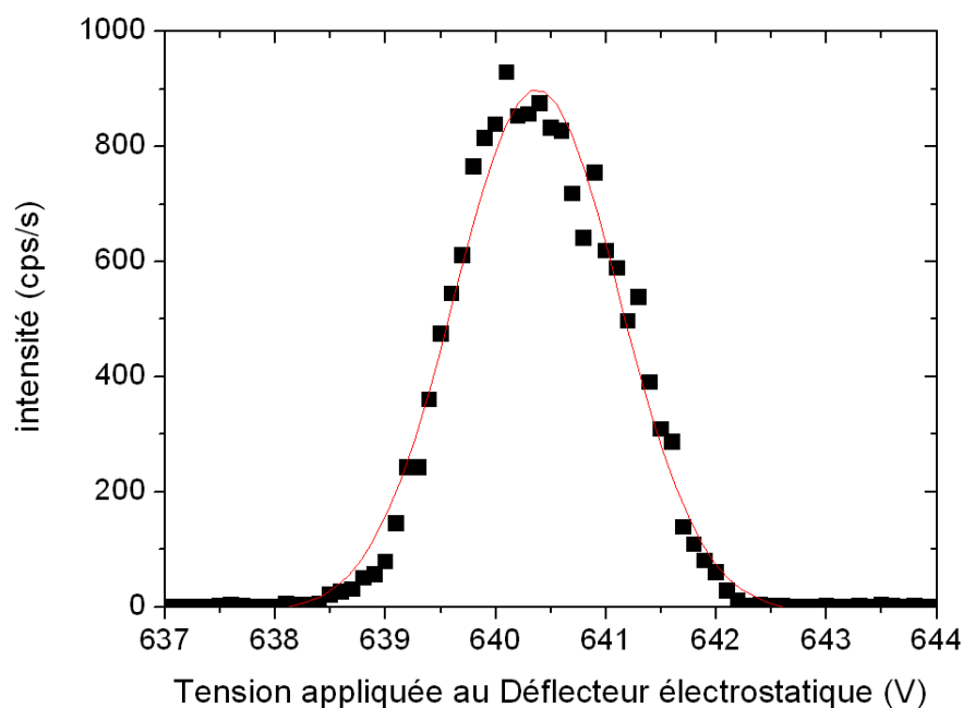
FIG. 1.33 – Distribution en énergie des agrégats : Intensité du signal en fonction de la tension aux bornes du déflecteur électrostatique
