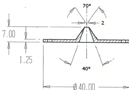
FIG. 1.7 – Schéma de l'écorceur utilisé dans le dispositif
