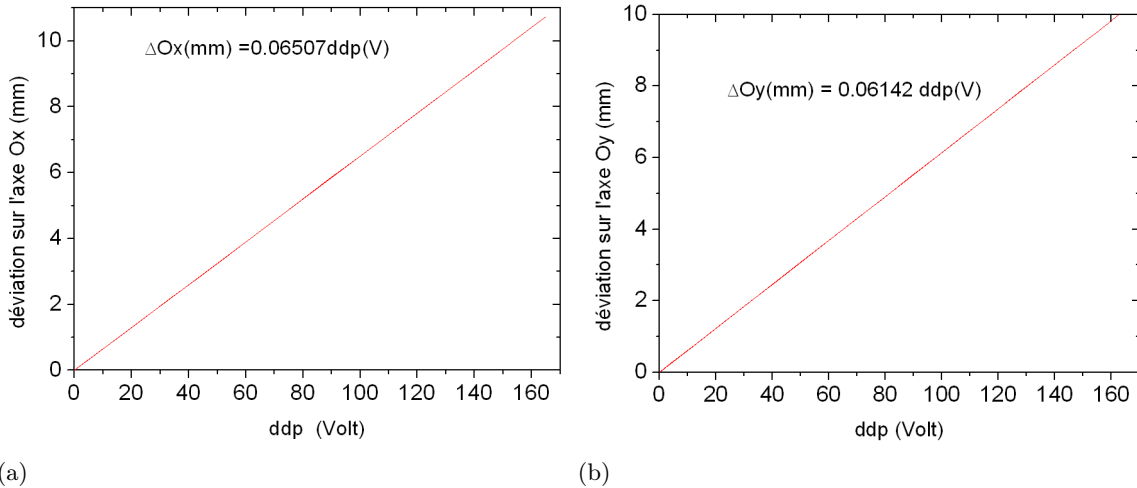
FIG. 1.18 – Déviation (en mm) à l'entrée du déflecteur d'une molécule d'eau ( m/z=18 ) accélérée à 6kV sous l'effet de l'application d'une tension sur une seule paire de steerers Ox (a) et Oy (b)
