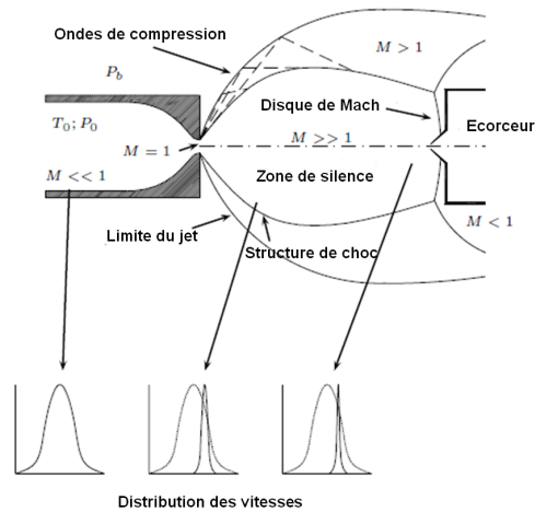
FIG. 1.9 – Structure et caractéristiques du jet supersonique
