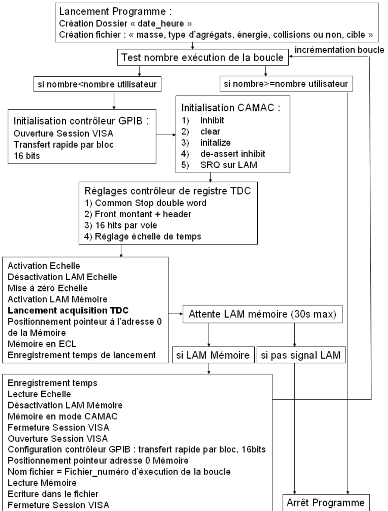
FIG. 2.9 – Organigramme du programme d'acquisition CAMAC
