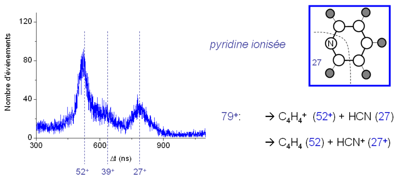
FIG. 3.34 – Pics principaux du spectre de fragmentation de Pyr^+
