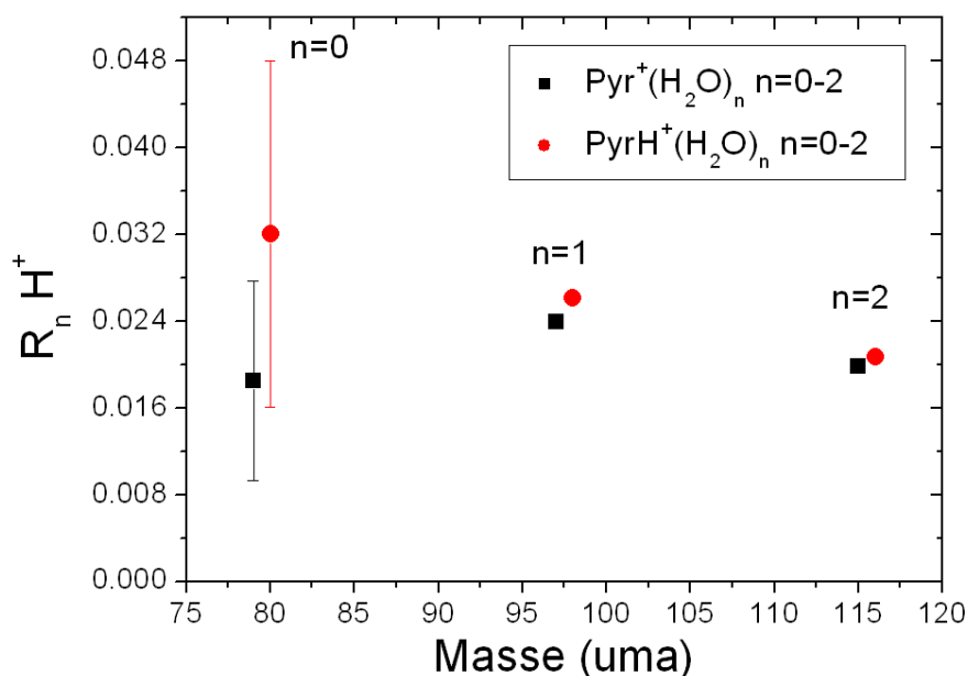
FIG. 3.52 – Rapport de branchement de \text{H}^+ issu de la dissociation de \text{PyrH}^+(\text{H}_2\text{O})_n et \text{Pyr}^+(\text{H}_2\text{O})_n ( n=0-2 )
