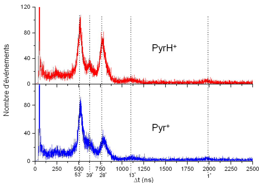
FIG. 3.33 – Spectre résultant de CID sur la pyridine protonée PyrH^+ et sur la pyridine ionisée Pyr^+ , accélérées à 95 \times 10^3 m/s
