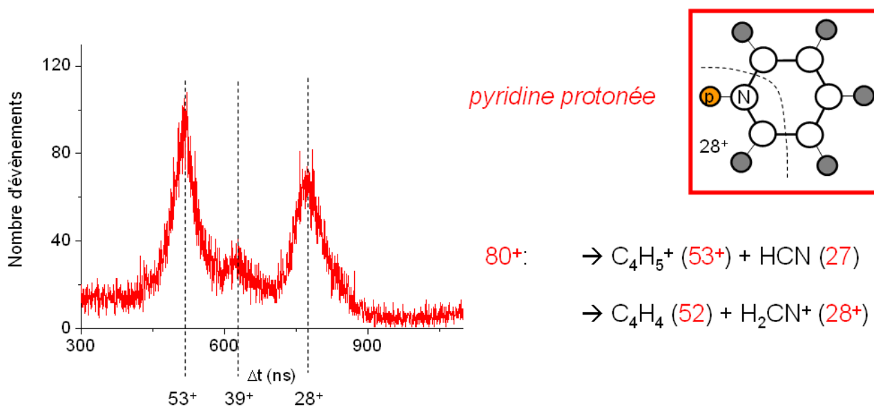
FIG. 3.36 – Pics principaux du spectre de fragmentation de \text{PyrH}^+
