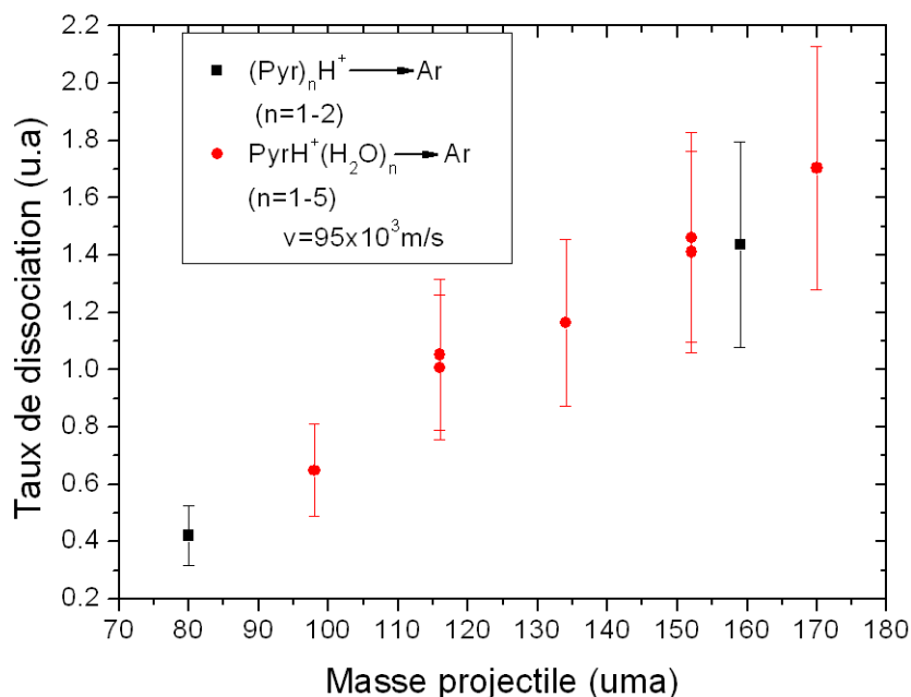
FIG. 3.55 – Taux de dissociation relatif des agrégats \text{PyrH}^+(\text{H}_2\text{O})_n ( n=0-5 ) ainsi que de (\text{Pyr})_2\text{H}^+ . Le taux de dissociation de \text{H}^+(\text{H}_2\text{O})_5 constitue le taux de référence.
