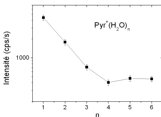
FIG. 3.31 – Intensité d'agrégats mixtes \text{Pyr}^+(\text{H}_2\text{O})_n en fonction de la taille
