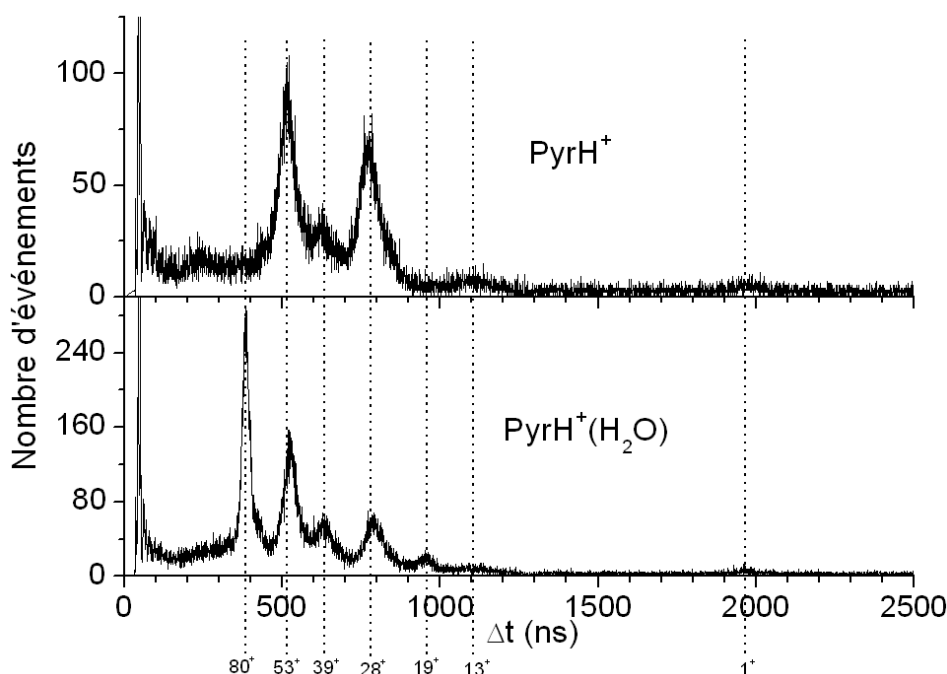
FIG. 3.45 – Spectre de fragmentation des agrégats protonés mixtes PyrH^+(H_2O)_n , n=0-1
