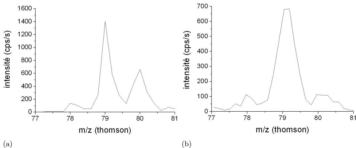
FIG. 3.27 – (a) Spectre de masse : pyridine déshydrogénée (78), pyridine ionisée (79), pyridine protonée (80) (b) idem, la pression partielle de pyridine étant inférieure
