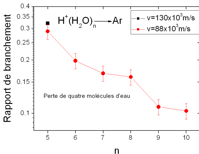
FIG. 3.17 – Rapport de branchement de perte de trois molécules d'eau lors de CID sur H^+(H_2O)_n n=4-5 à v = 130 \times 10^3 m/s et n=5-10 à v = 88 \times 10^3 m/s .
