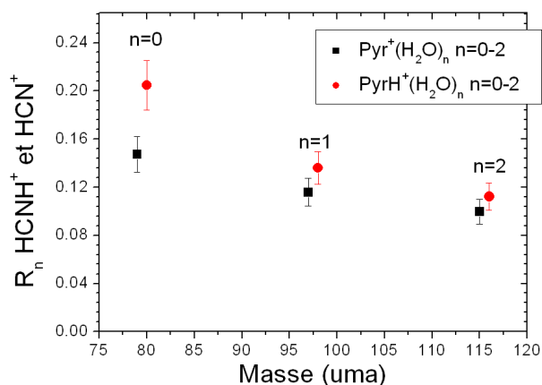
FIG. 3.44 – Rapport de branchement de production du fragment \text{HCNH}^+ provenant de \text{C}_5\text{H}_5\text{NH}^+(\text{H}_2\text{O})_n ( n=0,1,2 ) et de \text{HCN}^+ provenant de \text{C}_5\text{H}_5\text{N}^+(\text{H}_2\text{O})_n ( n=0,1,2 )
