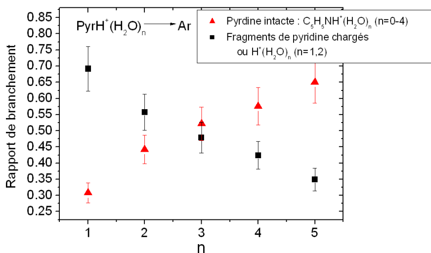
FIG. 3.53 – Comparaison entre le rapport de branchement de C_5H_5NH^+(H_2O)_n ( n=0-4 ) et des autres rapports obtenus lors de collision sur les agrégats C_5H_5NH^+(H_2O)_n ( n=1-5 )
