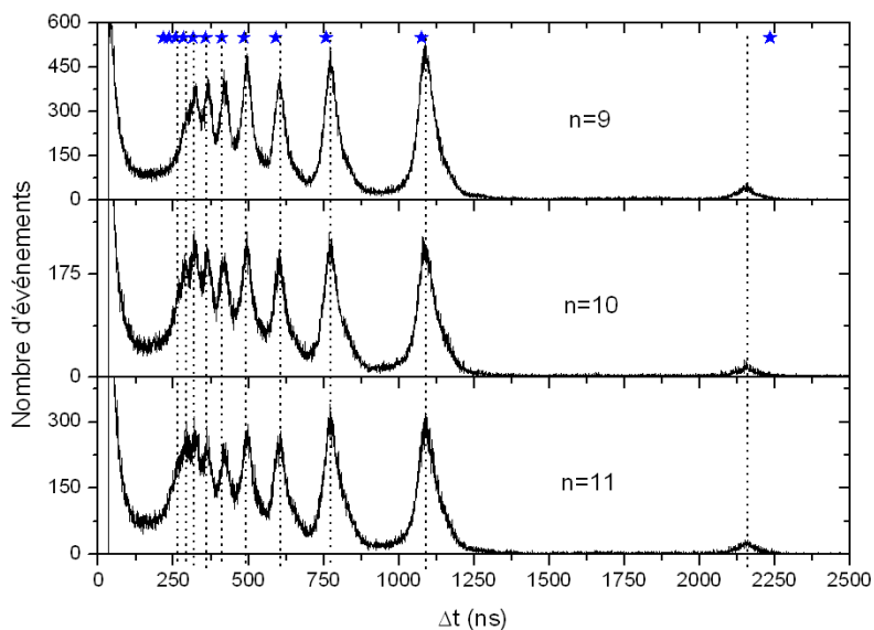
FIG. 3.9 – Spectre de fragmentation des agrégats d'eau protonés H^+(H_2O)_n , n=9-11 . La dissociation est induite par collision par croisement avec un jet d'argon. La collision se produit à une vitesse de 88 \times 10^3 m/s .
