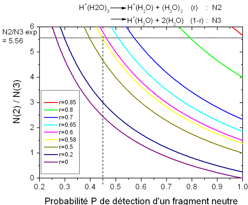
FIG. 3.7 – Évolution, en fonction de la probabilité de détection d'un fragment neutre et pour un taux donné de non-dissociation du dimère d'eau produit lors de la dissociation de H^+(H_2O)_3 , du rapport mesuré N(2)/N(3)
