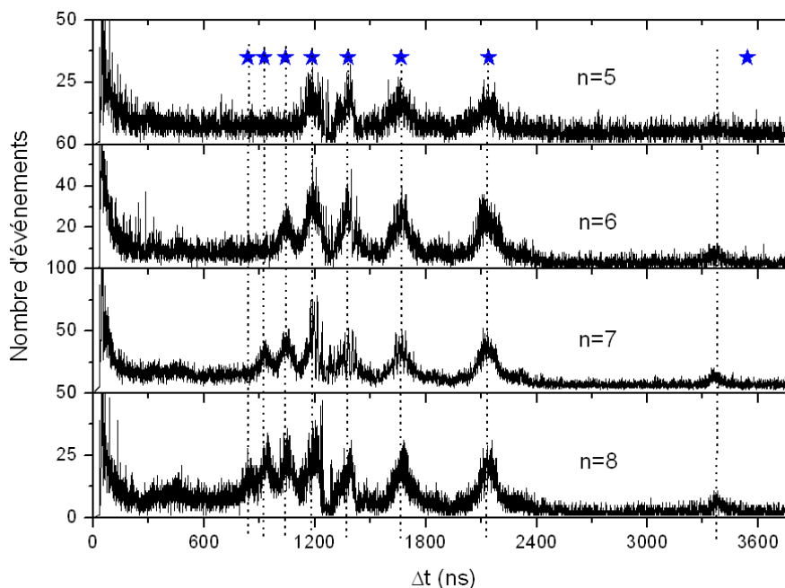
FIG. 3.10 – Spectre de fragmentation des agrégats d'eau protonés H^+(H_2O)_n , n=5-8 . La dissociation est induite par collision par croisement avec un jet d'argon. La collision se produit à une vitesse de 59 \times 10^3 m/s .
