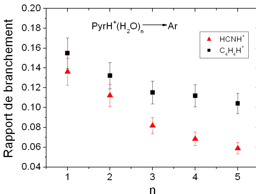
FIG. 3.50 – Rapport de branchement de H_2CN^+ (masse 28) et C_4H_4H^+ (masse 53) pour les agrégats PyrH^+(H_2O)_n ( n=0-5 )
