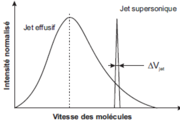
FIG. 1.2 – Distribution de vitesse suivant l'axe de la tuyère pour un jet effusif et un jet supersonique [11]
