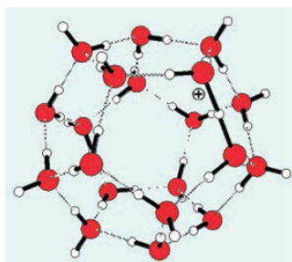
FIG. 3.2 – Forme clathrate de l'agrégat H^+(H_2O)_{21} [57]
