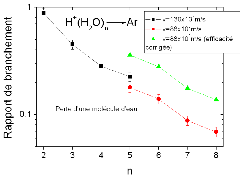
FIG. 3.14 – Rapport de branchement de perte d'une molécule d'eau lors de CID sur H^+(H_2O)_n n=2-5 à v = 130 \times 10^3 \text{ m/s} et n=5-8 à v = 88 \times 10^3 \text{ m/s} . L'efficacité concernant la vitesse de 88 \times 10^3 \text{ m/s} corrigée selon les valeurs déterminées à partir de Peko et Stephen [30] est également prise en compte.
