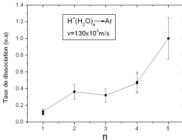
FIG. 3.24 – Taux de dissociation relatif des agrégats H^+(H_2O)_n ( n=1-5 ) sur une cible d'Ar à v = 130 \times 10^3 m/s
