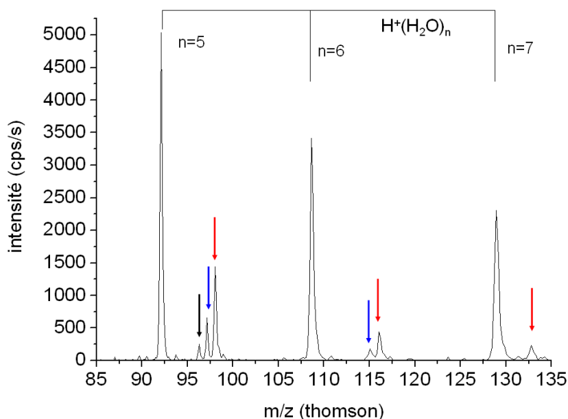
FIG. 3.29 – Spectre de masse d'agrégats d'eau et d'agrégats mixtes pyridine-eau. Les pics les plus intenses sont associés aux agrégats d'eau protonés H^+(H_2O)_n ( n=5,6,7 ). Les flèches rouges sont associées aux agrégats mixtes comportant une pyridine protonée C_5H_5NH^+(H_2O)_n ( n=1,2,3 ). Les flèches bleues sont associées aux agrégats mixtes contenant une pyridine ionisée C_5H_5N^+(H_2O)_n ( n=1,2 ). La flèche noire est associée à l'agrégat mixte contenant une pyridine déshydrogénée C_5H_4N^+H_2O
