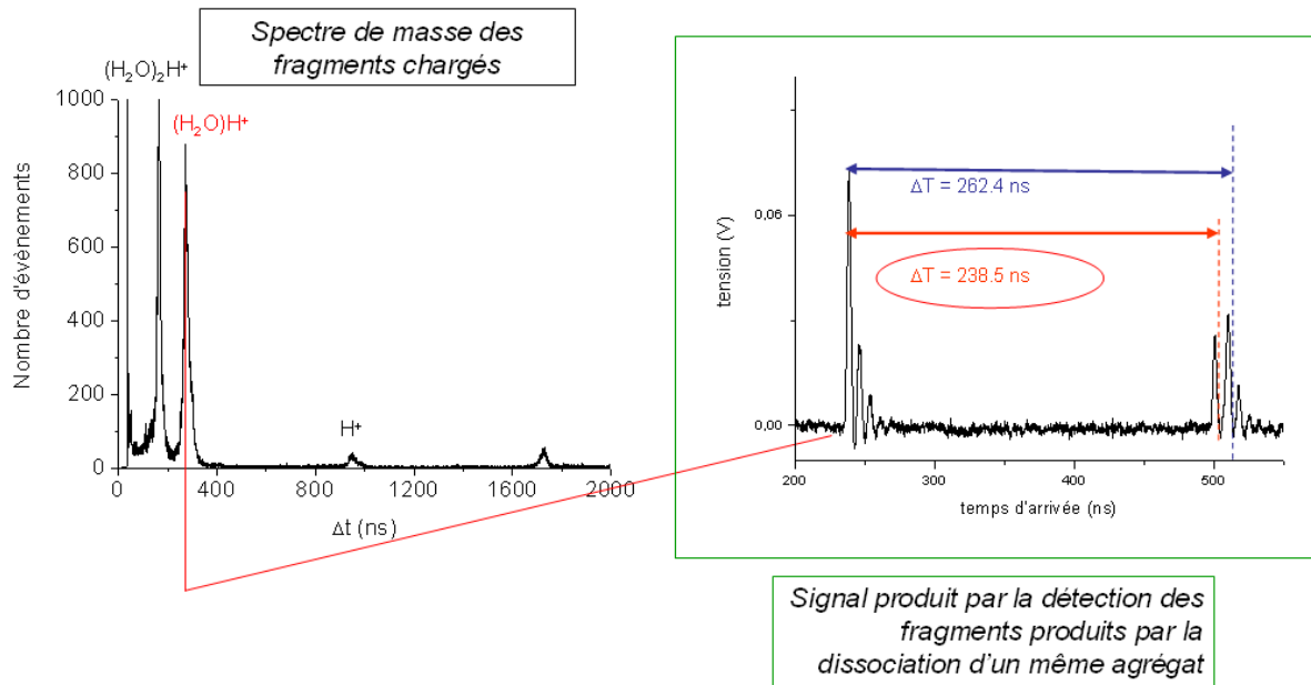
FIG. 3.4 – Spectre de fragmentation de H^+(H_2O)_3 à 8 keV sur une cible d'Ar.
