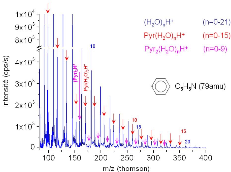
FIG. 1.29 – Spectre de masse d'agrégats d'eau protonés \text{H}^+(\text{H}_2\text{O})_n et d'agrégats mixtes protonés eau-pyridine
