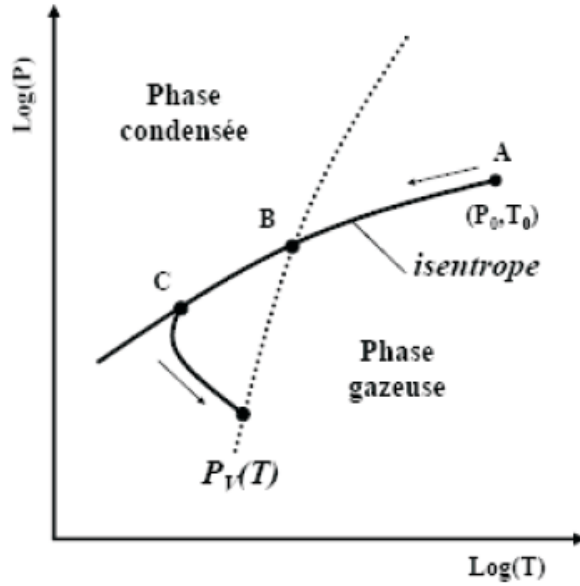
FIG. 1.3 – Diagramme de phase expliquant la formation des agrégats d'eau [13]
