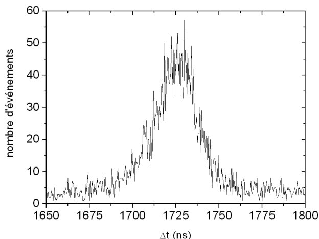
FIG. 2.32 – Pic de temps de vol associé au processus de capture électronique entre un atome d'Ar de la cible et l'agrégat incident H^+(H_2O)_3 ( v=167 \times 10^3 m/s )
