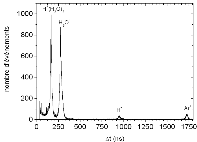
FIG. 2.31 – Spectre de temps de vol des fragments issus de la dissociation induite par collision de l'agrégat H^+(H_2O)_3 à une vitesse initiale de 167 \times 10^3 \text{ m/s} sur une cible d'Ar
