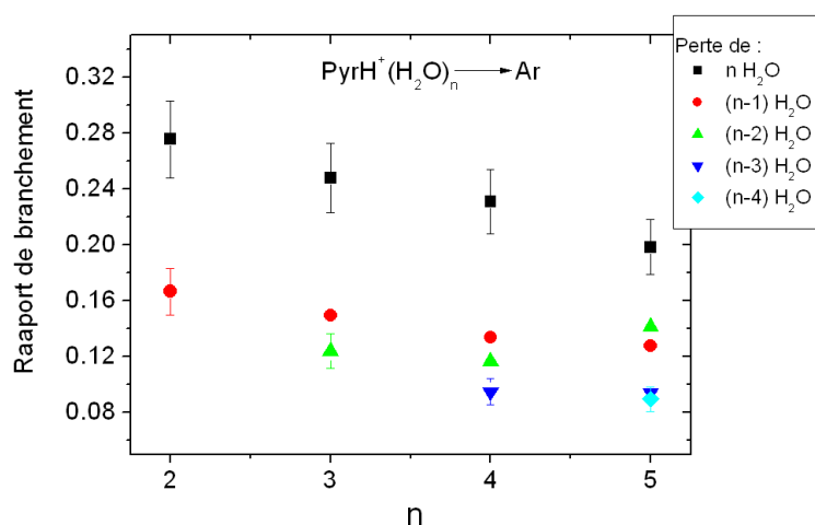
FIG. 3.48 – Rapport de branchement de perte de n molécules d'eau lors de la dissociation induite par collision d'agrégats mixtes \text{PyrH}^+(\text{H}_2\text{O})_n ( n=2-5 )
