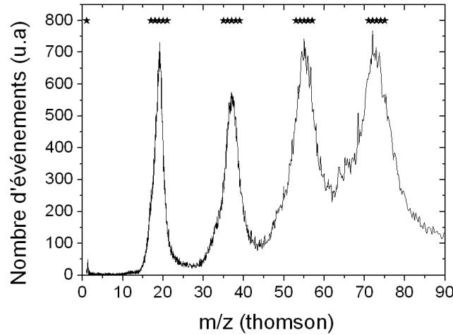
FIG. 2.34 – Spectre de temps de vol des fragments issus de la dissociation de H^+(H_2O)_5 lors d'une collision sur une cible d'Ar à une vitesse initiale de 130 \times 10^3 m/s. Chaque étoile est associée à une unité de masse.
