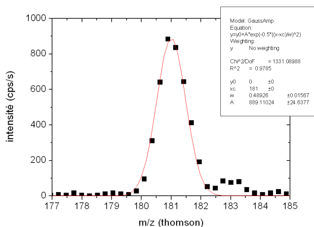
FIG. 1.30 – Intensité de l'agrégat H^+(H_2O)_{10} . La courbe d'ajustement est une gaussienne, de largeur à mi-hauteur proche de 1 m/z .
