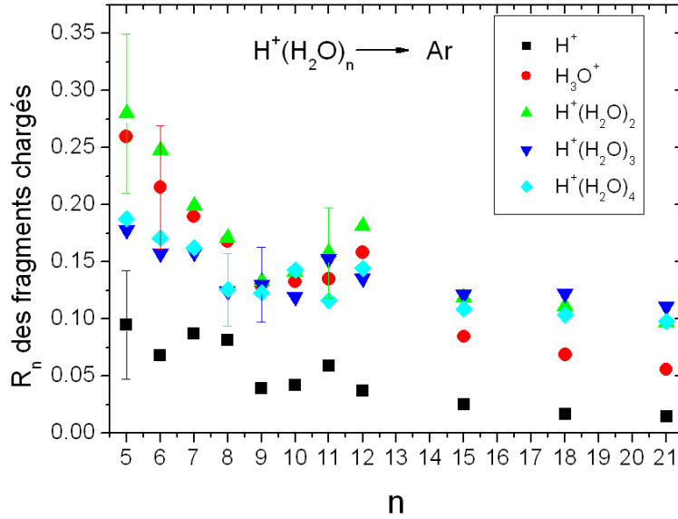
FIG. 3.23 – Rapport de branchement de production des différents fragments ioniques issus de H^+(H_2O)_n n=5-12;15;18;21 . v = 59 \times 10^3 m/s
