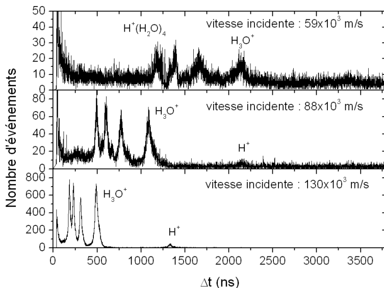
FIG. 2.30 – Spectres de temps de vol des fragments issus de la dissociation induite par collision de l'agrégat H^+(H_2O)_5 pour trois vitesses initiales
