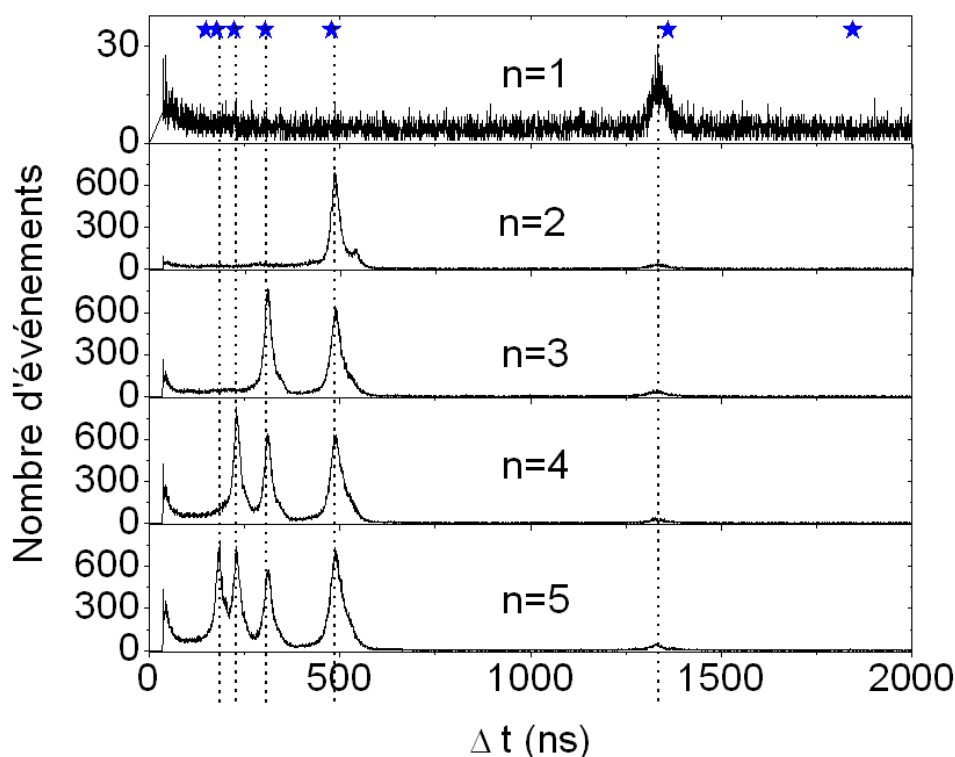
FIG. 3.13 – Spectre de fragmentation des agrégats d'eau protonés H^+(H_2O)_n n=1-5 . La dissociation est induite par collision par croisement avec un jet d'argon. La collision se produit à une vitesse de 130 \times 10^3 m/s . L'étoile la plus à droite correspond au processus de capture électronique par un agrégat incident sur un atome de la cible.
