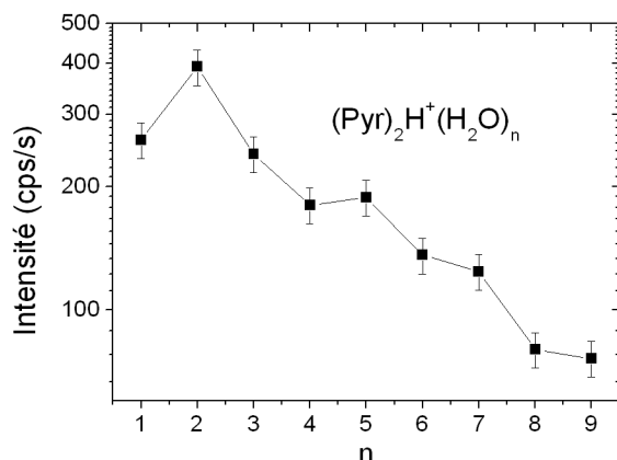
FIG. 3.32 – Intensité d'agrégats mixtes (\text{Pyr})_2\text{H}^+(\text{H}_2\text{O})_n en fonction de la taille
