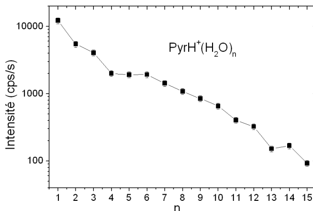
FIG. 3.30 – Intensité des agrégats de pyridine protonée et d'eau PyrH^+(H_2O)_n en fonction de la taille
