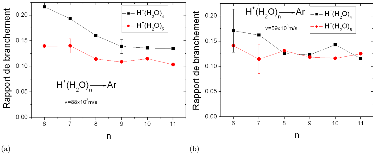
FIG. 3.22 – Rapport de branchement de production de H^+(H_2O)_4 et H^+(H_2O)_5 issus de H^+(H_2O)_n . (a) : n=6-11 v = 88 \times 10^3 \text{ m/s} (b) : n=6-11 v = 59 \times 10^3 \text{ m/s}
