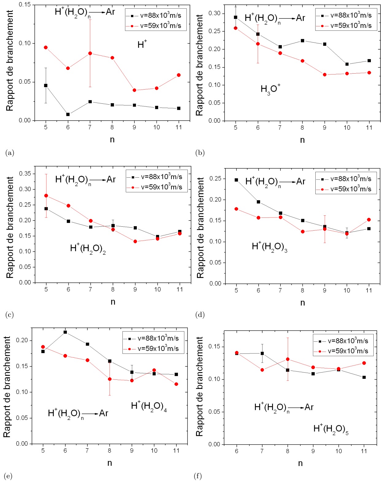
FIG. 3.21 – Rapport de branchement de production des différents ions issus de H^+(H_2O)_n n=5-11 . (a) : H^+ (b) : H_3O^+ (c) : H^+(H_2O)_2 (d) : H^+(H_2O)_3 (e) : H^+(H_2O)_4 (f) : H^+(H_2O)_5
