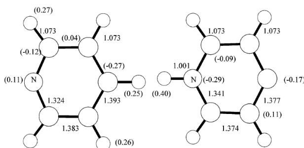
FIG. 3.35 – Structures optimisées de l'isomère conventionnel (à gauche) et distonique (à droite) de la pyridine ionisée. Les distances sont en angströms et les charges atomiques entre parenthèses (Y. Ibrahim et al. [114]).
