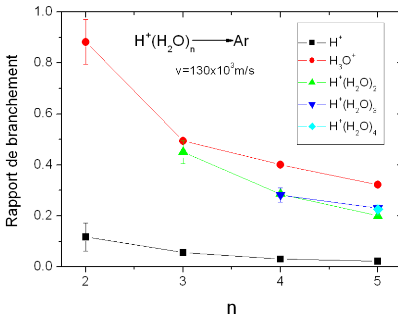
FIG. 3.18 – Rapport de branchement de production des différents fragments chargés issus de H^+(H_2O)_n n=1-5 . v = 130 \times 10^3 \text{ m/s}
