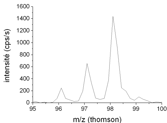
FIG. 3.28 – Spectre de masse : pyridine déshydrogénée (96), pyridine ionisée (97), pyridine protonée (98), chacune associée à une molécule d'eau
