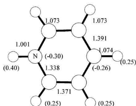
FIG. 3.37 – Structure optimisée de la pyridine protonée. Les distances sont en angströms et les charges atomiques entre parenthèses (Y. Ibrahim et al.[114]).
