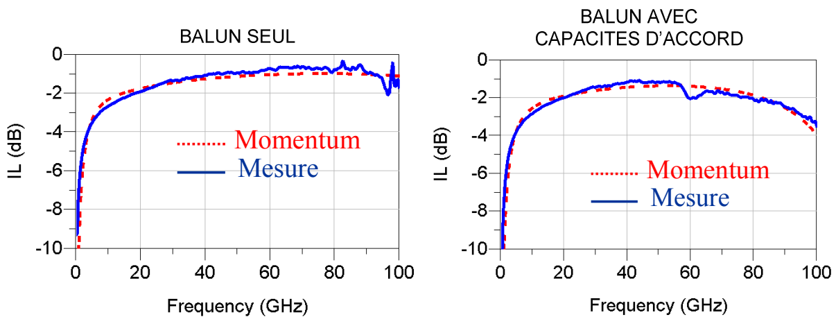
Figure III-56 : Mesure des pertes d'insertion ( IL ) du balun avec et sans capacité d'accord.
