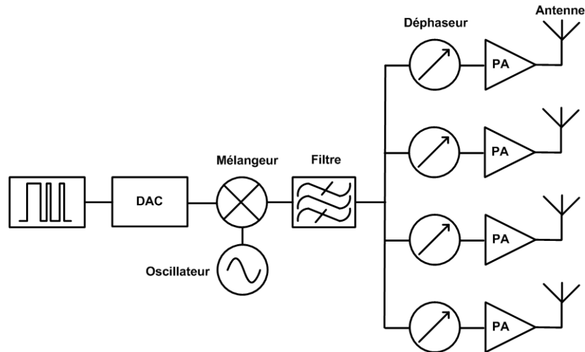
Figure I-16: Architecture d'émission à formation de faisceau - déphasage analogique RF.
