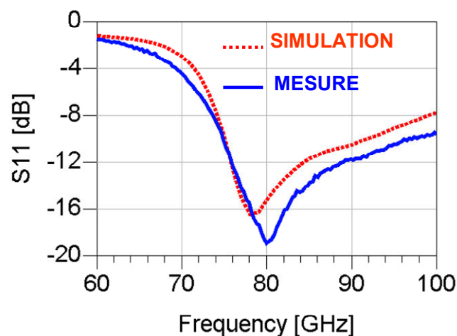
Figure IV-13 : Résultats de mesure de la co-intégration PA diff 50Ω/Antenne 50Ω.
