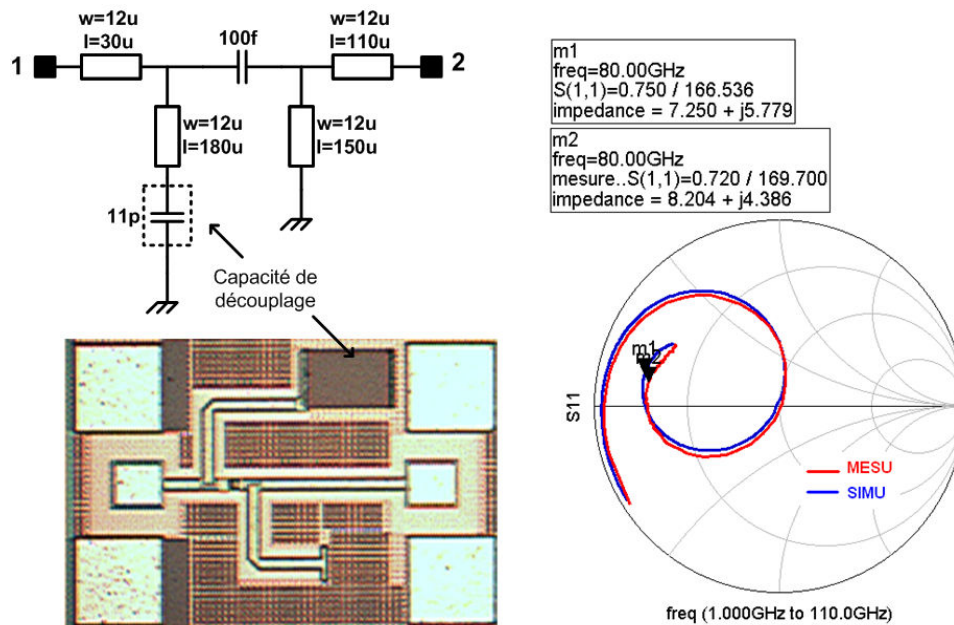
Figure III-37 : Structure et modélisation du réseau d'adaptation en sortie.
