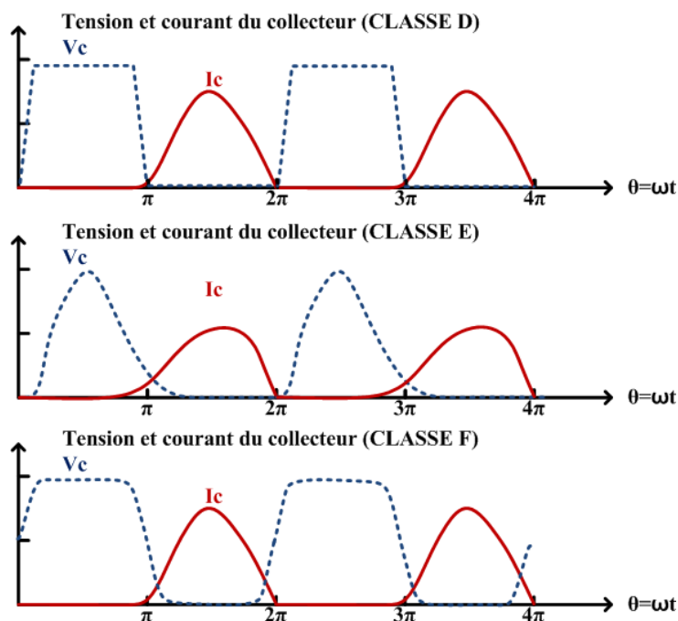
Figure II-12: Forme d'onde des tensions et des courants des PAs en classe non-sinusoidale.
