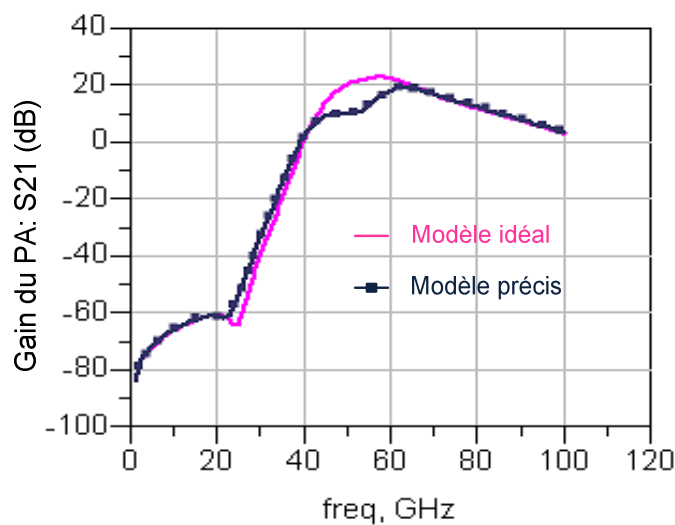
Figure III-35 : Comparaison du paramètre S_{21} simulé de l'amplificateur de puissance entre un modèle idéal et un modèle précis de la capacité de découplage.
