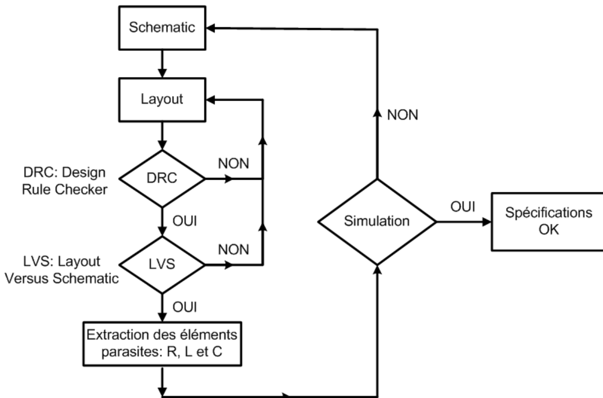
Figure III-1 : Procédé de conception du circuit.
