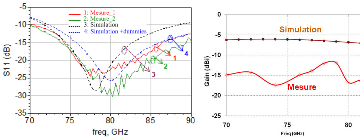
Figure IV-3 : Résultats de mesure de l'antenne dipôle sur silicium.
