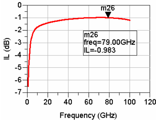
Figure III-52 : Simulation Momentum de la perte d'insertion IL du transformateur.
