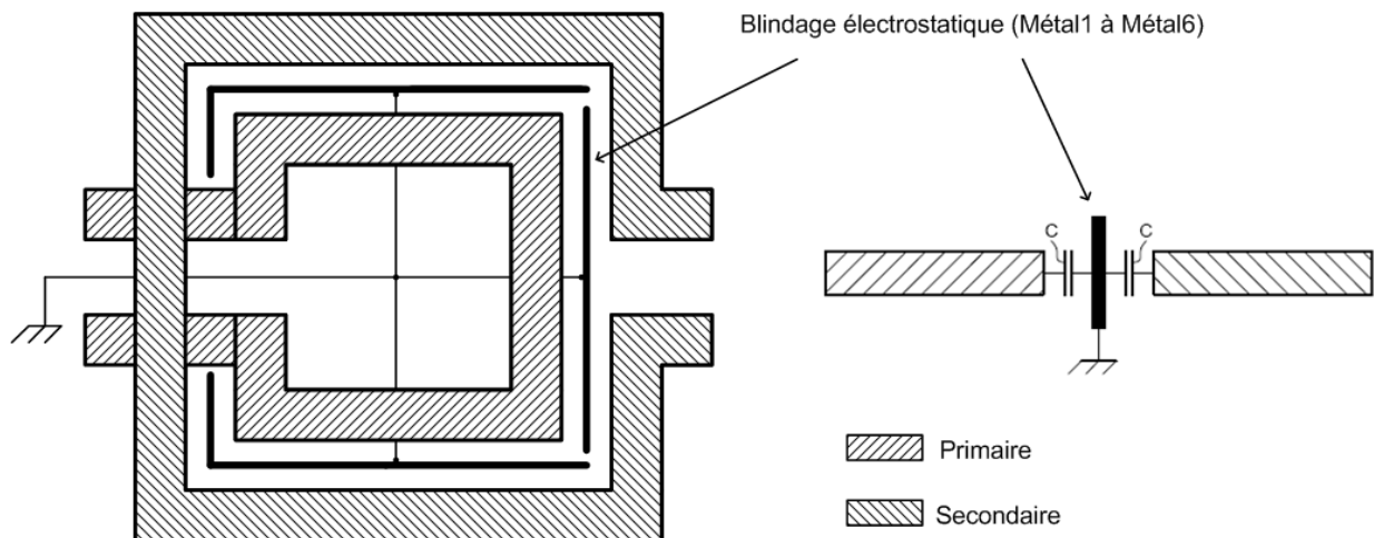
Figure III-51 : Représentation du balun avec le blindage électrostatique.
