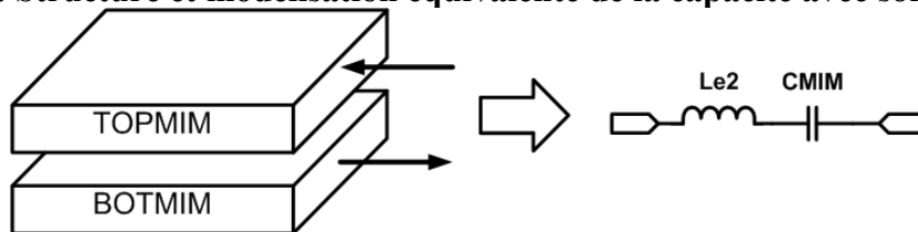
Figure III-32 : Structure et modélisation équivalente de la capacité avec sorties parallèles
