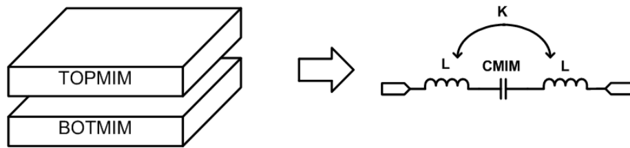
Figure III-30 : Structure et modélisation schématique de la capacité MIM.
