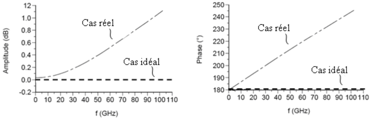
Figure III-48: Impact des capacités de couplage.
