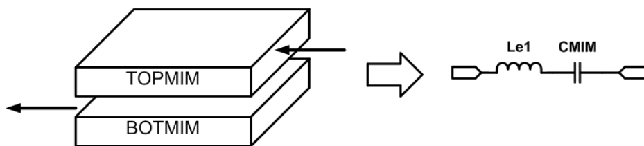
Figure III-31 : Structure et modélisation équivalente de la capacité avec sortie en opposées
