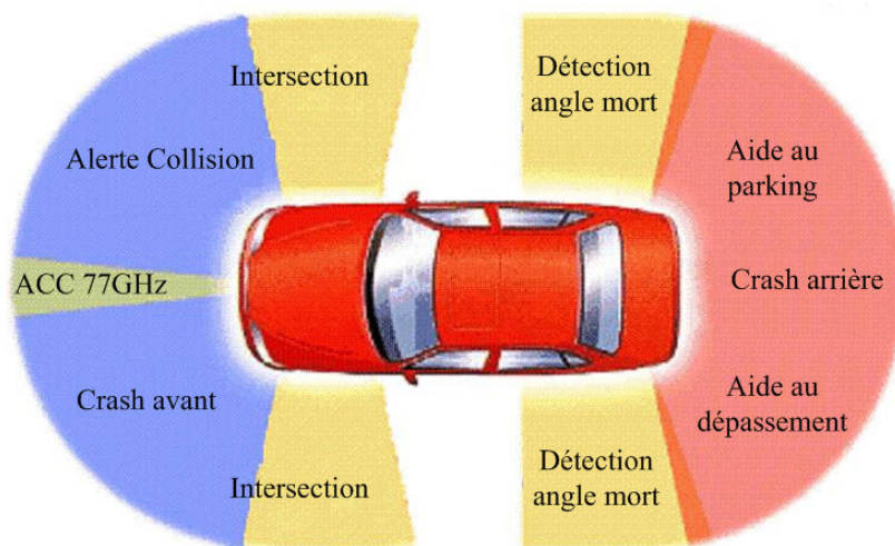
Figure I-4: Différentes applications de sécurité autour d'un véhicule par l'installation de plusieurs radars.
