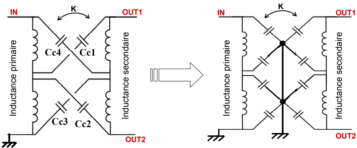
Figure III-49 : Suppression des capacités de couplage d'un transformateur intégré.
