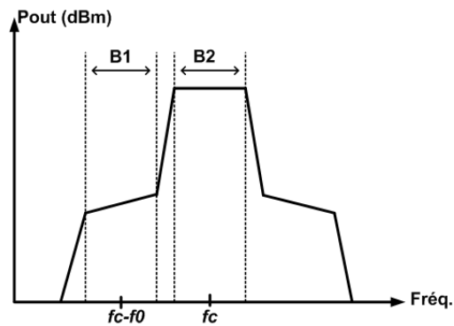
Figure II-6: Méthode de calcul de l'ACPR.
