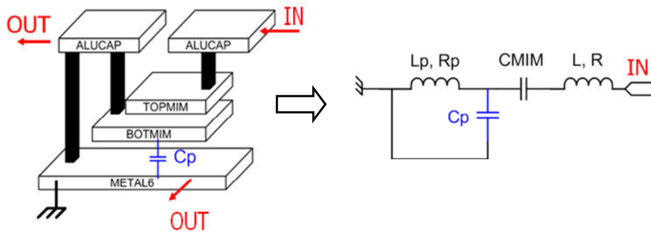
Figure III-34 : Structure physique et schématique de la capacité de découplage avec ses connexions.
