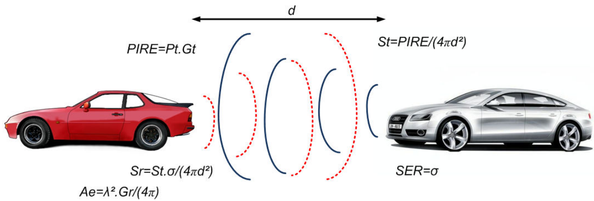
Figure IV-1 : Fonctionnement du système radar.
