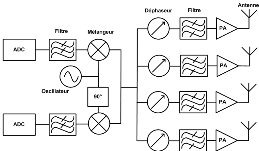
Figure I-17: Architecture de réception à formation de faisceau - déphasage analogique RF.
