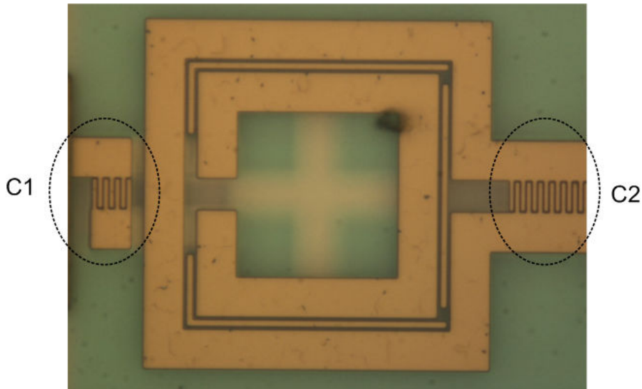
Figure III-55 : Photographie du balun avec capacité d'accord.
