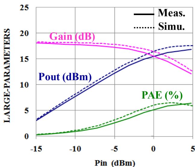
Figure III-61 : Mesure et simulation du gain, de la puissance de sortie et du rendement du PA différentiel avec balun intégré en fonction de la puissance d'entrée à 79GHz.
