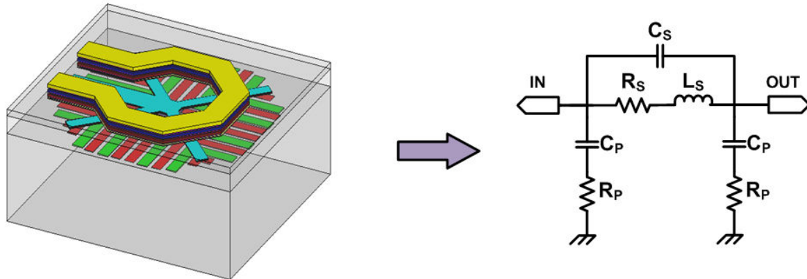
Figure II-29 : Structure d'une inductance et modélisation schématique.
