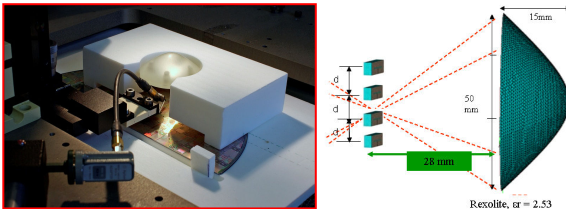
Figure IV-22: Antenne sur puce (silicium) associé avec une lentille en Rexolite [PIN10].
