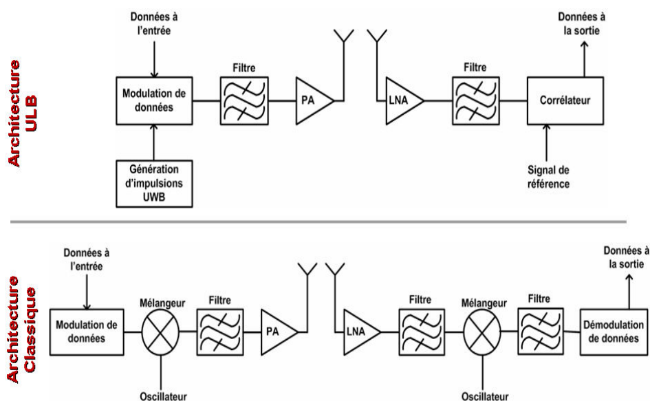
Figure I-7: L'architecture Emetteur/Récepteur d'un système de communication ULB et bande étroite.
