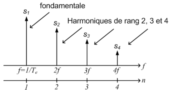
Figure A-6: Spectre d'un signal impulsionnel.
