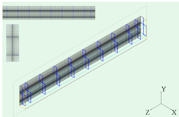
Figure III.13 : Maillage de la géométrie du refroidisseur
