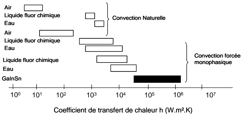
Figure I.16 : Comparaison du coefficient de transfert de chaleur h pour l'eau, les fluors chimiques et un liquide m\u00e9tallique (GaInSn)(Mudawar 2001) .
