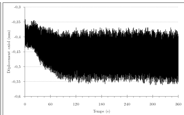
FIGURE 10.17 – Évolution du déplacement axial : la compression induite par la torsion est de moindre intensité (essai 19).
