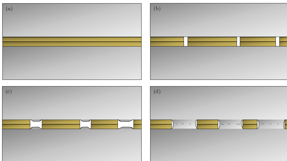
FIGURE 1.17 – Schéma de principe du mécanisme de jonction en soudage par pression
