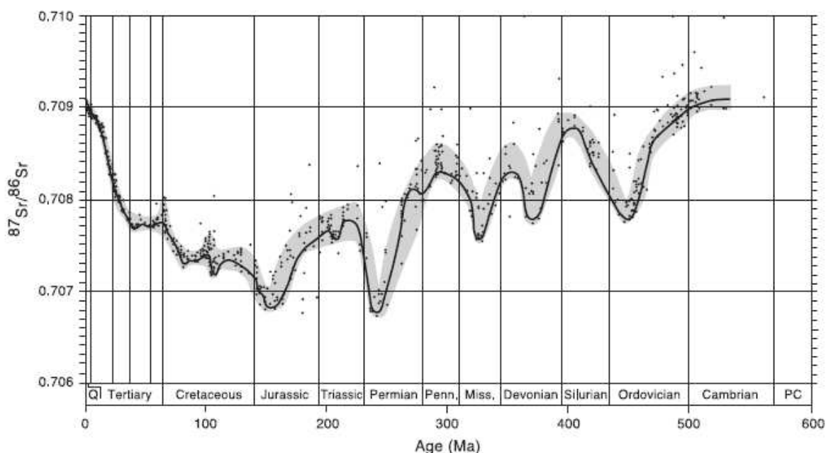
Figure 1. 6 : Courbe de variation du rapport ^{87}\text{Sr}/^{86}\text{Sr} dans l'eau de mer pendant le Phanérozoïque, basée sur l'analyse des carbonates marins, des roches évaporitiques et des fossiles (Burke et al., 1982).
