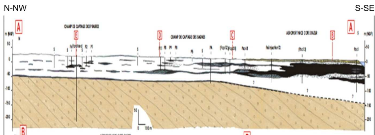
Figure 2. 5: Profil interprétatif de la nappe alluviale à l'aval de la basse vallée du Var (tiré de H2EA et Mangan, 2010).
