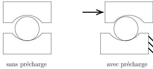
FIG. III.7: Effet d'une charge axiale appliquée sur une bague de roulement
