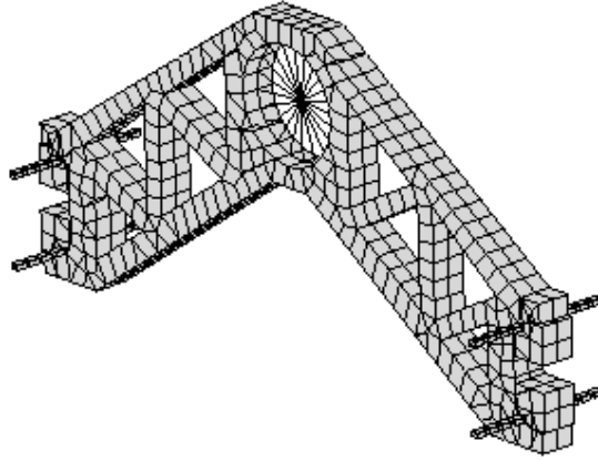
FIG. V.1: Maillage 3D du support-palier type treillis
