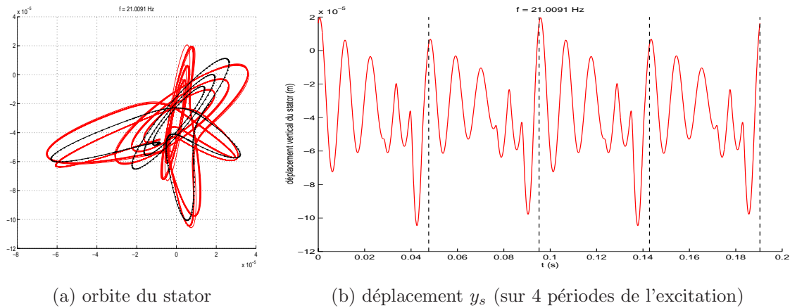
FIG. III.25: Solution 2T -périodique à 21 Hz
