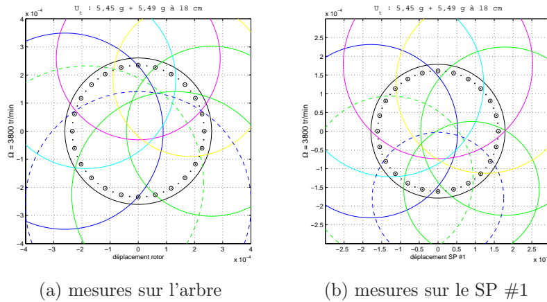
FIG. V.22: Equilibrage au niveau du disque fan par la méthode des 3 masselottes
