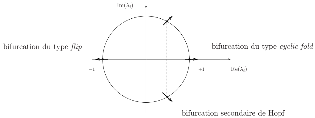
FIG. II.8: Les principaux types de bifurcation
