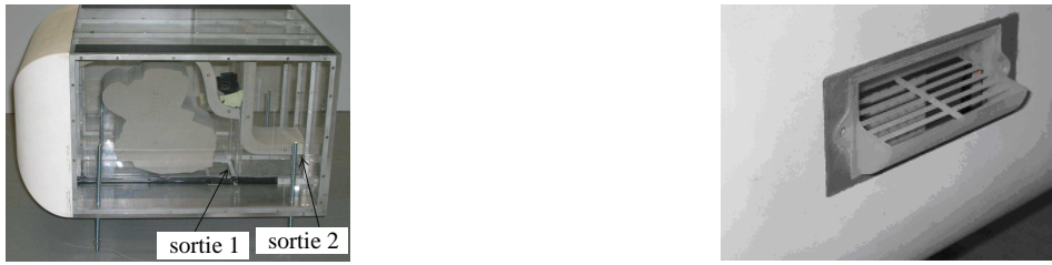
Figure II-43 : Maquette simplifiée du compartiment moteur (à gauche) et sa section d'entrée (à droite) [IVA-05]
