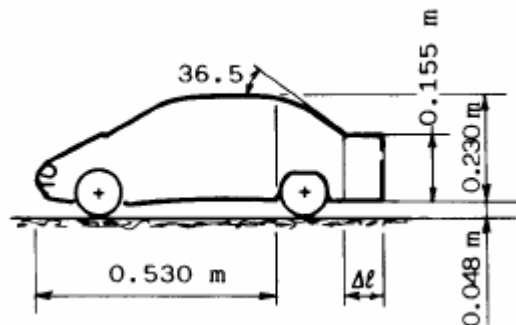
Figure III-40 : Maquette à l'échelle 1/5^{\text{ème}} d'un véhicule de type tricorps utilisé pour valider expérimentalement la relation d'Onorato [ONO-84].
