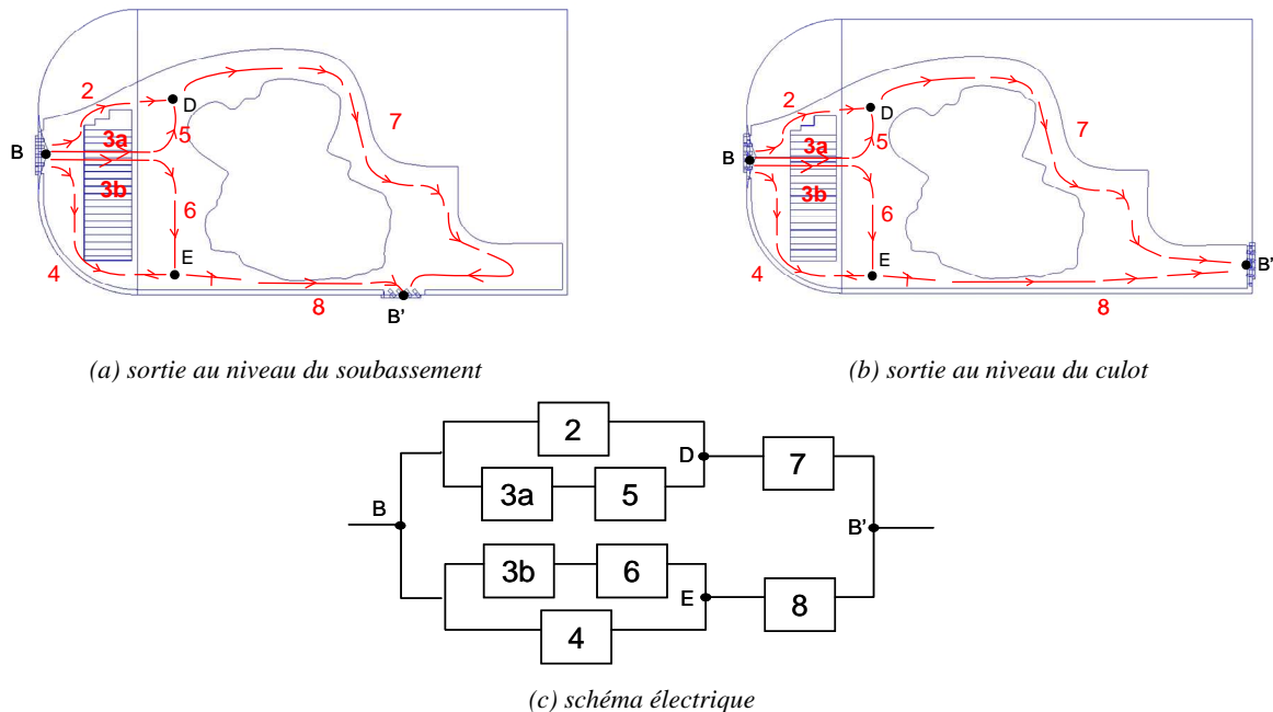
Figure V-15 : Ecoulements élémentaires internes au compartiment moteur pour les sorties 2 (a), 3 (b) et 4 (c), et schéma électrique correspondant (d).
