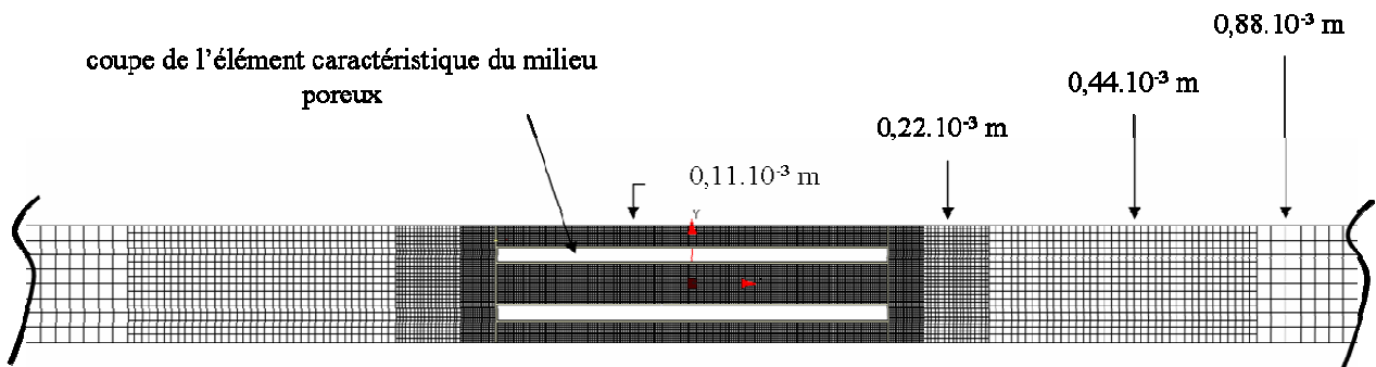
Figure IV-11 : Coupe du domaine de calcul en y = 0 décrivant les régions du maillage et les tailles de mailles associées.
