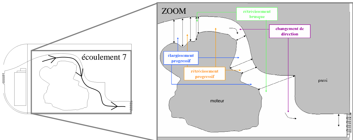
Figure V-23 : Décomposition, en pertes de charge élémentaires, de l'écoulement 7 au-dessus du moteur.
