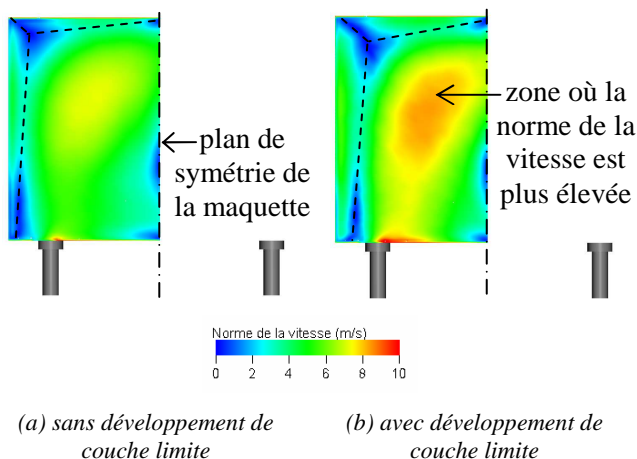
Figure IV-20 : Répartition de la norme de la vitesse au culot de la maquette simplifiée.
