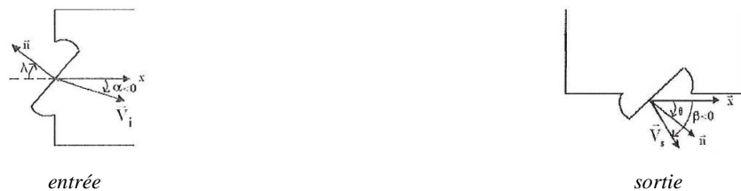
Figure II-42 : Configurations géométriques dans les sections d'entrée et de sortie du compartiment moteur lorsque les angles a et b sont introduits pour caractériser la direction des vecteurs vitesse [IVA-05].
