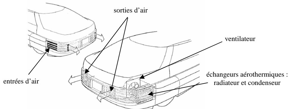
Figure II-19 : Système de refroidissement du concept car Probe IV [SAN-83].
