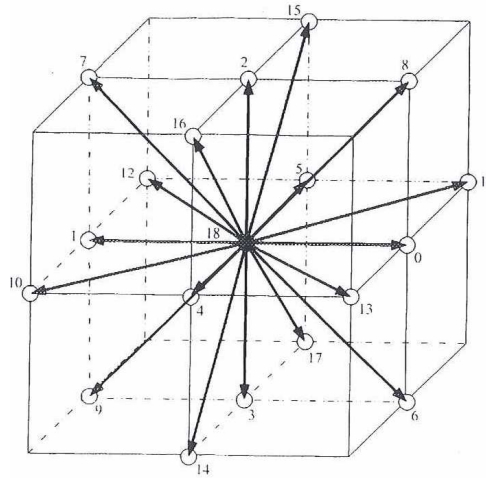
Figure F-2 : Modèle D3Q19.
