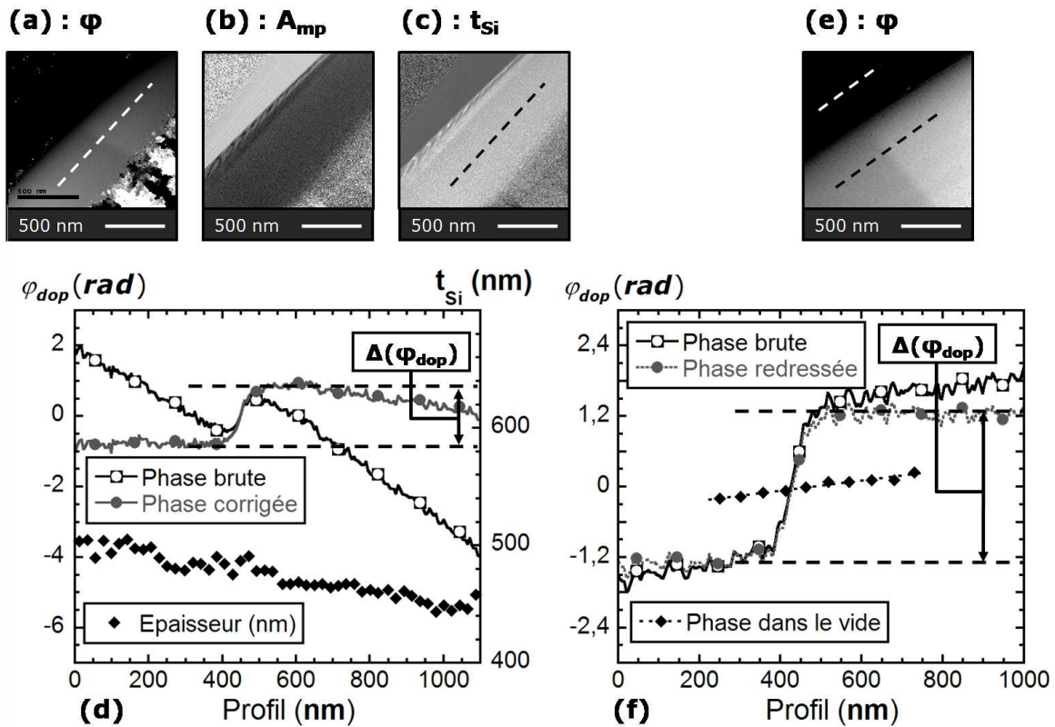
FIGURE III.13 – Image de phase (a), d’amplitude (b), et épaisseur extraite de l’amplitude (c) d’une jonction p-n symétrique (échantillon 2 : 2 \cdot 10^{18} at \text{cm}^{-3} ) préparée par FIB à 30 keV. L’image de phase correspond à la figure (III.12)(c), avec un grandissement et une orientation différents après avoir subi un redressement de phase. Les faces de cet échantillon ne sont pas parallèles, une pente d’épaisseur significative se manifeste. L’image de phase (e) est extraite d’un autre échantillon (qui n’est pas représenté dans la figure (III.12)). Son épaisseur est constante, mais un champ électrostatique dans le vide introduit une pente de phase sur l’ensemble de l’image. Les profils représentés dans (d) sont extraits de (a,b,c). Les profils de (f) sont extraits de (e). La cartographie d’épaisseur (c) est extraite de l’image d’amplitude (b) avec \lambda_{ipm} = 130 nm. En utilisant V_0 = 11,5 V, nous pouvons corriger le profil de phase par une correction \Delta\varphi_{correc} dépendante des écarts \Delta t_{Si} d’épaisseur. La courbe redressée présente une asymétrie inattendue, imputée à des effets de charge dans le silicium, ou à une variation d’épaisseur non linéaire
