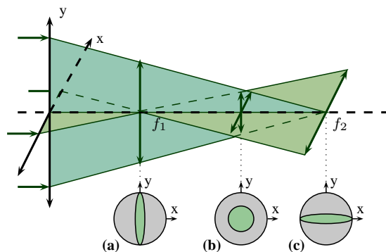
FIGURE II.12 – Forme d'un faisceau astigmatique suivant l'axe optique. Un faisceau parallèle est focalisé au foyer d'une lentille. Les deux axes x et y de la lentille ont des focales différentes ( f_1 pour x , f_2 pour y ). Les images formées au premier foyer (a), au point de moindre aberration astigmatique (b) et au second foyer (c) sont schématisées.
