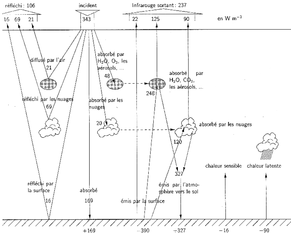
FIG. 6.11 – Bilan radiatif annuel moyen du système Terre-atmosphère. Source : Jacques Lefrere - cours de rayonnement de l'université Paris VI.
