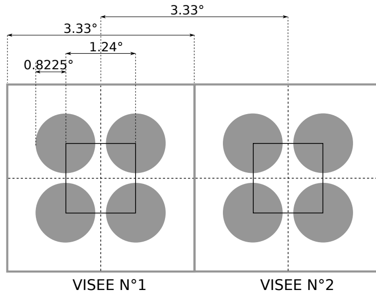
FIG. 6.10 – Géométrie de la visée IASI. Les disques gris représentent les champs de vue des quatre capteurs.
