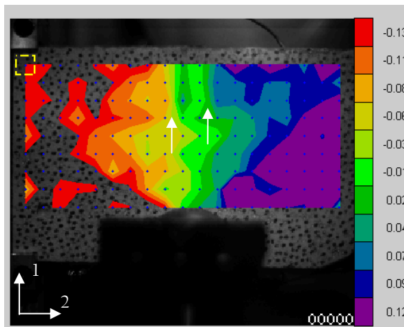
(a) Champ de déplacement U2 en pixel, essai MB50 humide n°23, image n°40, t = 60 \mu s – vecteurs déplacement associés (Amplitude : x100)
