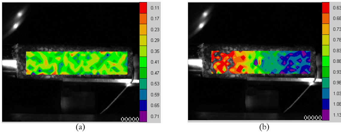
Figure 4-40 : (a) Champ de déplacement axial (en pixel, en déduisant le mouvement de corps solide) au moment où la contrainte s'annule ( t = 0 \mu\text{s} sur le graphe de la Figure 4-35a) et (b) champ de déplacement axial (en pixel, absolu) 35 \mu\text{s} plus tard – 1 \text{ pixel} = 0,561 \text{ mm} , taille d'éléments : 8 pixels
