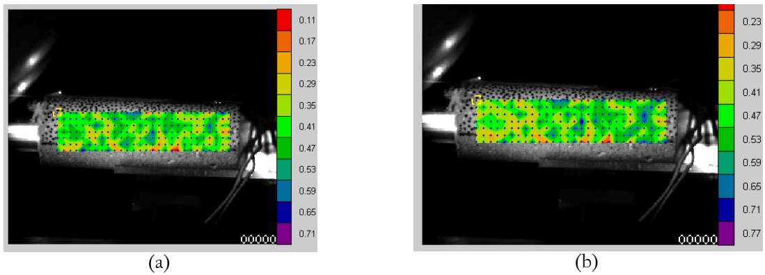
Figure 4-38 : Champ de déplacement axial (en pixel) (a) à t = 56 \mu\text{s} et (b) à t = 60 \mu\text{s} – Essai 49s sur MB50 sec
