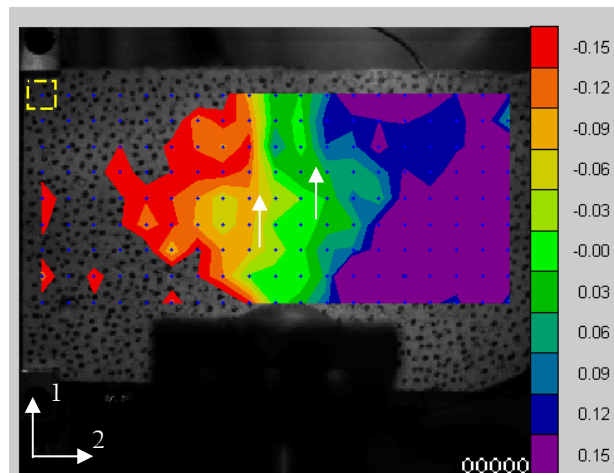
(a) Champ de déplacement U2 en pixel, essai MB50 humide n°23, image n°40, t = 60 \mu s – vecteurs déplacement associés (Amplitude : x100)
