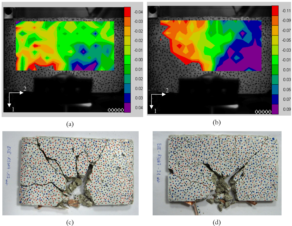
Figure 5-23: Champ de déplacement U2 en pixel (1 pixel \approx 0,65 mm) – essai n°17, (a) t = 15 \mu\text{s} et (b) t = 60 \mu\text{s} ; Epreuve post mortem pour (a) l'essai n° 17 et (b) n°21
