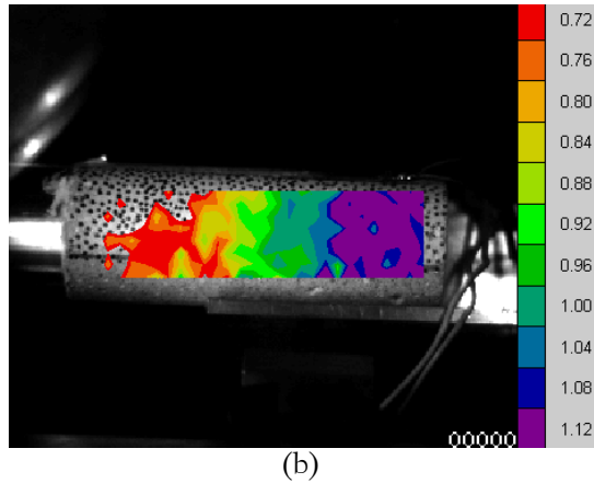
Figure 4-39 : (a) Champ de déplacement axial (en pixel) à t = 72 \mu\text{s} (en déduisant le mouvement de corps solide) et vecteurs déplacement correspondant (Amplitude \times 50 ) et (b) champ de déplacement axial à t = 92 \mu\text{s}
