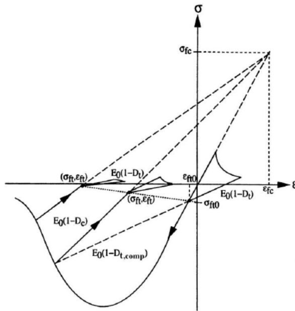
Figure 2-31 : Principe du modèle PRM illustré en ID [Pontiroli, 1995]
