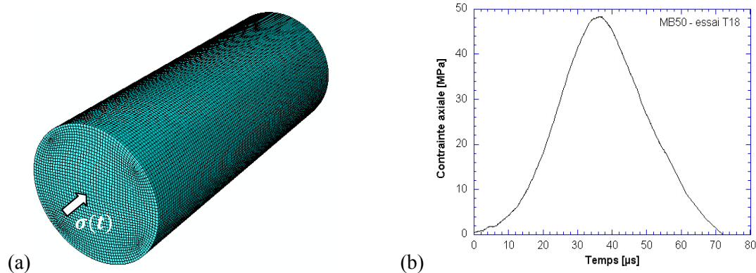
Figure 4-12: (a) maillage utilisé pour les simulations d'écaillage et (b) pulse de chargement incident pour ces calculs
