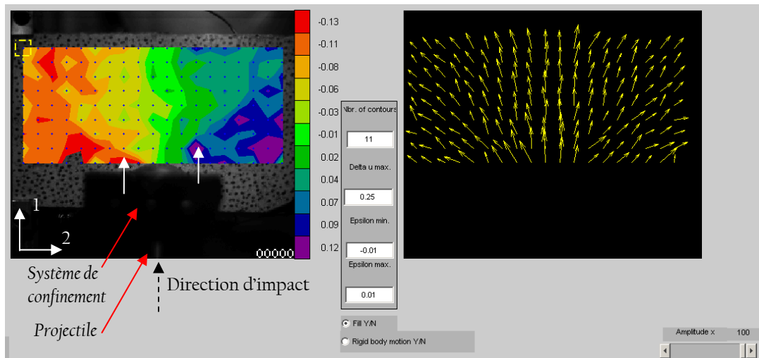
(a) Champ de déplacement U2 en pixel, essai MB50 humide n°23, image n°40, t = 60 \mu s – vecteurs déplacement associés (Amplitude : x100)
