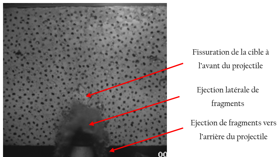
Figure 5-36 : Pénétration du projectile dans le carreau de béton R30A7 sec, Essai n°15, image n°58, t = 600 \mu s après impact
