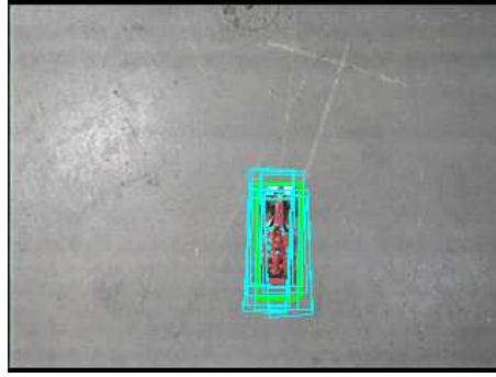
FIGURE 3.13 – Exemple d'initialisation des particules autour de la position de l'objet. Par souci de clarté seules 30 particules ont été représentées.
