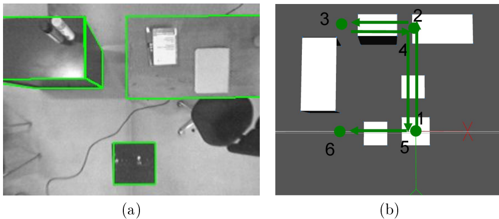
FIGURE 6.12 – Exemple de vue de la caméra embarquée avec la reprojektion du modèle obtenue (a) et trajectoire demandée (b).
