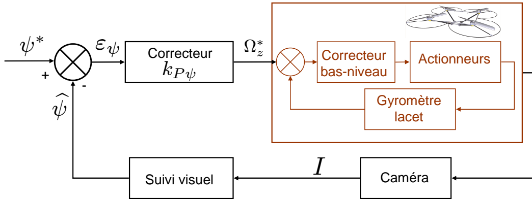
FIGURE 6.1 – Contrôle du lacet.
