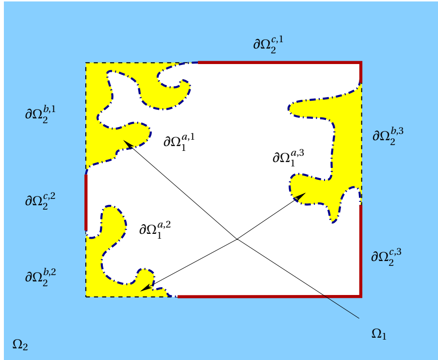
FIGURE 5.8: Problème acoustique sur la structure complexe - Rappel des notations
