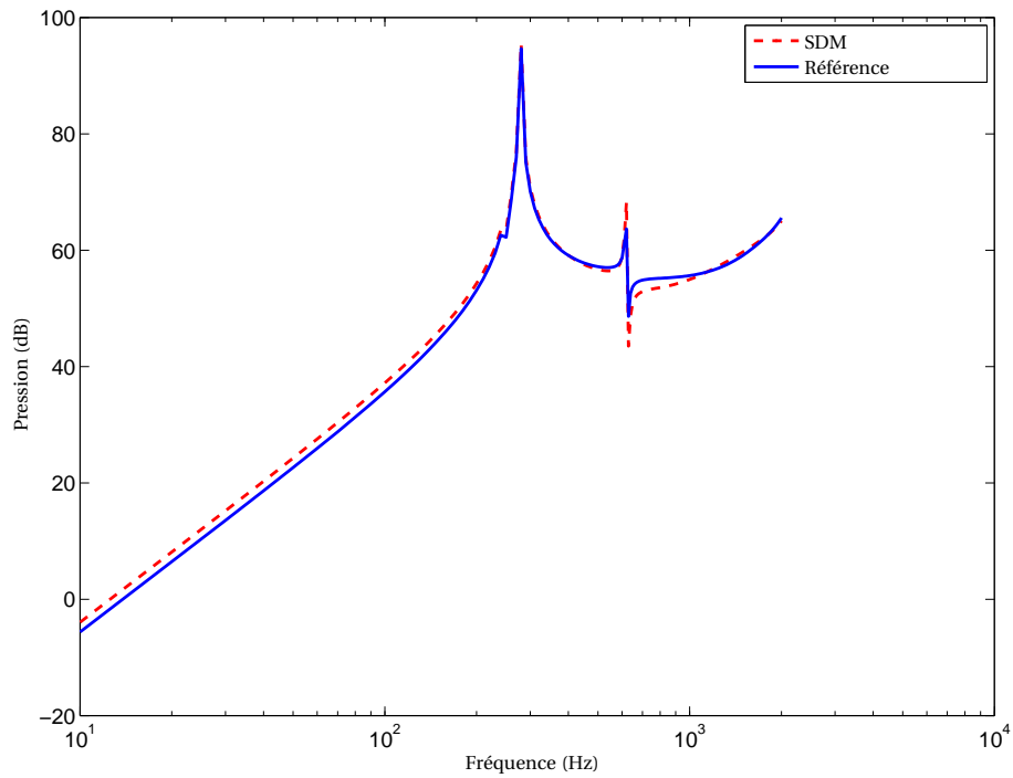
FIGURE 5.17: Pression au centre de la face arrière
