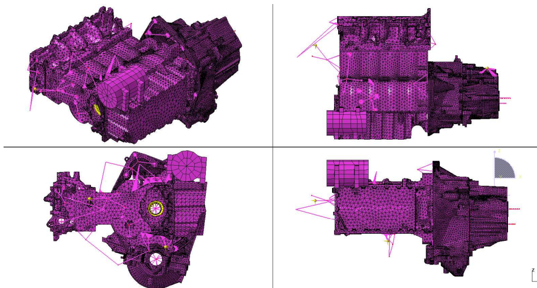
FIGURE 4.20: Visualisation du GMP avec le carter cylindres simplifié
