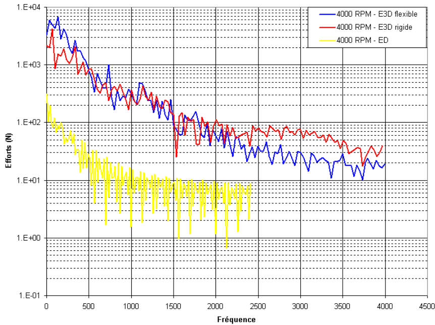
FIGURE 2.11: Efforts paliers moteur DW12 à 4000 tr/min
