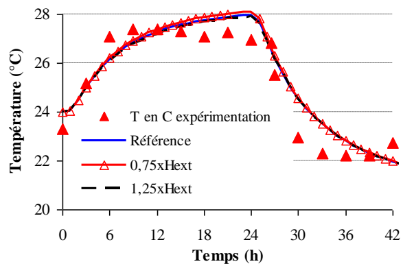
Figure 2. 28 : Influence des coefficients de convections thermiques et massiques extérieurs sur la température en C.
