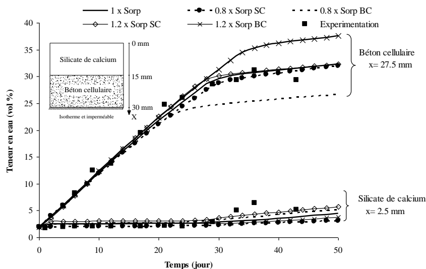
Figure A. 11 : Influence de la courbe de sorption sur les résultats.
