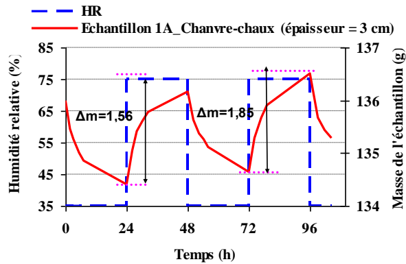
Figure A. 53: La variation de la masse de l'échantillon 1A Chanvre-chaux ( e=3 cm) pour le TEST@24,24h.
