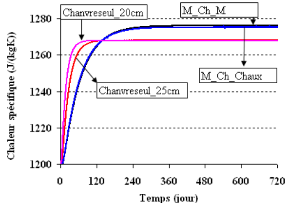
Figure 3. 20: Chaleur spécifique.
