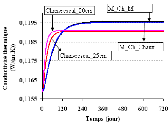
Figure 3. 19 : Conductivité thermique.
