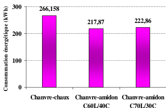
Figure 4.10 a : Consommation énergétique.
