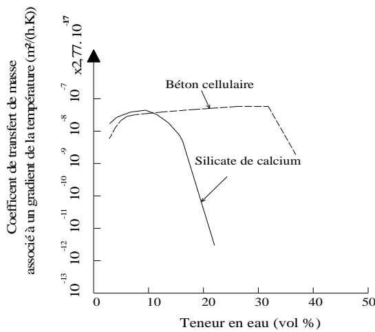
Figure A. 8: Coefficient de transfert de masse associé à un gradient de la température.
