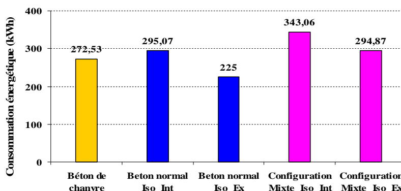
Figure 3.87: Consommation énergétique en fonction des configurations étudiées.
