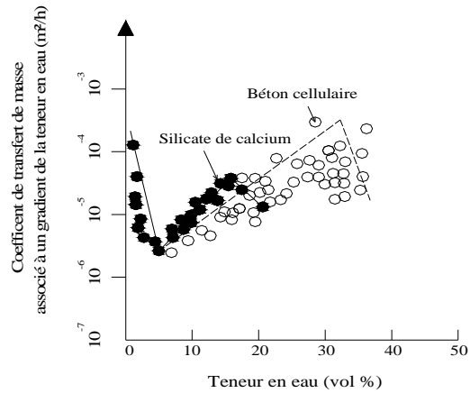
Figure A. 7: Coefficient de transfert de masse associé à un gradient de la teneur en eau.
