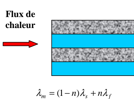
Figure 1.15a : Modèle en parallèle
