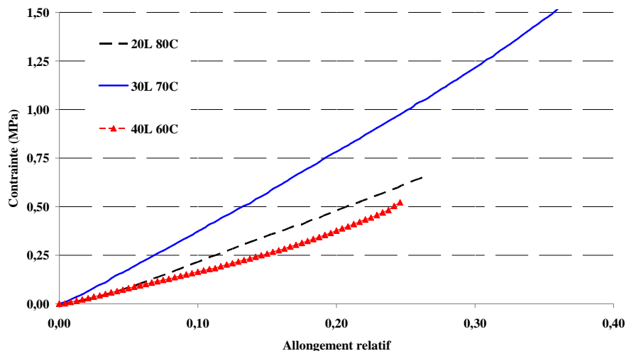
Figure 4. 2: Relation contrainte déformation des différentes formulations du béton de chanvre- amidon (Hotineanu, 2010).
