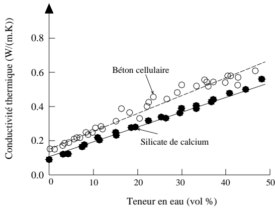
Figure A. 6: La conductivité thermique des matériaux utilisés.
