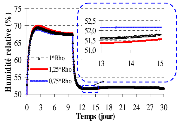
Figure 3. 30: Influence de la masse volumique sur l'humidité relative intérieure du local.
