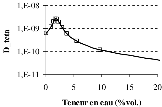
Figure 2. 7: Evolution de la diffusivité hydrique isotherme D_{\theta} en fonction de la teneur en eau volumique du béton de chanvre.
