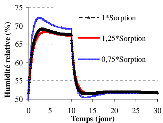
Figure 3. 34: Influence de l'isotherme de sorption sur l'humidité relative intérieure du local.
