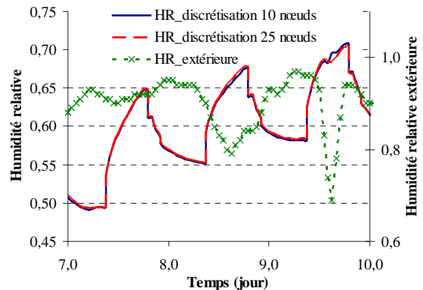
Figure 3. 51 : Influence de la finesse de discrétisation sur l'humidité relative du local.
