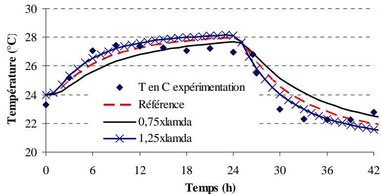
Figure 2. 21 : Influence de la conductivité thermique sur l'évolution de la température en C.
