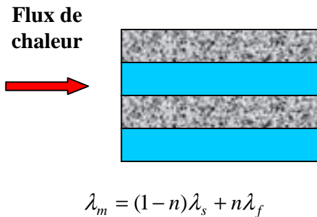
Figure 1.15a : Modèle en parallèle
