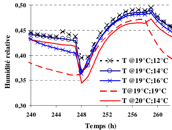
Figure 3. 59: Variation de l'humidité relative du local pour les différentes programmations de chauffage.
