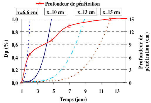
Figure A. 31: Variation de la valeur de D_p (1 %) et de la profondeur de pénétration hydrique.
