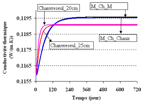
Figure 3. 19 : Conductivité thermique.
