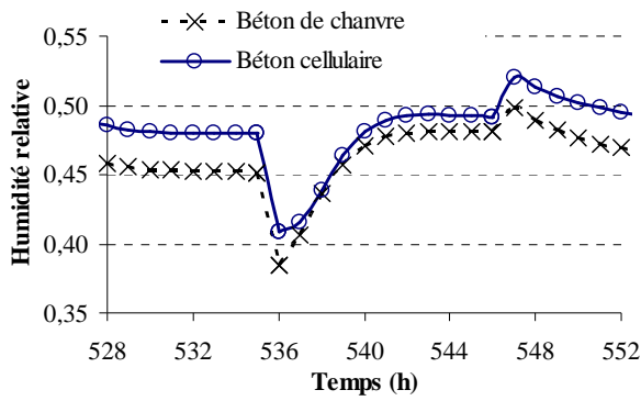
Figure 3. 84: Humidité relative du local de 22 ème jour pour un taux de surface vitrée totale.
