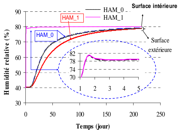
Figure A. 26: Variation de l'humidité relative aux surfaces extrêmes pour les modèles HAM_1 et HAM_0.
