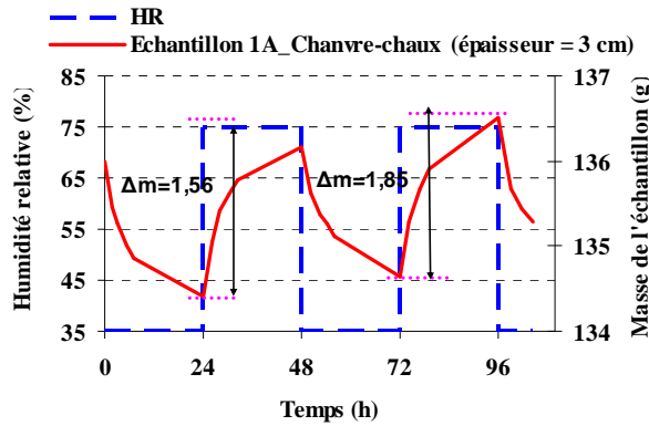
Figure A. 53: La variation de la masse de l'échantillon 1A_Chanvre-chaux ( e=3\text{ cm} ) pour le TEST@24,24h.
