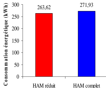
Figure 4.7b : Consommations énergétiques.
