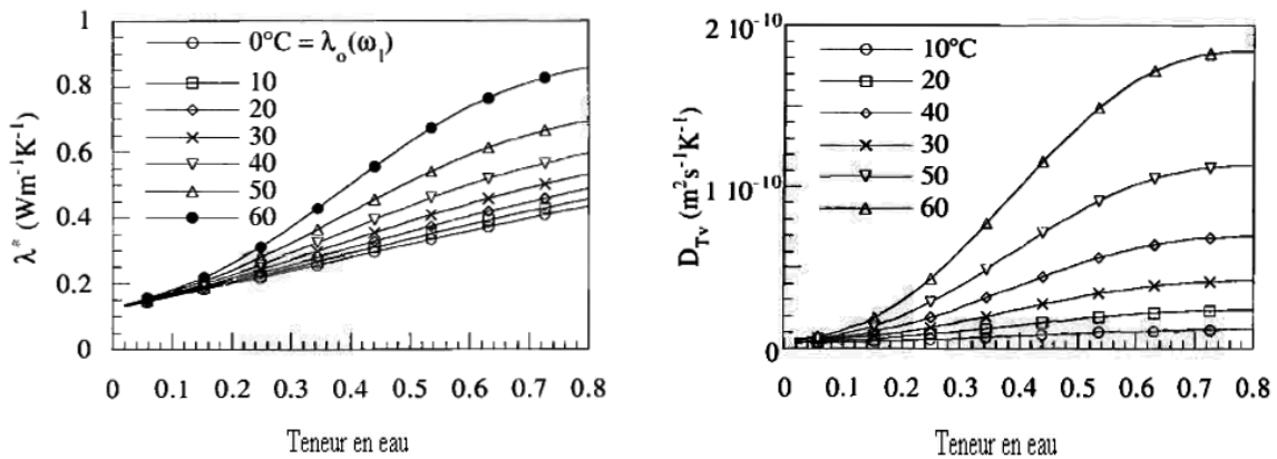
Figure 2. 5 : La conductivité thermique et les coefficients de diffusion de la vapeur en fonction de la teneur en eau volumique sous un gradient de température pour le cas du béton cellulaire (Crausse et al., 1996).
