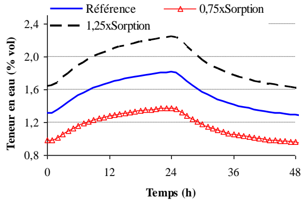
Figure 2. 26 : Influence de l'isotherme de sorption sur la teneur en eau en C.
