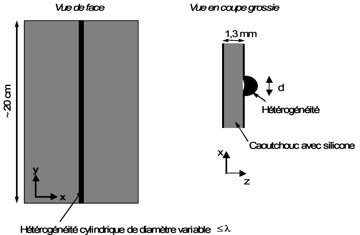
Figure 3. Le plan hétérogène vu de face et en coupe grossie.
