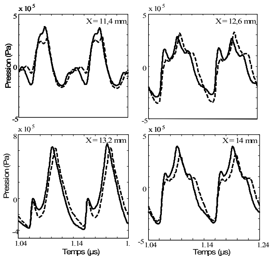
Figure 38. Formes temporelles de la pression mesurée (trait plein) et calculée (pointillé) en z = 7,4 mm du plan hétérogène de 30 demi-cylindres de diamètre 1,5 mm espacés de 3 mm, et à diverses positions transverses (indiquées sur les figures).
