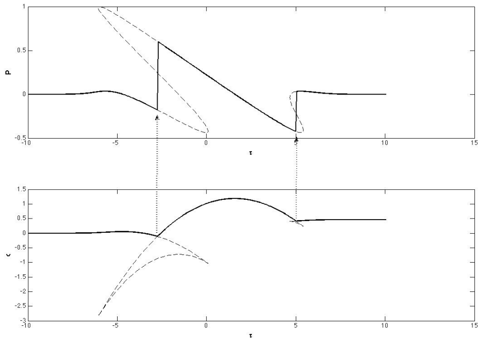
Figure 28. Principe de la méthode de Hayes : en haut la pression, en bas le potentiel. Lignes en tirets : solutions de Poisson multivaluées. Lignes continues : solutions mono-valuée (maximum pour le potentiel). La correspondance entre les chocs pour le potentiel (points anguleux) et la pression (discontinuités) est repérée par les flèches.
