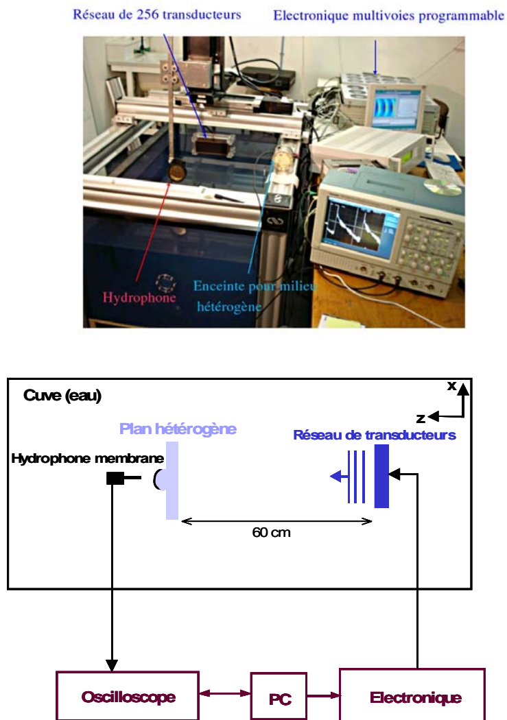
Figure 1. Dispositif expérimental
